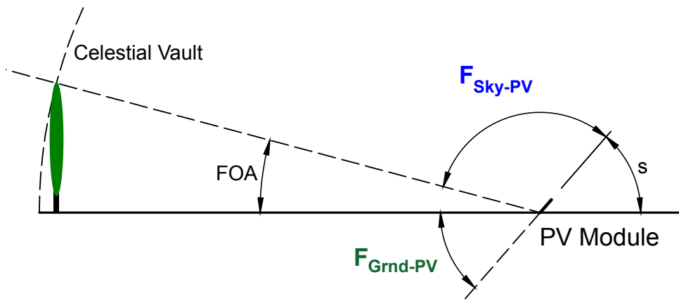
(d) View factors for frontal modules
