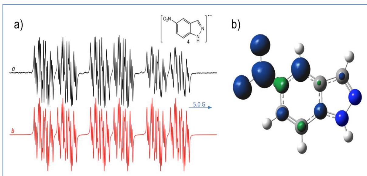
Figure 10 : a) spectre RSE (a) des espèces radicalaires électrogénérées du 4 (1 mM) dans 0,1 M Bu 4 NClO 4 -CH 3 CN. E_{app} = E^0_1 . En rouge (b) est reportée la simulation théorique correspondante. b) Densités de spin iso-surfaces pour l'anion radicalaire du 4 .
