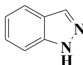
1H-indazole ( 1 )*
