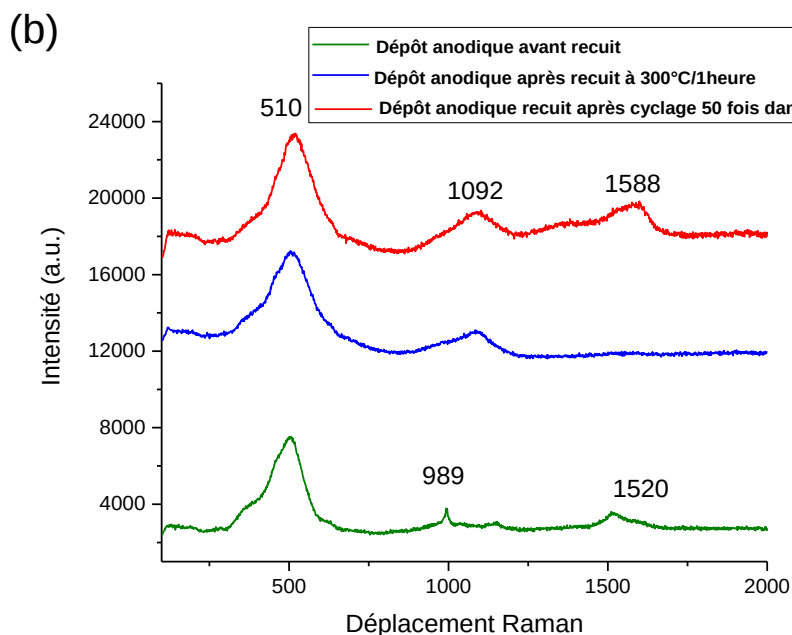
Figure 27 : Analyse (a) DRX et (b) spectroscopie Raman des couches de NiOxHy déposées par oxydation en milieu aqueux
