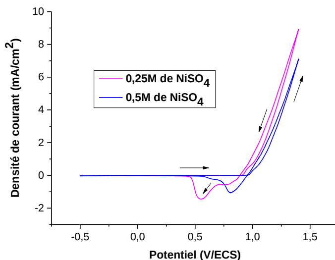
Figure 22 : Voltampérométrie cyclique du bain anodique avec 0,25M et 0,5M de NiSO 4 dans la gamme de potentiel [-0,5 ; 1,4V/ECS] ( v_b=10 \text{ mV.s}^{-1} )
