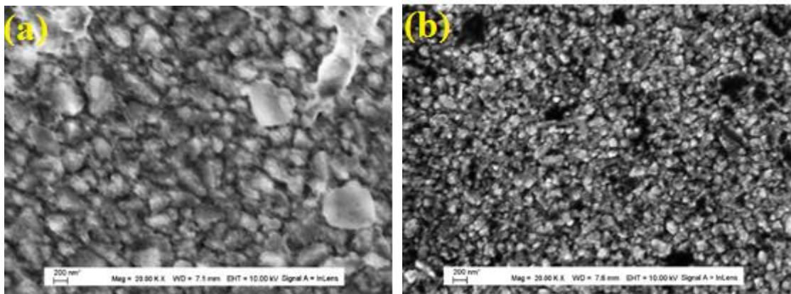
Figure 20 : Images MEB de la couche de CuFeO 2 (a) avant et (b) après recuit
