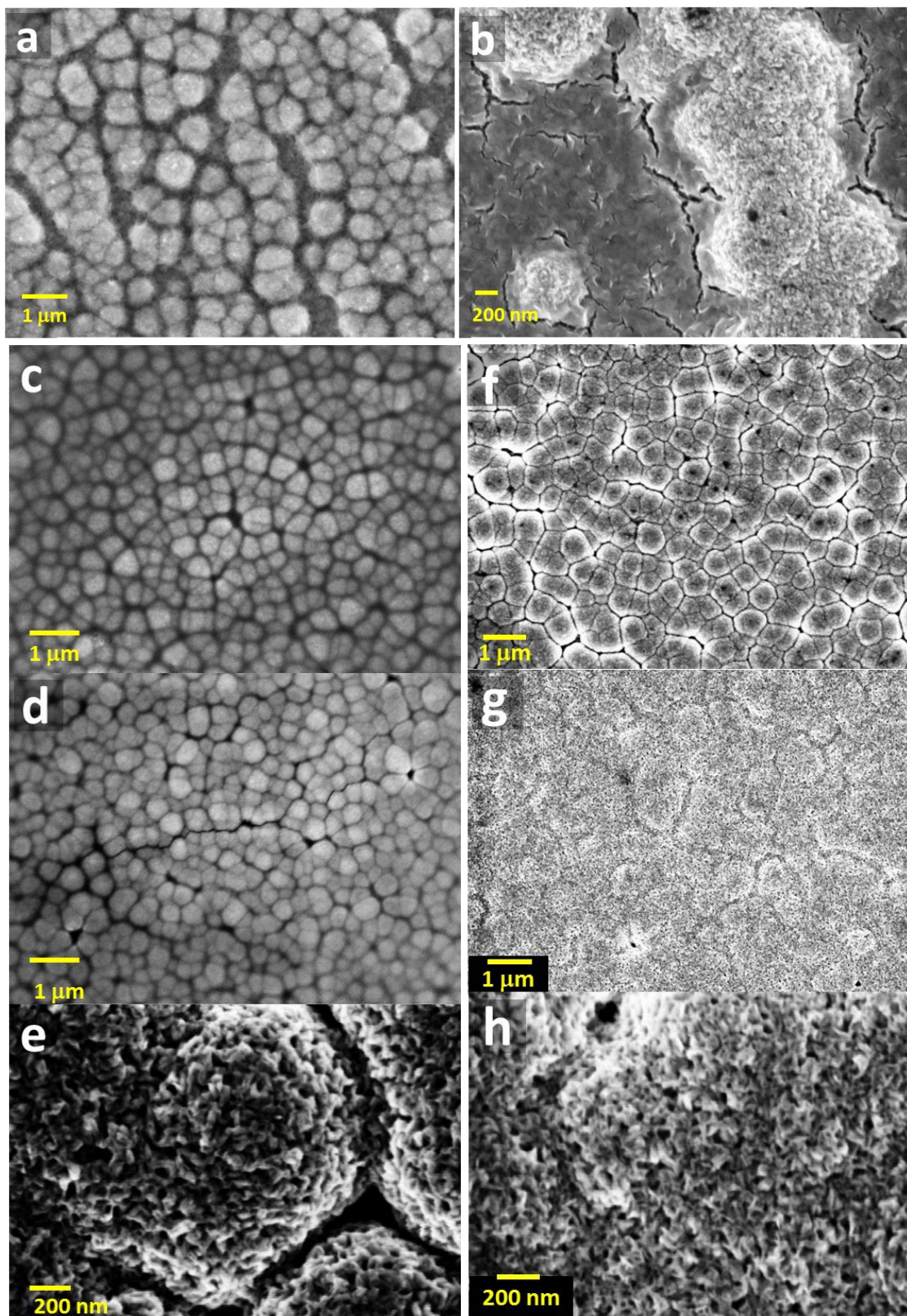
Figure 14 : Clichés MEB des couches déposées à (a,b) -0,80V/ECS, (c,d,e) -0,85V/ECS, (f,g,h) -0,90V/ECS. (a,c,f) Couches séchées à 200°C/10 minutes, (b,d,e,g,h) Couches recuites à 450°C/16h
