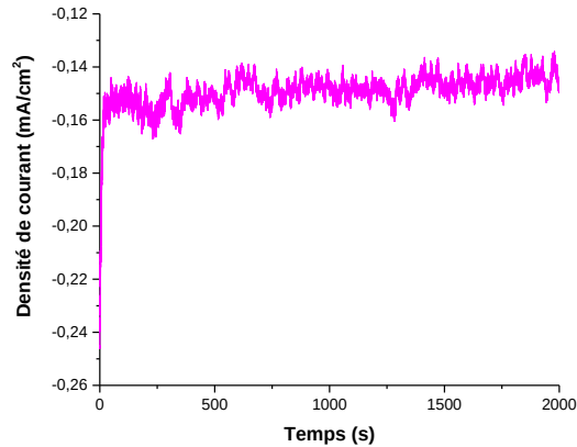
Figure 19 : Courbe de dépôt de CuFeO 2
