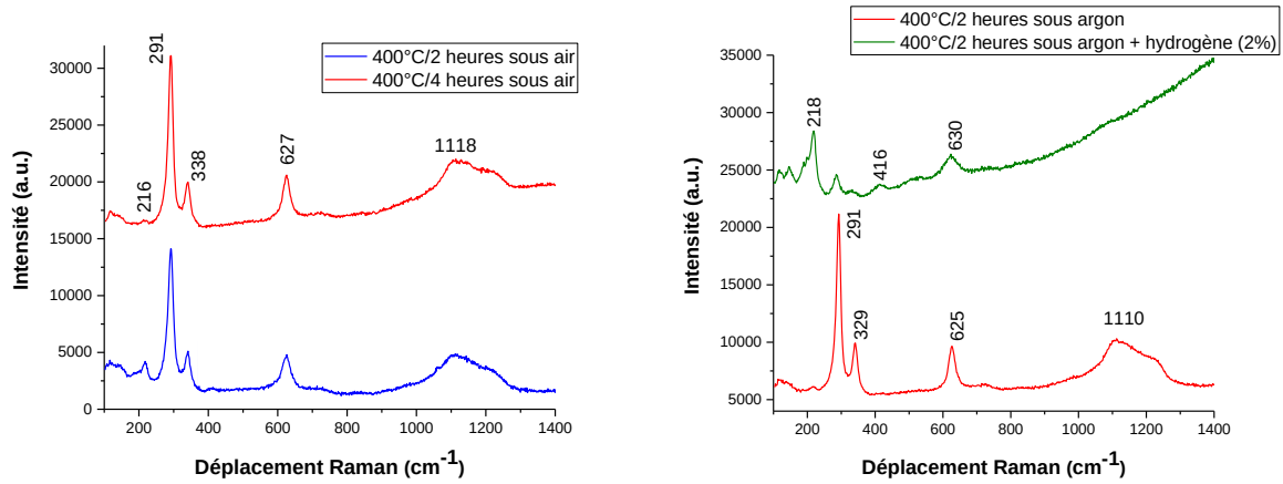
Figure 9 : Spectres Raman des couches de \text{Cu}_2\text{O} recuites à 400^\circ\text{C} (a) sous air pendant 2 heures et 4 heures (b) sous argon et sous argon + hydrogène (7%) pendant 2 heures
