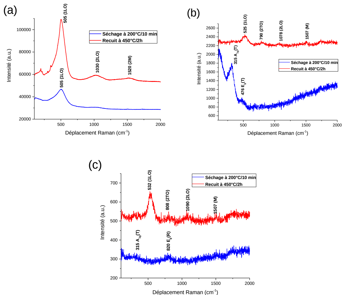
Figure 3 : Spectres Raman des couches déposées à -0,85 V/ECS après séchage à 200°C/10 min et après recuit à 450°C/2h sous air pour (a) DMSO seul (b) DMSO_eau (2%) (c) DMSO_eau (25%)
