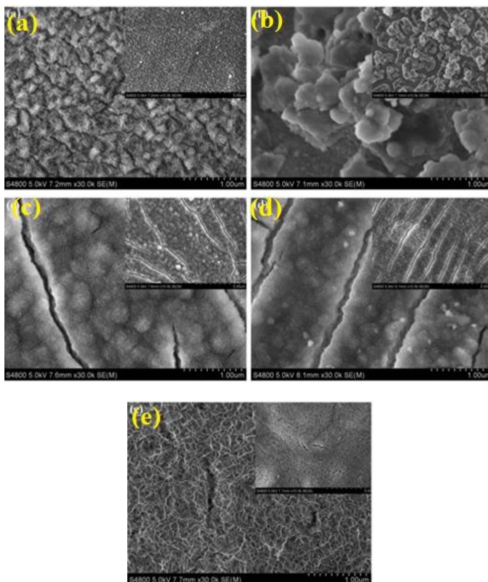
Figure 15 : Images MEB des couches Ni(OH) 2 déposées à -0.7V/ECS à différentes températures (a) 20°C, (b) 30°C, (c) 40°C, (d) 50°C et (e ) 65°C [62]
