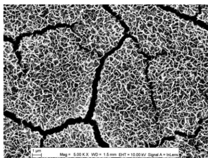
Figure 12 : Vue générale d'une couche recuite à 450°C pendant 30 minutes
