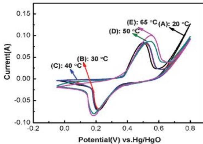
Figure 16 : Voltampérométrie cyclique des films de \text{Ni(OH)}_2 déposés à -0.7V/ECS obtenus à différentes températures
