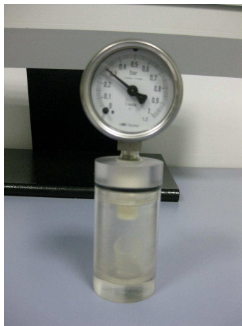
Figure 2.26 – Photo d'un manocalcimètre : Le conteneur est fermé avec un manomètre qui mesure l'augmentation de la pression due à la production de CO_2 résultant de la dissolution de CaCO_3 dans le réacteur.
