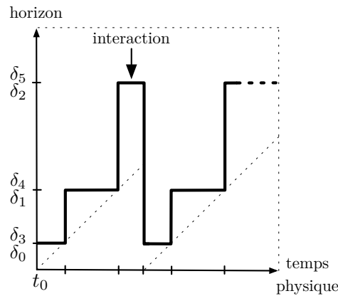
FIGURE 3.4 – Progression des horizons d'ordonnancement en présence d'une interaction.
