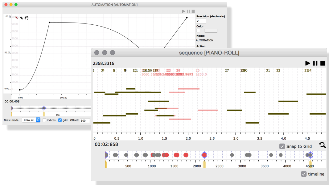
FIGURE 4.6 – Objets musicaux dédiés au MIDI implémentés à partir de la structure s-object : automation et piano-roll.
