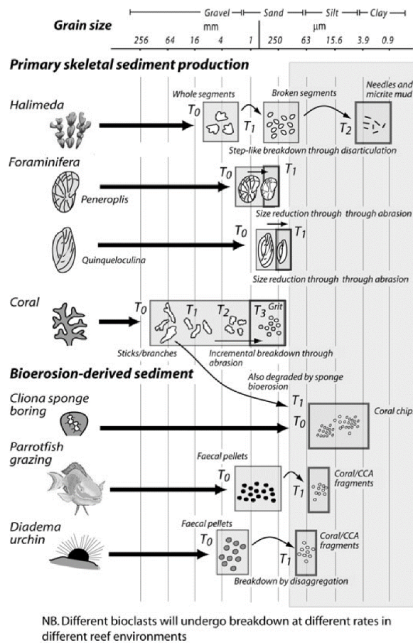
Figure 1-7: Modes de désintégration des particules bioclastiques en fonction de leur origine. La granulométrie d'origine (T 0 ) évolue sous l'action de l'altération vers différentes tailles (T 1 , T 2 , T 3 ) pour aboutir à une granulométrie finale (rectangle en gras). Dans la plupart des systèmes insulaires, des tailles de grains critiques (zone encadrée de gris à droite du diagramme) peuvent être identifiées en dessous de laquelle les sédiments sont peu susceptibles de contribuer à la construction des plages. (Source : Perry et al., 2011)
