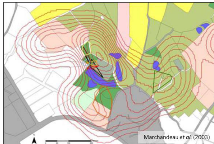
Figure 1.8. Effet spatial d’étangs sur une population de lapins de garenne à partir de l’estimation par noyaux des domaines vitaux dans les Deux-Sèvres par Marchandeaudeau et al. (2003). Les étangs sont représentés en bleu et les autres aplats de couleurs sont l’occupation du sol en fonction du type de cultures. Les lignes rouges correspondent à la probabilité de présence des lapins : forte probabilité de présence au centre, qui diminue vers l’extérieur.
