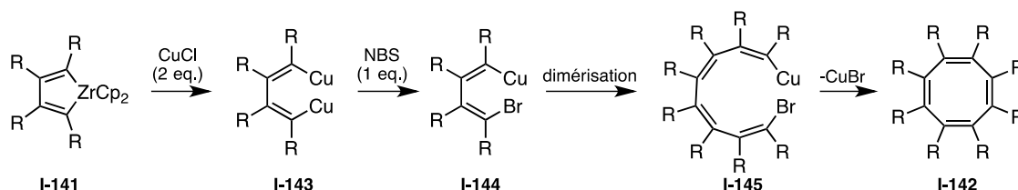
Schéma 44. Mécanisme de formation des COTs I-142 à partir de zirconacyclopentadiènes I-141
