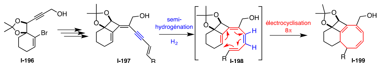
Schéma 62. Stratégie de synthèse de cyclooctatriènes I-199 par semi-hydrogénation de triènes I-197
