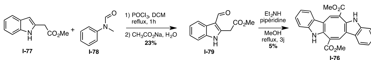
Schéma 23. Synthèse de la Caulerpine I-76 développée par Maiti et al.
