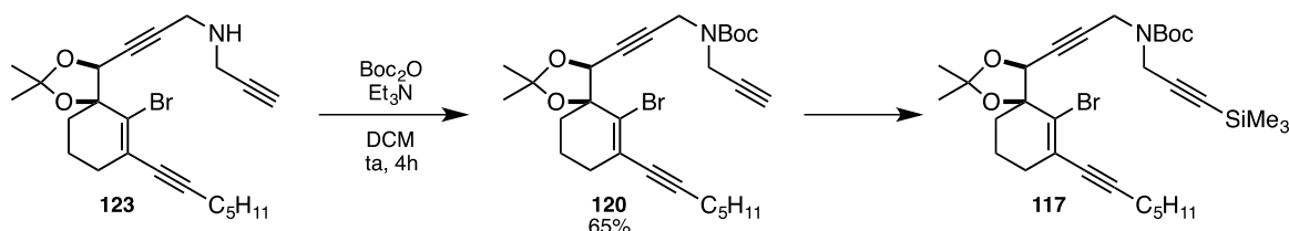
Schéma 154. Synthèse du substrat 117 par protection de l'amine libre 123 puis silylation de l'alcyne terminal 120
