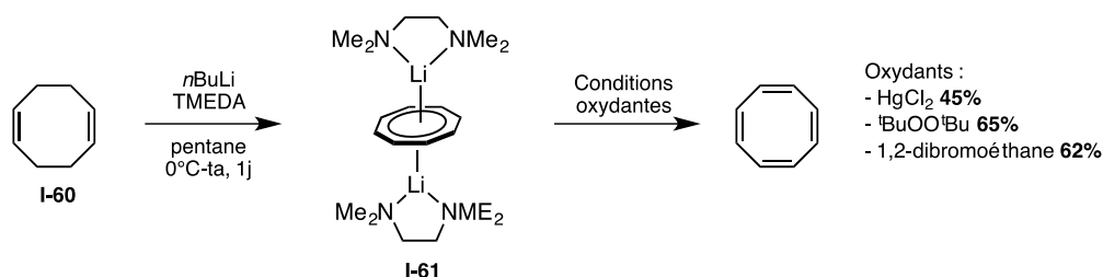
Schéma 16. Synthèse en deux étapes du COT
