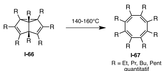
Schéma 19. Réarrangement thermique de semibullvalènes I-66 en COTs I-67 selon Xi et al.
