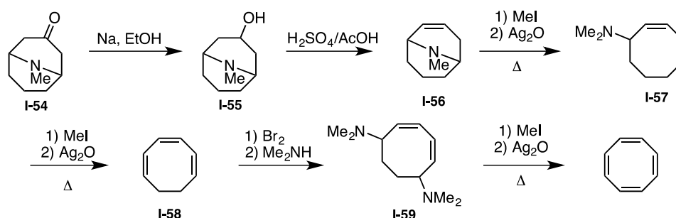
Schéma 14. Première synthèse du COT développée par Willstätter et Waser
