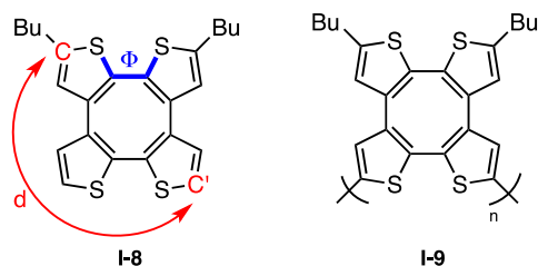
Figure 2. Le monomère cyclooctatétrathiophène et son polymère
