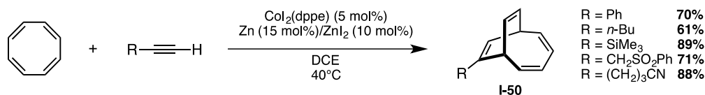
Schéma 12. Cycloaddition [6+2] de COT et d'alcynes vrais selon Bueno et al.
