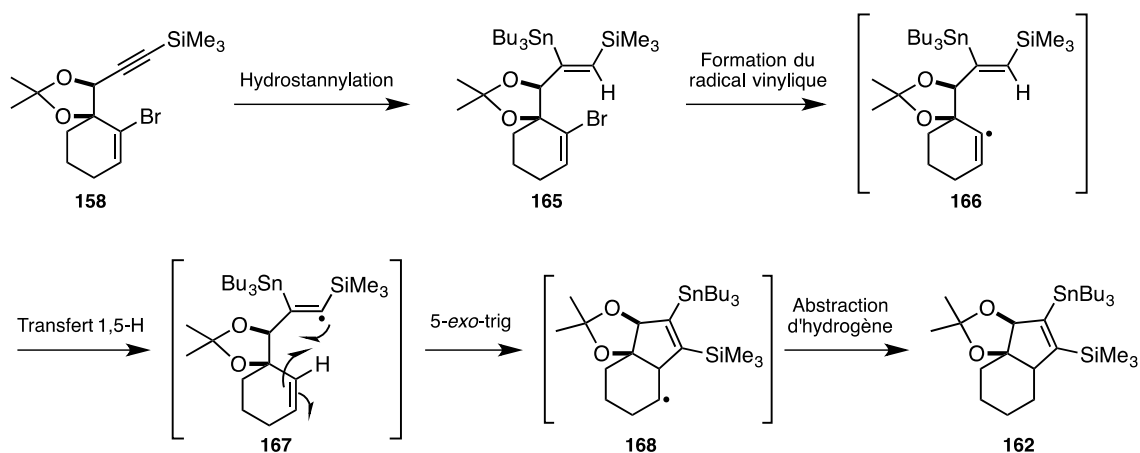
Schéma 167. Mécanisme postulé pour la formation du composé 162
