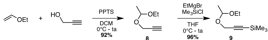
Schéma 78. Synthèse de l'éther propargylique 9
