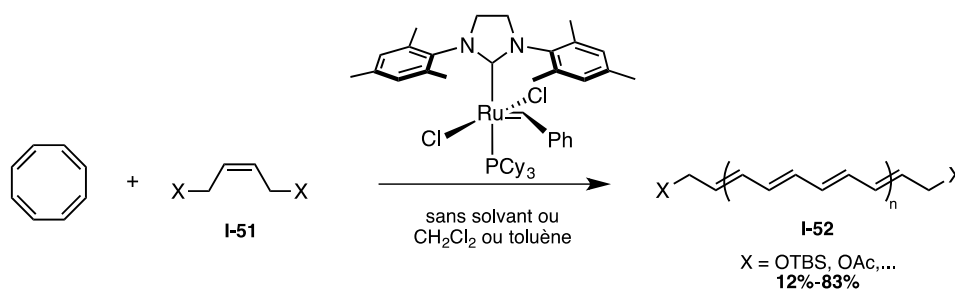
Schéma 13. Polymérisation du COT par ouverture de cycle par métathèse selon Grubbs et al.
