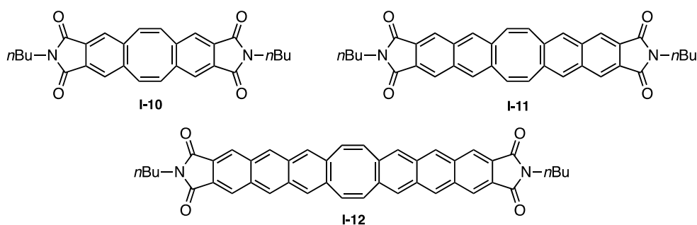
Figure 3. Systèmes \pi multifluorescents changeant de conformation par photoexcitation
