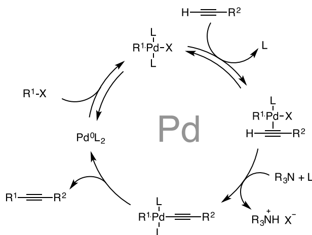
Schéma 81. Mécanisme postulé du couplage de Sonogashira sans cuivre
