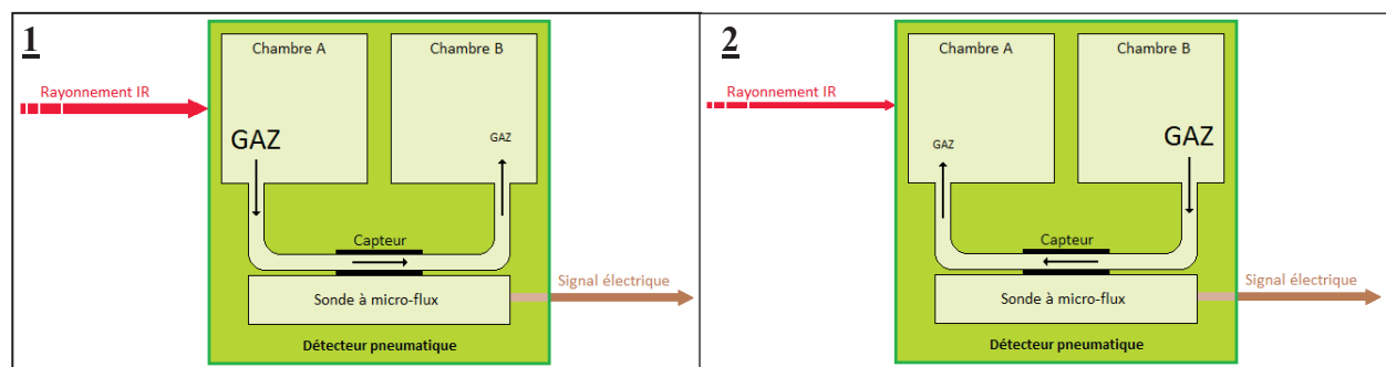
Schéma 4 : Fonctionnement d'un détecteur pneumatique. Chambre A, Chambre d'Absorption ; Chambre B, Chambre de compensation. 1 , Rayonnement infrarouge (IR) issu de la cellule « référence ». 2 , Rayonnement infrarouge (IR) issu de la cellule « échantillon » dans le cadre d'une mesure de respiration.
