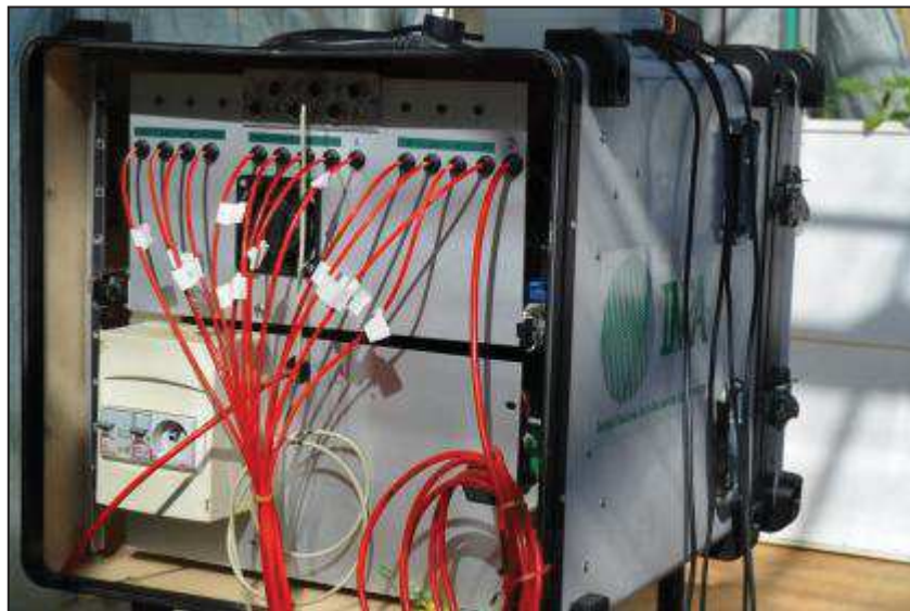
Image 2 : Caisson contenant l'appareillage électronique et l'analyseur de gaz (vue arrière).
