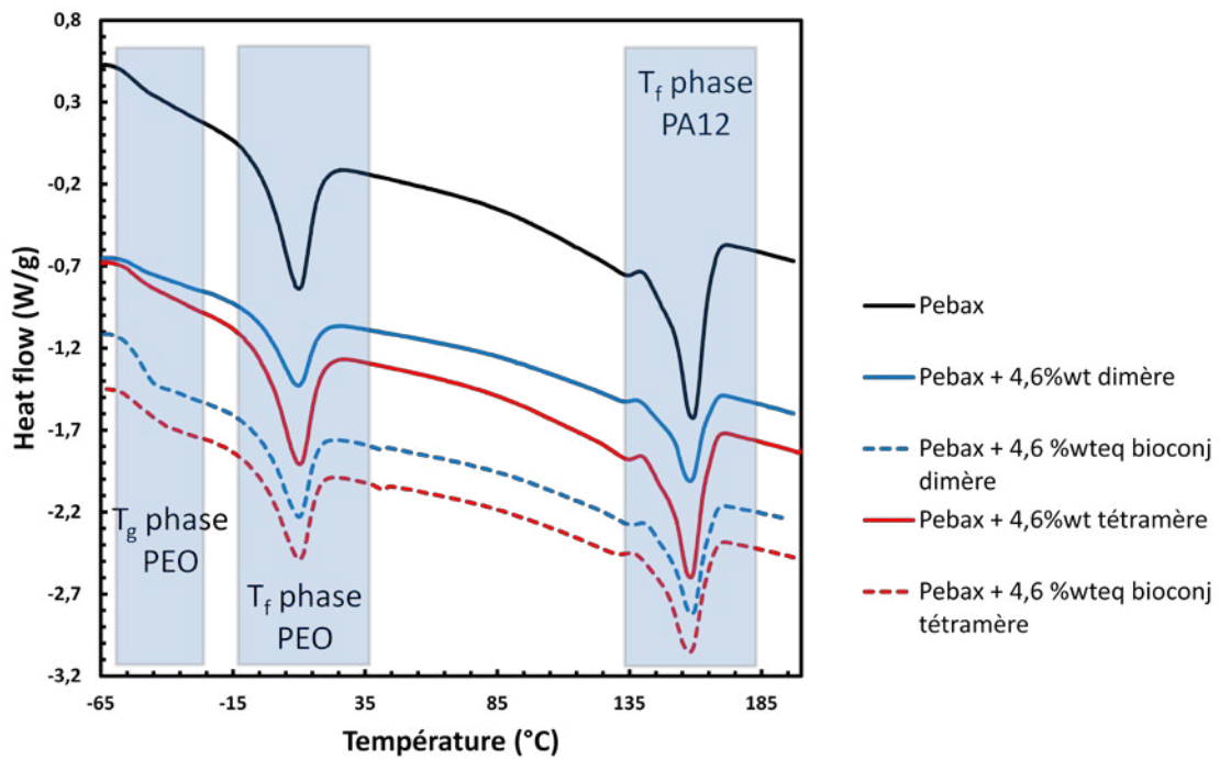
Figure 73 – Thermogrammes des membranes Pebax® additivées avec taux maximal d'additifs pseudopeptidiques. Chauffé à 10 °C/min de -80 °C à 200 °C (cycle 2).
