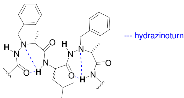
Figure 46 - Structuration par hydrazinoturn au sein des oligomères 1:1[ \alpha/\alpha -N ^{\alpha} -Bn-hydrazino] déterminée dans le CDCl 3 138,139 .
