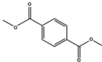
Figure 15 - Motif répétitif diméthyltéréphtalate T 51
