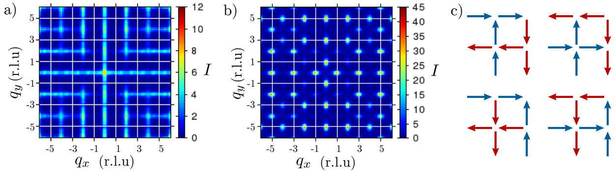
FIGURE 4.11 – Comparaison des facteurs de structure obtenus après désaimantation numérique d'un réseau de 12800 spins avec h = 1 . a) Termes dipolaires J_1, J_2 seulement (phase F). b) Termes dipolaires jusqu'à r_c = 6 (phase M). c) Représentation de la maille unité pour les quatre états Manhattan dégénérés.
