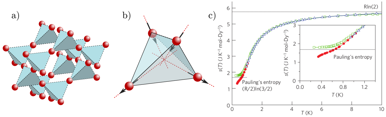
FIGURE 1.6 – a) Schéma du réseau pyrochlore, constitué de tétraèdres connectés par leurs sommets. Dans les glaces de spin, les atomes de terres rares (en rouge) sont situés aux angles des tétraèdres. b) L'axe de quantification des spins Ising est selon les bissectrices des tétraèdres; ils peuvent pointer vers l'intérieur ou l'extérieur. c) Entropie expérimentale du composé \text{Dy}_2\text{Ti}_2\text{O}_7 , sur une plage de température allant de 0.34 à 12 K. Les points verts et rouges correspondent respectivement aux mesures de Ramirez et de Pomaranski. Extrait de la référence [80].
