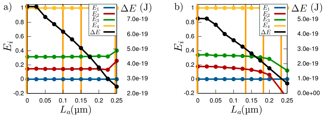
FIGURE 3.16 – Simulations micromagnétiques des niveaux d’énergie des vertex en fonction de L_a , pour la géométrie a) SG et b) LG. L’épaisseur de permalloy est fixée à 3 nm. Les barres verticales oranges représentent les valeurs de L_a réalisées expérimentalement.
