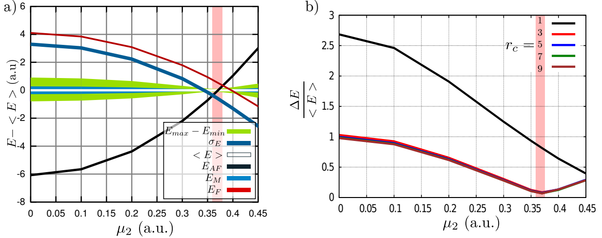
FIGURE 3.10 – a) Graphe équivalent à la figure 3.8 en considérant des interactions entre dipôles de charges jusqu’à r_c = 10 . b) Graphe montrant la différence entre l’énergie maximale et minimale des états étudiés en fonction de \mu_2 . Le tracé est répété pour plusieurs portées r_c . L’énergie est normalisée par rapport à l’énergie moyenne des configurations.
