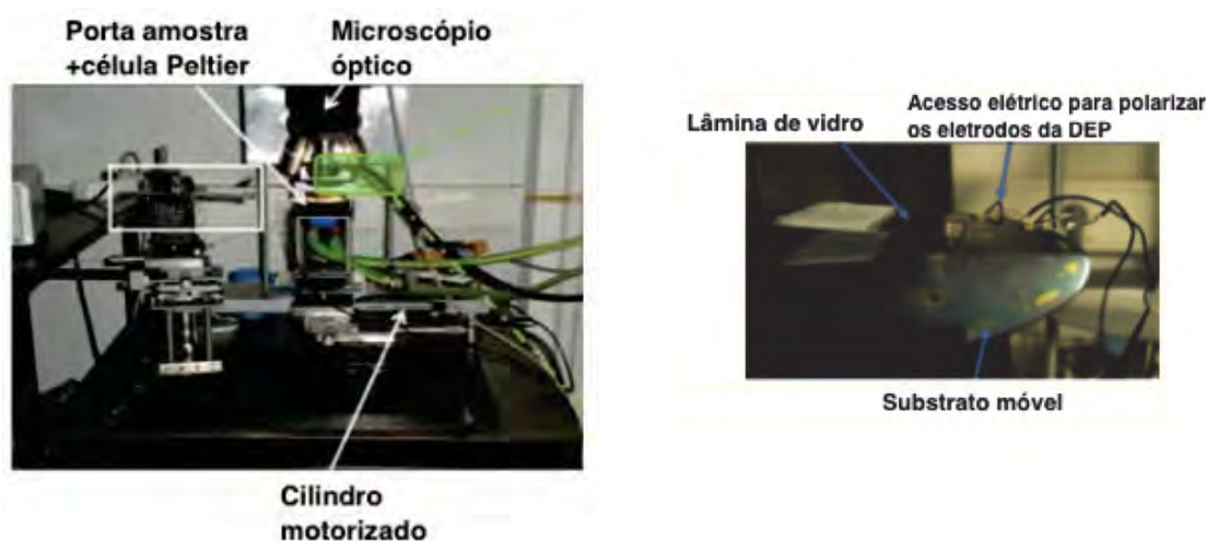
Figura 3.15: Montagem experimental do equipamento utilizado para a realização da dielctroforese acoplada à montagem capilar para alinhamento dos nanofios no substrato de HSQ/SiO 2 /Si [77].
