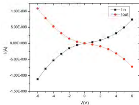
Figure 4.6: IxV de nanofil ZnO avec siliciuration Ni à température ambiante.
