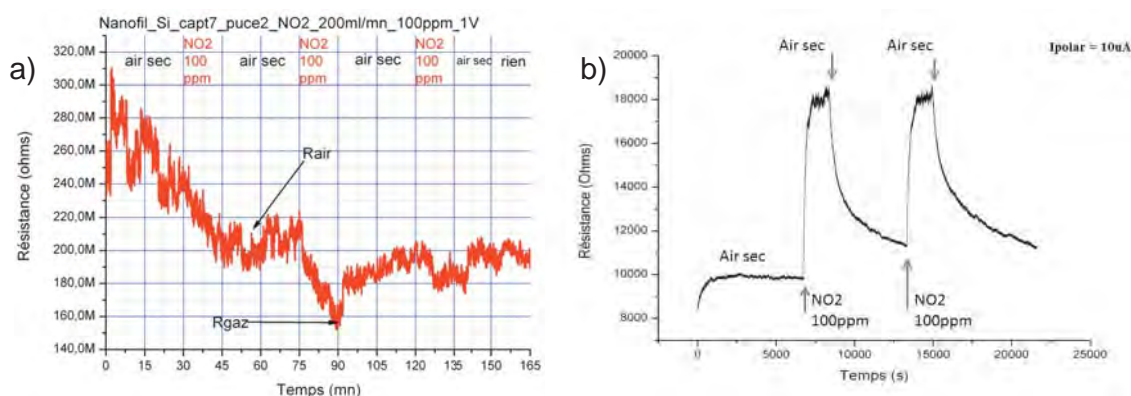
Figure 4.24: Rxt l'application de \text{NO}_2 (100 ppm) pour le fil de a) Si et b) InAs
