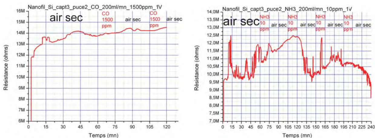
Figura 4.35: Gráfico ( R_{xt} ) de fios de Si, ambos com V = 1V , sob aplicação de diferentes gases, tais como: À esquerda) CO (1500 ppm) e, À direita) \text{NH}_3 (10 ppm)
