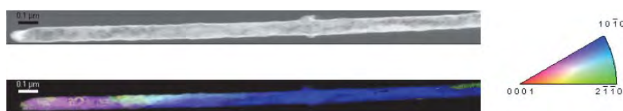
Figure 4.12: L'image en niveaux de gris est une image en champ sombre et l'image couleur présente les différents plans cristallins dans l'échantillon. A côté, la carte d'orientation.
