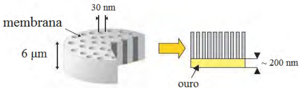
Figura 3.1: À esquerda: membrana de policarbonato com poros de 30 nm de diâmetro e espessura de 6 \mu\text{m} . À direita: deposição de uma camada de ouro com espessura de \sim 200 \text{ nm} [2].
