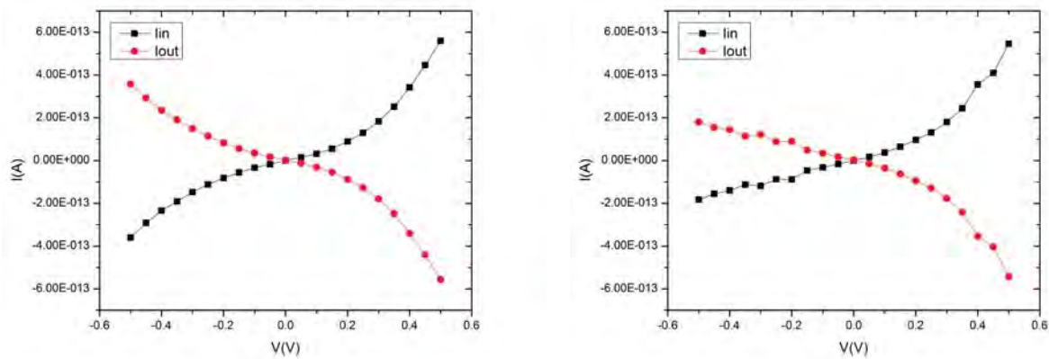
Figura 4.48: À esquerda, medida IxV fio Si. À direita, medida IxV do outro fio em formato de cruz
