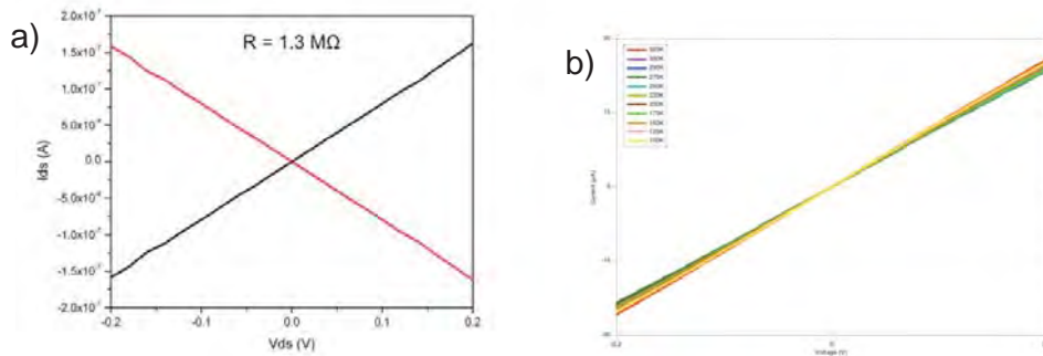
Figure 4.5: a) IxV à température ambiante avec une résistance apparente de 1,3 MΩ. b) IxV à différentes températures.
