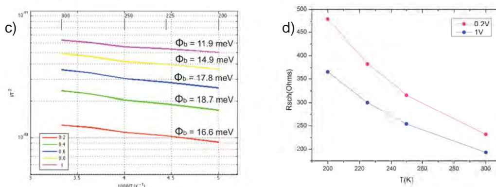
Figure 4.4: a) I \times V à différentes températures; b) Tracé d'Arrhenius, qui à 200 K est l'état off [30]. c) Tracé d'Arrhenius de 300K à 200 K; d) R_{Schottky} en fonction de T pour des fils de Si dopé avec siliciuration Ni.
