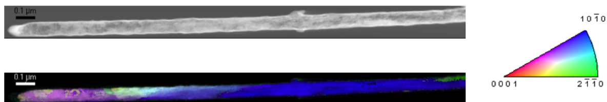
Figura 5.14: A imagem em escala de cinza é uma imagem em bright field virtual e a imagem colorida mostra os diferentes planos cristalinos presentes na amostra. Ao lado, o mapa de orientação.
