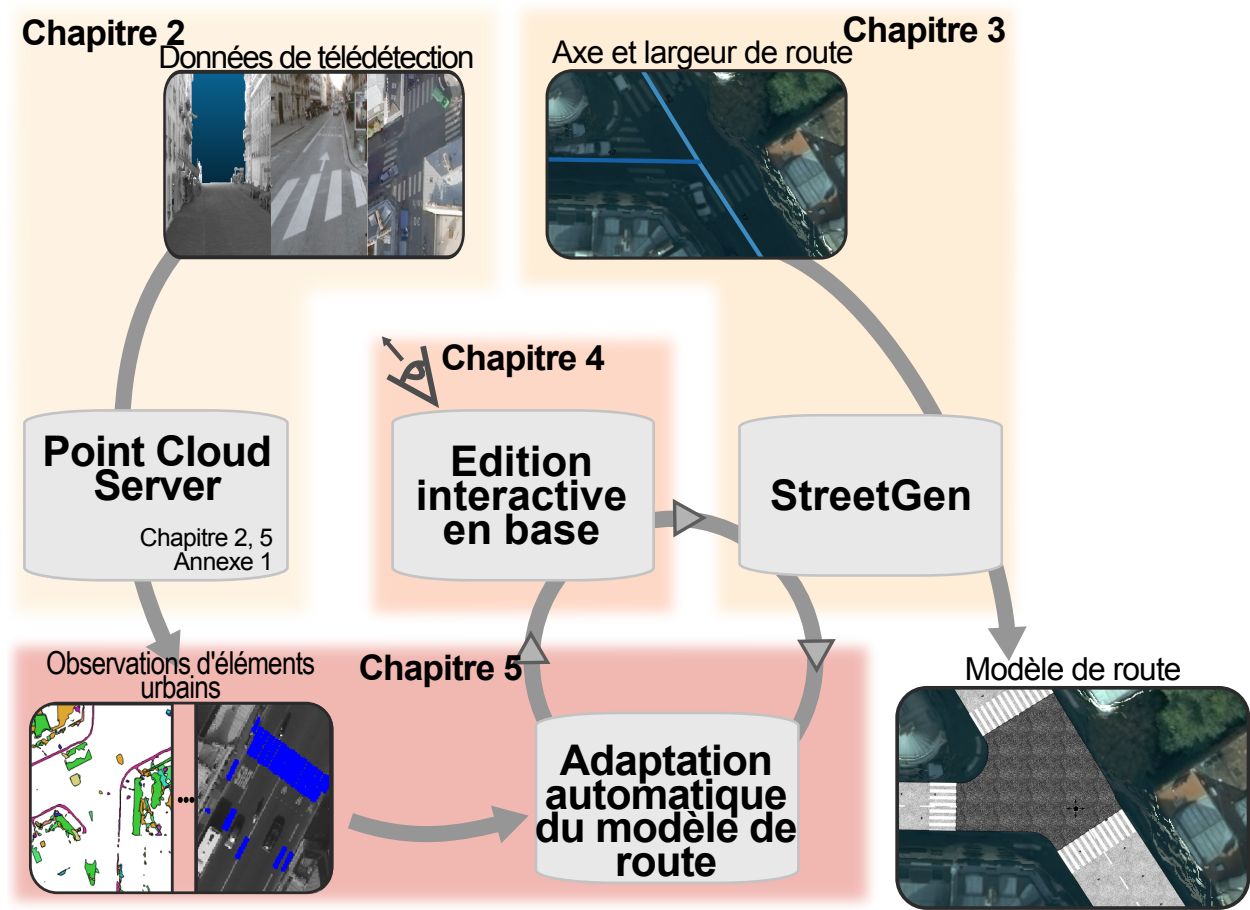
FIGURE 2 : Résumé graphique du travail de la thèse. En partant d'un réseau d'axe routier et de largeur approximatifs, un modèle de rue est généré avec StreetGen (chapitre 3). Ce modèle peut ensuite être interactivement modifié avec tous les logiciels SIG classiques en utilisant l'interaction en base (chapitre 4). En complément, le modèle peut aussi être automatiquement ajusté (chapitre 5) à des observations d'éléments urbains issus de télédétections massives, qui sont gérées dans le serveur de nuage de point (Point Cloud Server) (chapitre 2, annexe A).
