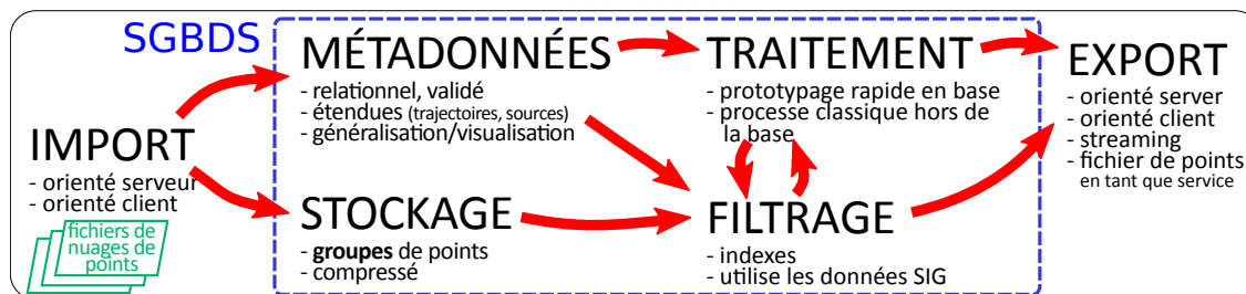
FIGURE 5 : chapitre 2 : gestion de nuages de point en base de données avec le Point Cloud Server (PCS).
