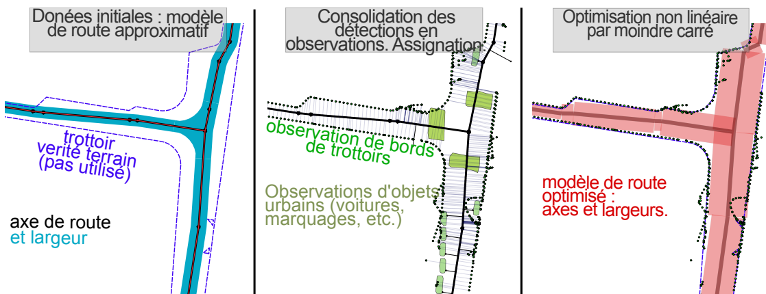
FIGURE 8 : Les données initiales sont des axes de routes et des largeurs de route approximées, ce qui décrit un modèle de route basique. A partir de données de télédétections (image, Lidar), différentes détectations d'éléments caractéristiques de la rue sont extraites (objets urbains, bords de trottoirs, etc.). Ces détectations sont consolidées (filtrage, fusion) en observations, puis assignées à des segments d'axe de route. Une méthode d'optimisation robuste non linéaire par moindres carrés adapte ensuite le modèle aux observations. Le modèle adapté est alors beaucoup plus proche de la réalité, même quand notre modèle de route est trop simple pour une situation complexe (route de largeur variable, changements de trottoir asymétriques, courbes). L'utilisateur peut de plus ajouter des observations manuellement si nécessaire.
