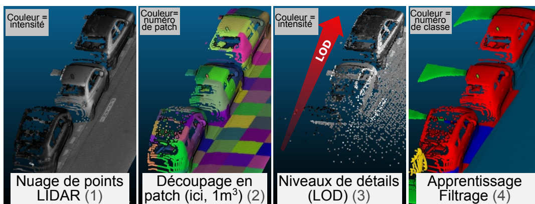
FIGURE 9 : (1) Les nuages de points initiaux sont denses et contiennent beaucoup de points. (2) Les nuages sont découpés en patches et stockés dans le Point Cloud Server. (3) Les patches sont ré-ordonnés selon un ordre de LOD implicite (illustré ici avec un gradient continu). (4) Le nouvel ordonnancement produit un descripteur de dimensionnalité multi-échelles utilisé comme descripteur pour de l'apprentissage et du filtrage.
