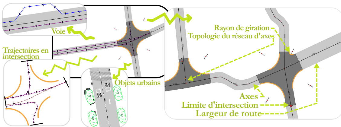
FIGURE 7 : Nous proposons de gérer l'interaction directement dans la base de données plutôt que dans un logiciel spécifique. Le modèle de rue (StreetGen) est re-généré automatiquement lorsque l'utilisateur édite les paramètres du modèle à l'aide d'interacteurs pratiques. Le modèle de route, les informations de trafic et les objets urbains peuvent être édités.
