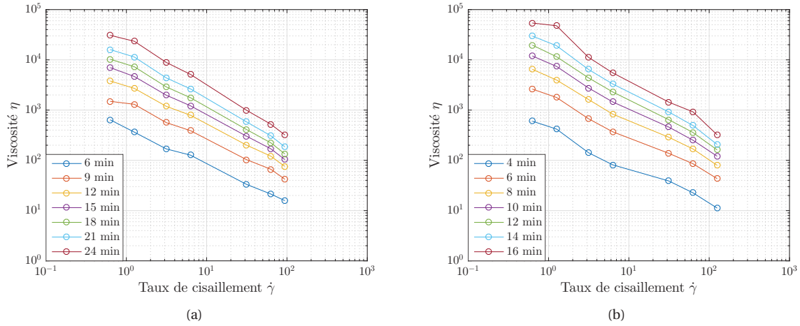
Figure D.5 – Courbes de viscosité représentées sur une échelle logarithmique : (a) à T_0 = 20\text{ °C} ; (b) à T_0 = 25\text{ °C} .
