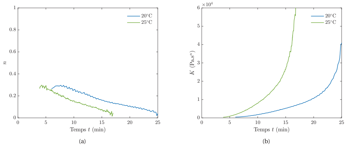
Figure D.6 – Identification des paramètres n et K de la loi puissance en fonction du temps à T_0 = 20\text{ °C} (courbe bleue) et à T_0 = 25\text{ °C} (courbe verte).
