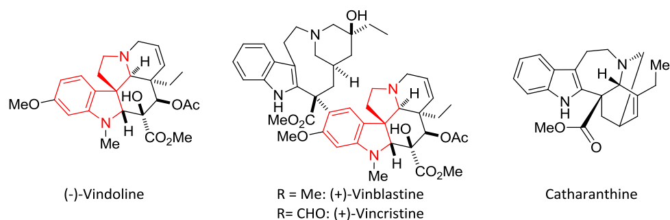
Figure 4 : Vinca-alcaloïdes
