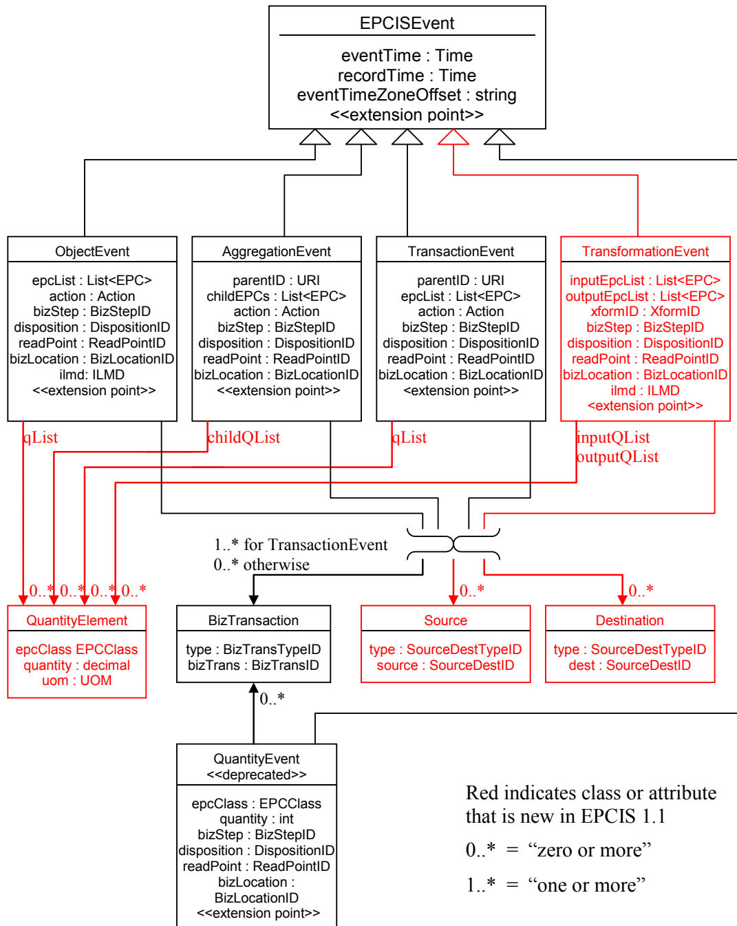
FIGURE 2.2 – Description des notions utilisées par le protocole EPCIS
