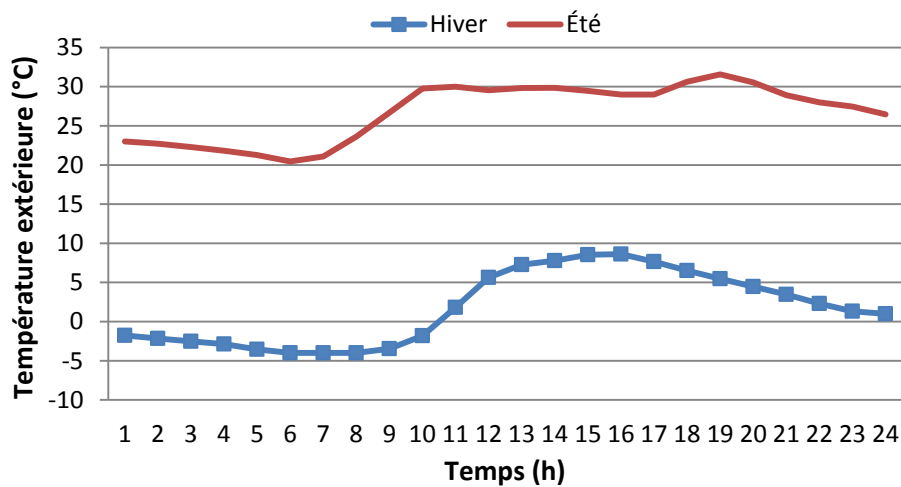
Figure IV.14. Température extérieure
