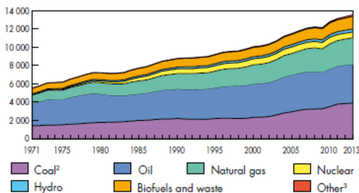
Figure I.3. Consommation mondiale d'énergie primaire de 1971 à 2013 en Mtep
