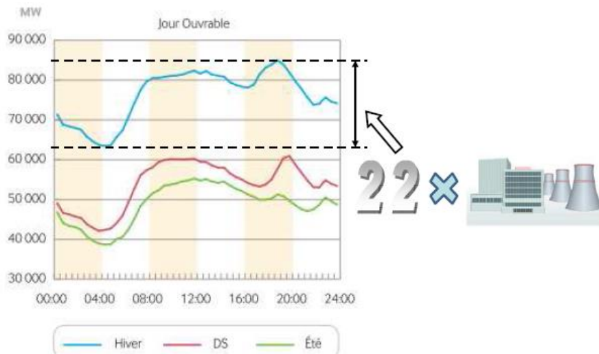
Figure I.7 Consommations typiques journalières en été, en demi-saison (DS) et en hiver.
