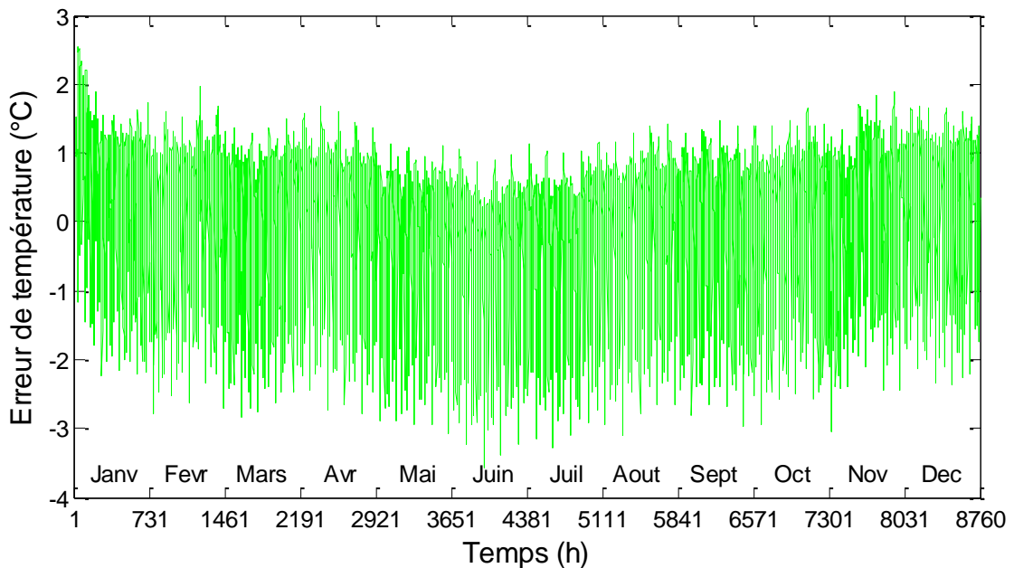
Figure IV.6. Ecart de température entre le modèle RC et le modèle EnergyPlus. Durée de simulation : 1 année (8760 heures) ; Données météo : Carpentras
