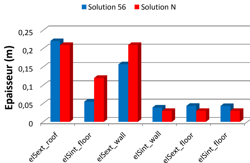
Figure II.8 Solutions optimales de l'épaisseur de l'isolation thermique obtenues par les optimisations continues et discrètes : Solution 56 (continue) & Solution N (discrète)
