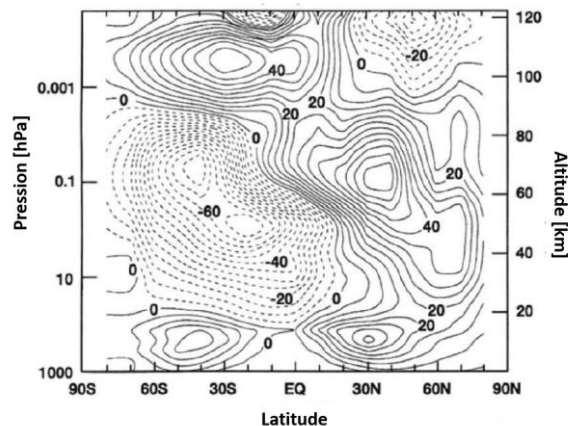
Figure 2.17 : Vitesses de vents zonaux moyens exprimés en m.s -1 (Holton et al., 1995)
