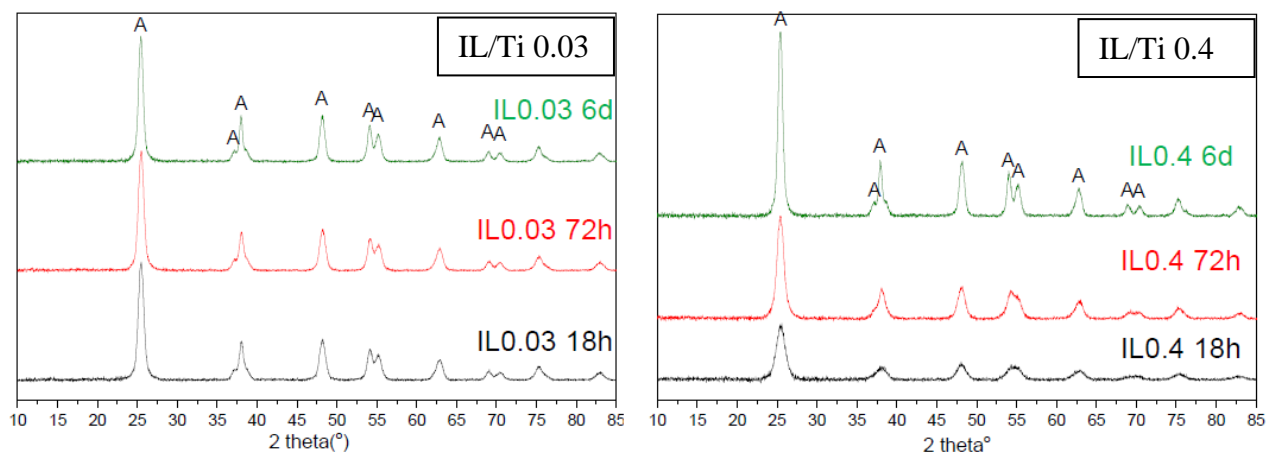
Figure 5 : Influence de la durée de murissement sur la cristallinité de \text{TiO}_2 synthétisé avec un ratio molaire \text{BmimPF}_6/\text{Ti} 0.03 et 0.4 après calcination à 550\text{ }^\circ\text{C} .
