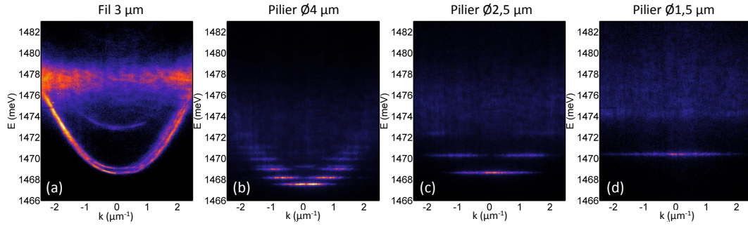
FIGURE 4.30 – Émission de polaritons résolue en angle et en énergie dans une cavité gravée ( 1 puits InGaAs, \mathcal{Q} \sim 30000 ) selon différentes géométries. La mesure est effectuée pour un fil de 3 \mu\text{m} de large (a) et des piliers circulaires de diamètre 4 \mu\text{m} (b), 2,5 \mu\text{m} (c) et 1,5 \mu\text{m} (d).
