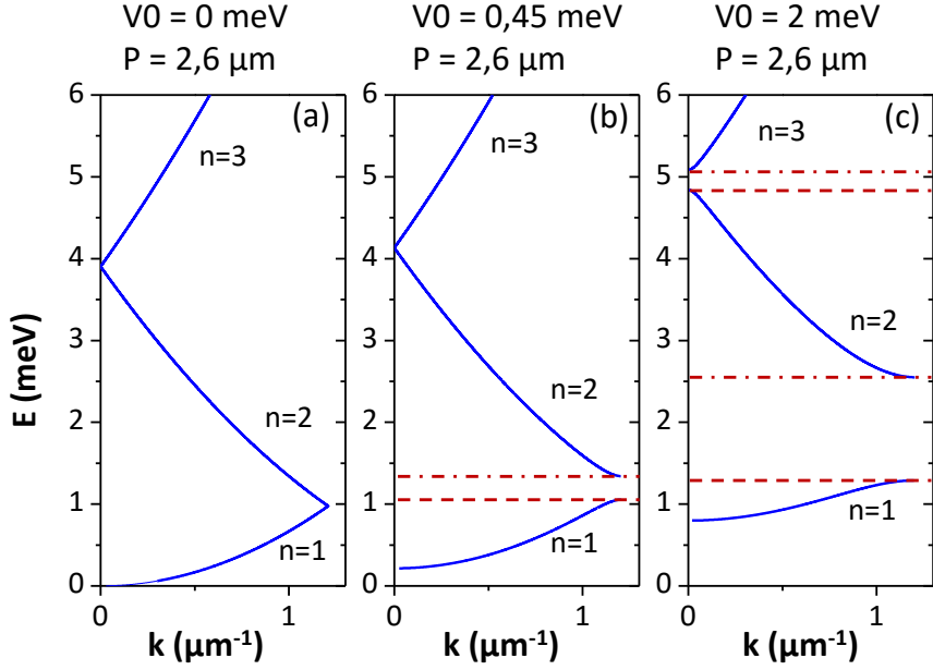
FIGURE 3.2 – (a-c) Structure de bande d’un potentiel carré périodique calculée à partir du modèle de Kroenig-Penney pour m_p = 5,7 \times 10^{-5} m_e , P = 2,6 \mu\text{m} et (a) V_0 = 0 \text{ meV} , (b) 0,45 \text{ meV} , (c) 2 \text{ meV} .
