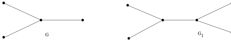
Figure 4.4: Ajout d'un cycle
