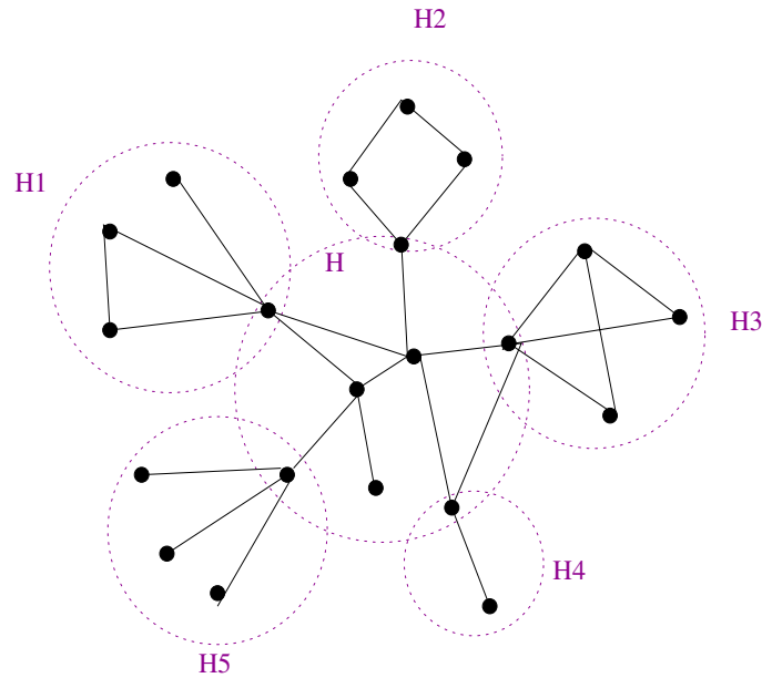
Figure 4.3: Graphe H-type-fleur
