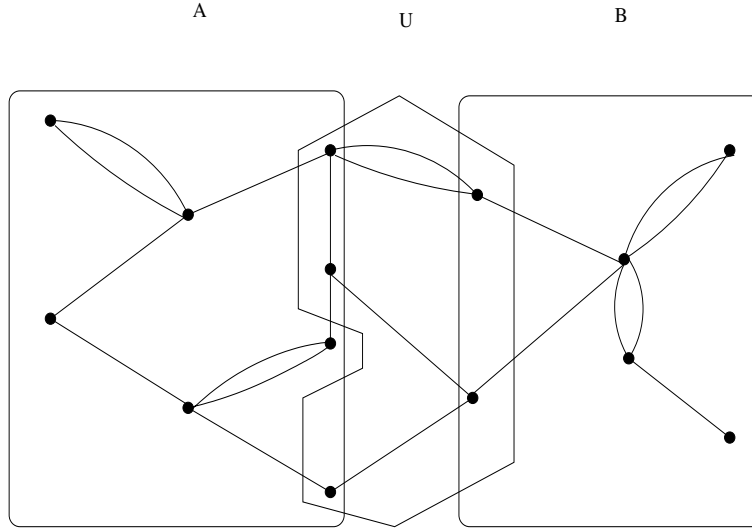
Figure 4.6: Les parties A , U et B dans le graphe G .
