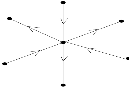
Figure 2.4: Le graphe en étoile S_6
