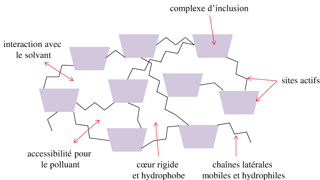
Figure 35. Structure tridimensionnelle d'un matériau à base de CDs (Morin-Crini et al. 2015b).
