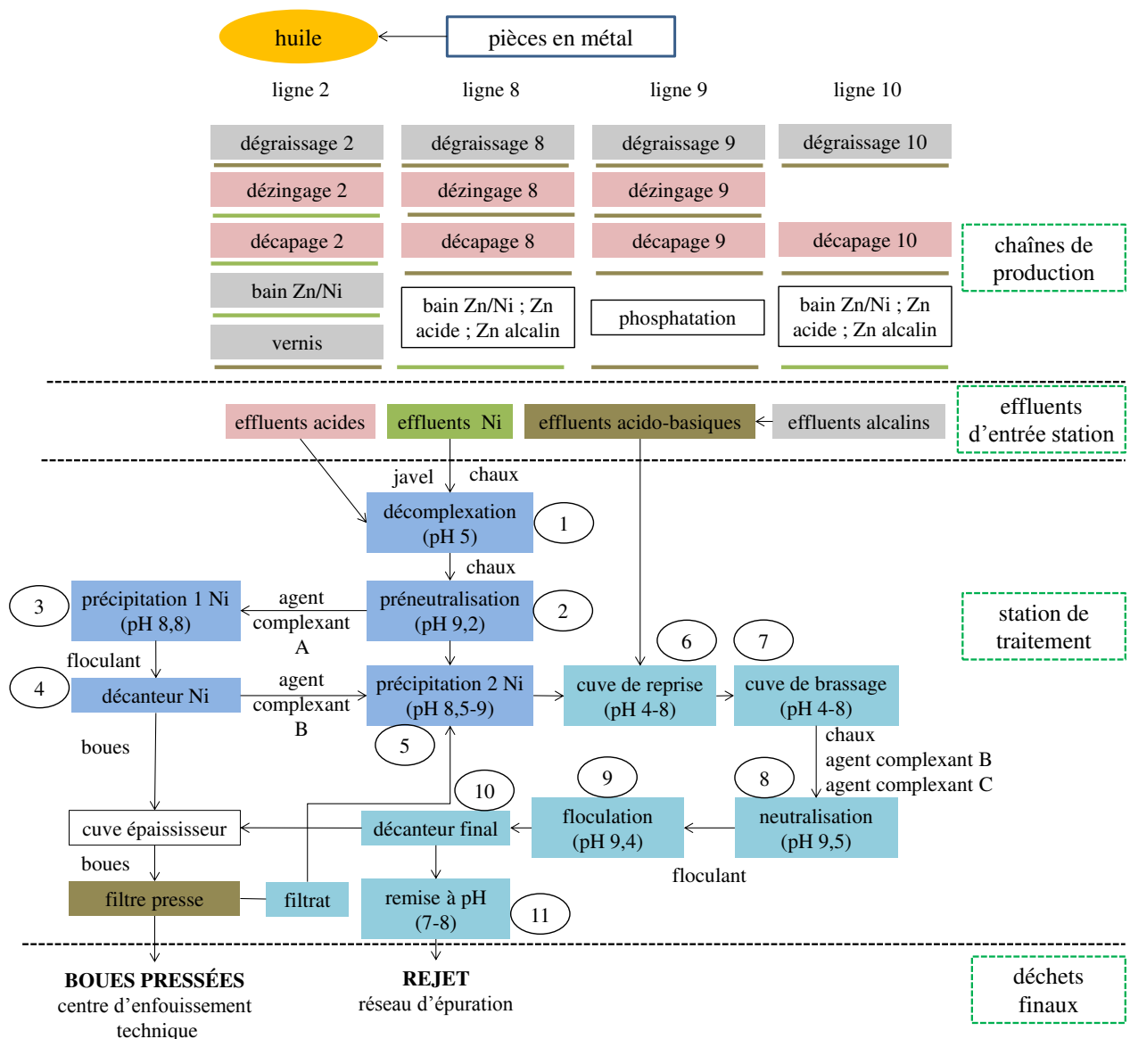
Figure 58. Vue d'ensemble de l'atelier de production et de la station de traitement des eaux usées de l'entreprise Zindel (chaque case colorée représente un point d'échantillonnage).
