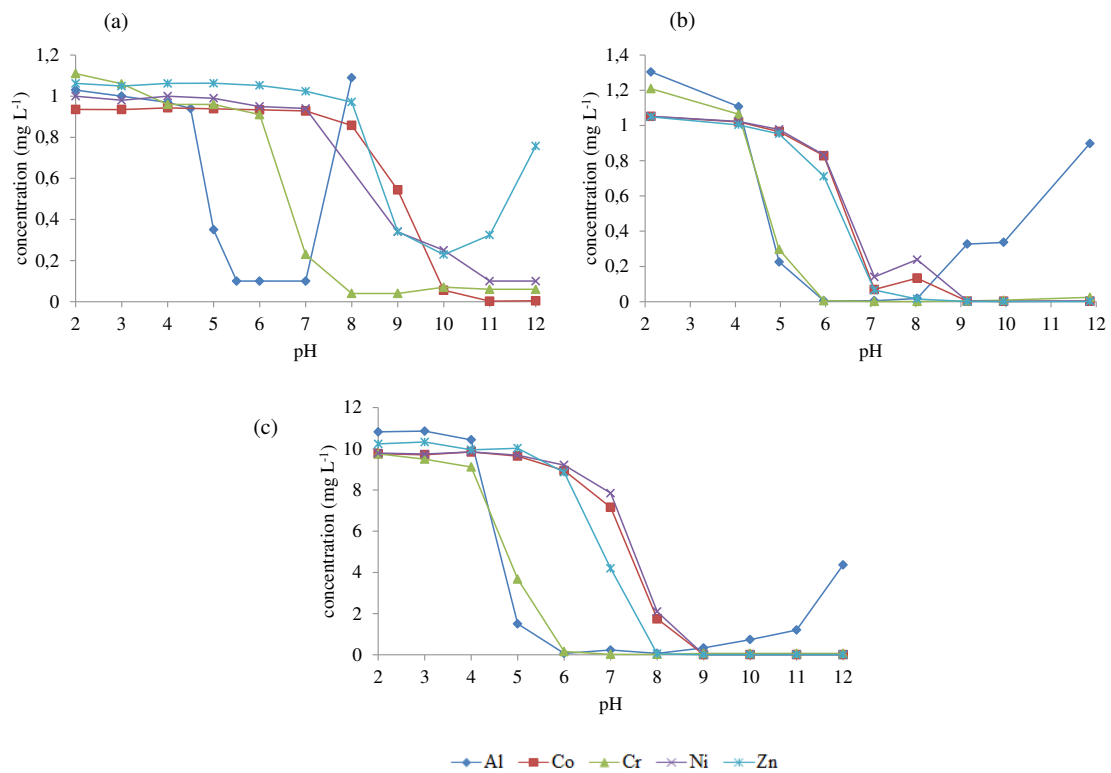
Figure 94. Courbes de précipitation des 5 métaux : (a) seul ( 1 \text{ mg L}^{-1} ) et en mélange à (b) 1 \text{ mg L}^{-1} et (c) 10 \text{ mg L}^{-1} .
