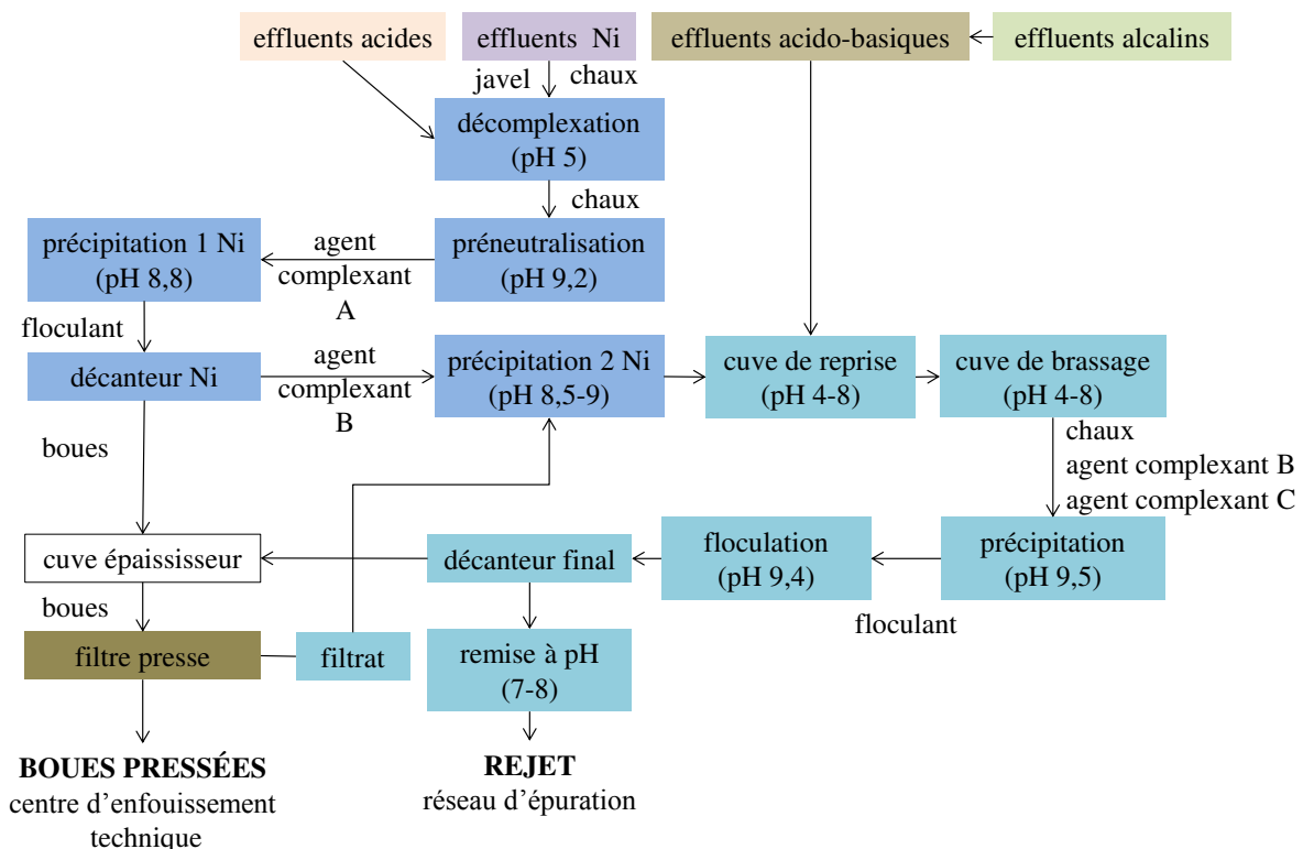
Figure 40. Schéma de la station de traitement des eaux de Zindel (2012).
