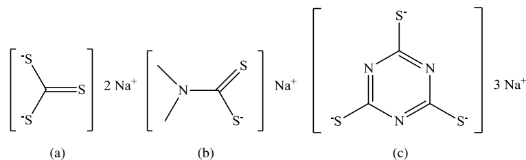
Figure 19. Formules chimiques du (a) thiocarbonate de sodium, (b) diméthylthiocarbamate de sodium et (c) trimercaptotriazine.
