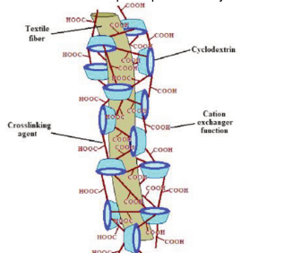
Fig. 1 : structure d'une fibre non tissée de PET fonctionnalisée avec le BTCA et de la β-CD [1]
