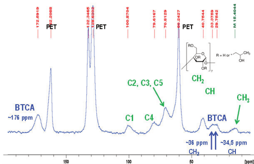
Figure 81. Interprétation des bandes du spectre CPMAS du PET BTCA-CD (en vert les carbones de l'unité glucose de la CD et en bleu les carbones du BTCA).
