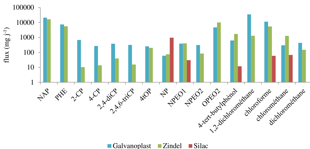
Figure 57. Flux ( g j^{-1} ) des principales substances organiques pour Galvanoplast (débit moyen de 199 m^3 j^{-1} ), Silac ( 66 m^3 j^{-1} ) et Zindel ( 172 m^3 j^{-1} ).
