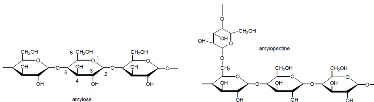
Figure 28. Structures de l'amylose et de l'amylopectine.
