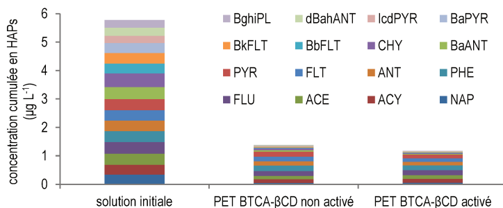
Fig. 2 : variation de la concentration de 16 HAPs en solution synthétique en fonction de l'activation des fibres de PET-BTCA-βCD
