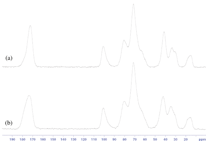
Figure 76. Spectres MAS des polyBTCA-CD acide (a) et basique (b).
