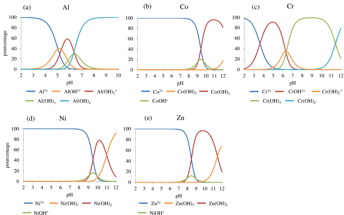
Figure 95. Principales espèces présentes dans l'eau en fonction du pH pour les 5 métaux seuls ( 1 \text{ mg L}^{-1} ), (a) Al, (b) Co, (c) Cr, (d) Ni et (e) Zn (courbes théoriques réalisées via le logiciel Visual Minteq).
