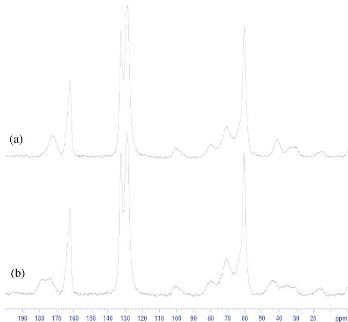
Figure 82. Spectre CPMAS du PET BTCA-CD (a) acide et (b) basique.
