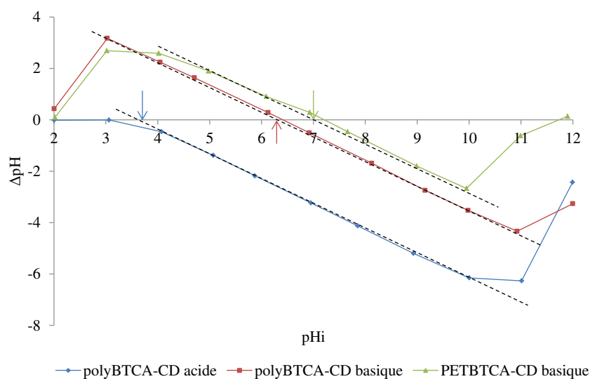
Figure 70. Détermination du pH_{pcn} pour les différents matériaux.
