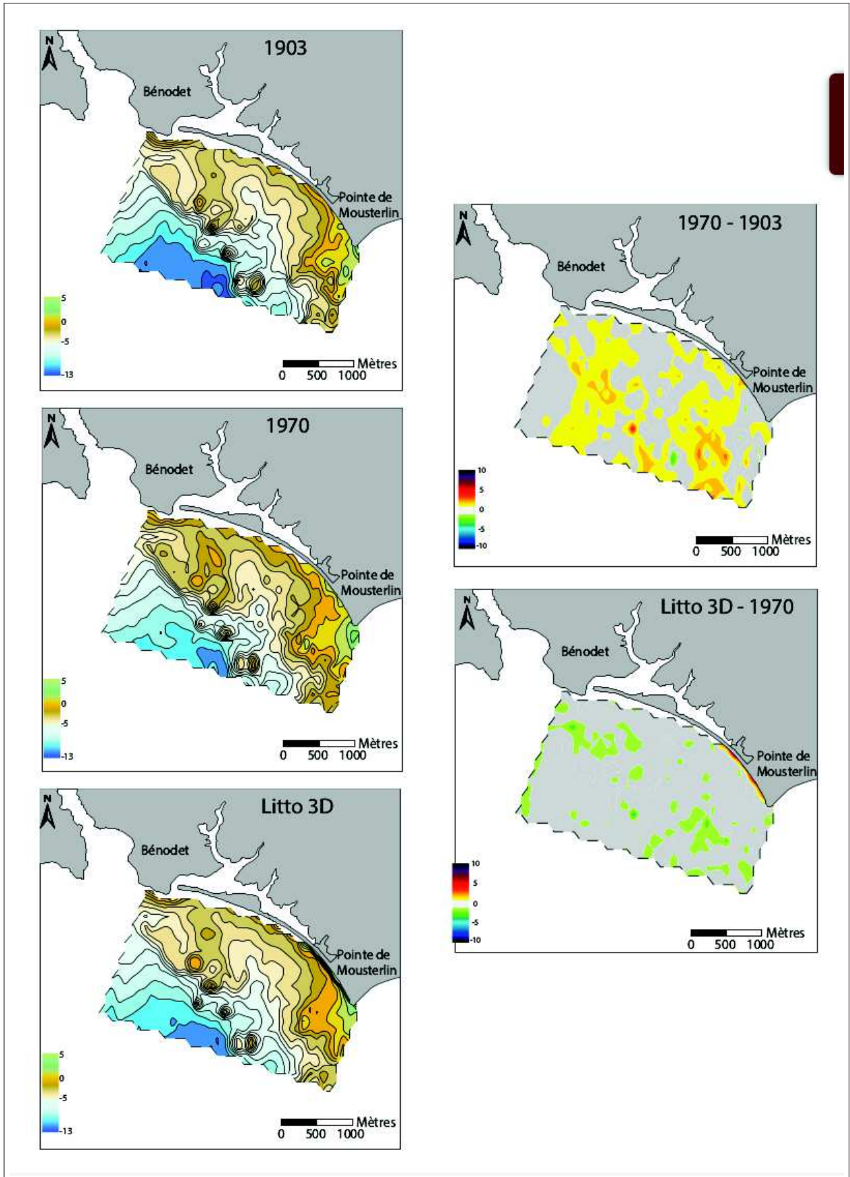
FIGURE 2.31 – Zone 3 secteur est : MNT et MNT différentiels (échelle de couleur : dégradé jaune-rouge = accrétion et dégradé vert-bleu = érosion)
