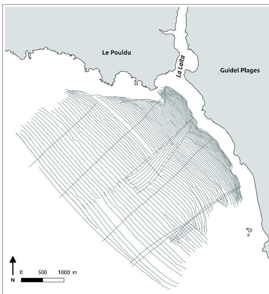
FIGURE 3.23 – Profils sismiques réalisés sur le secteur de Guidel durant la mission Fissel 4.
