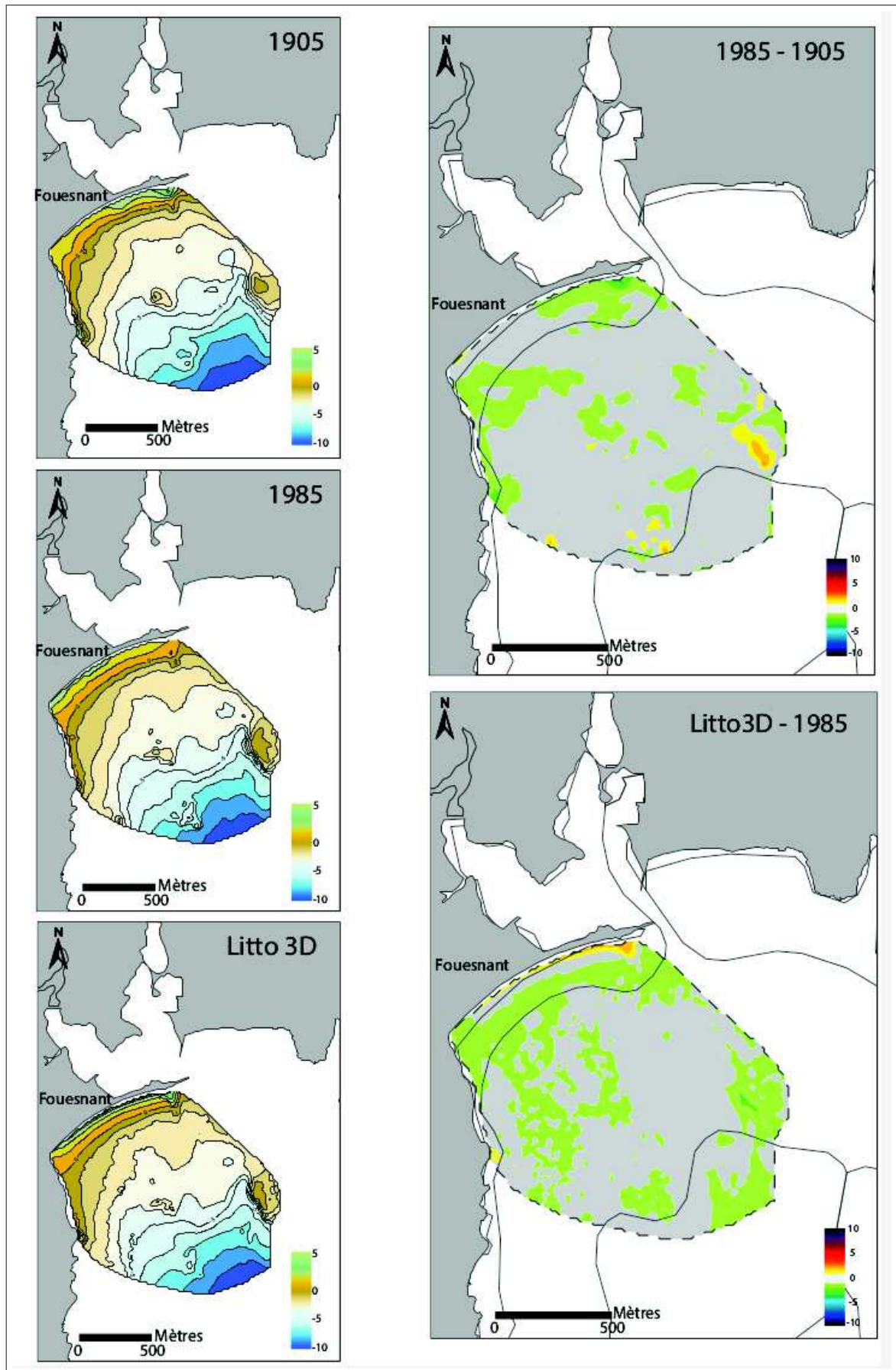
FIGURE 2.27 – Zone 2 : MNT et MNT différentiels (échelle de couleur : dégradé jaune-rouge = accrétion et dégradé vert-bleu = érosion)
