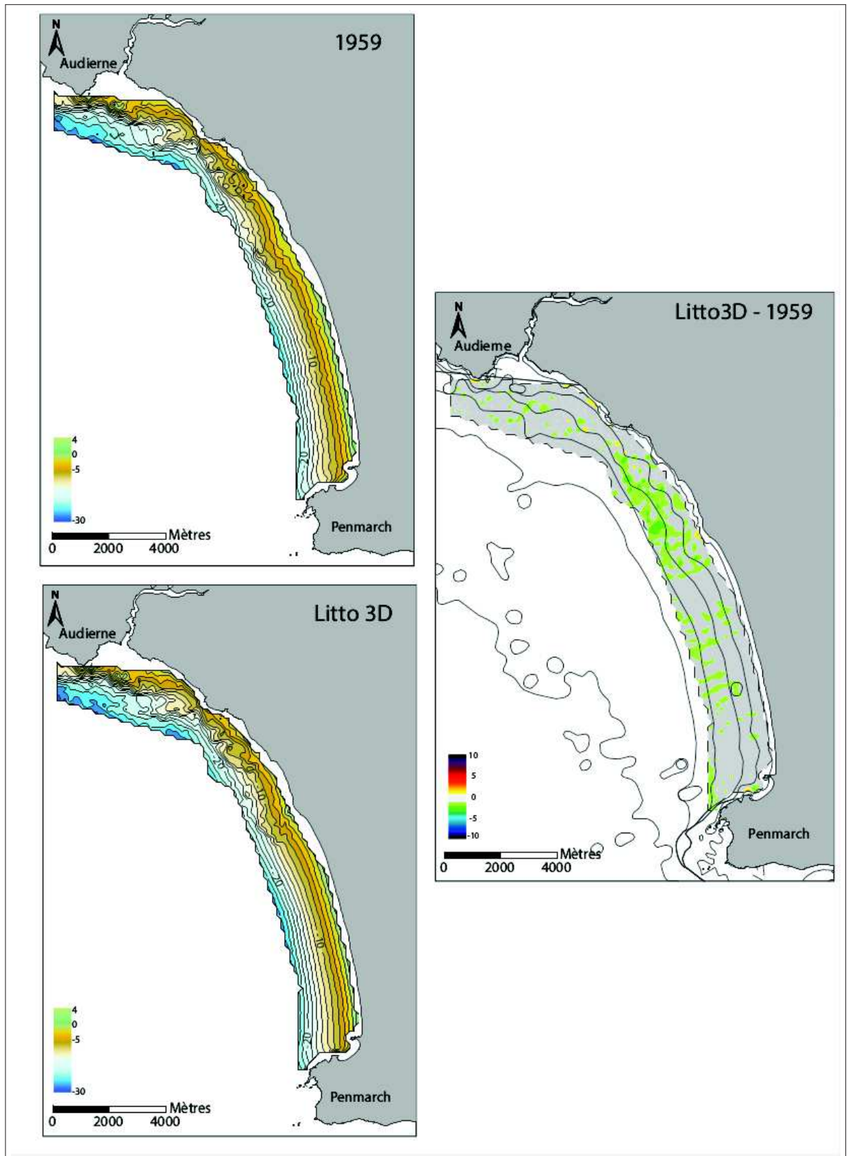
FIGURE 2.34 – Zone 4 : MNT et MNT différentiels (échelle de couleur : dégradé jaune-rouge = accrétion et dégradé vert-bleu = érosion)
