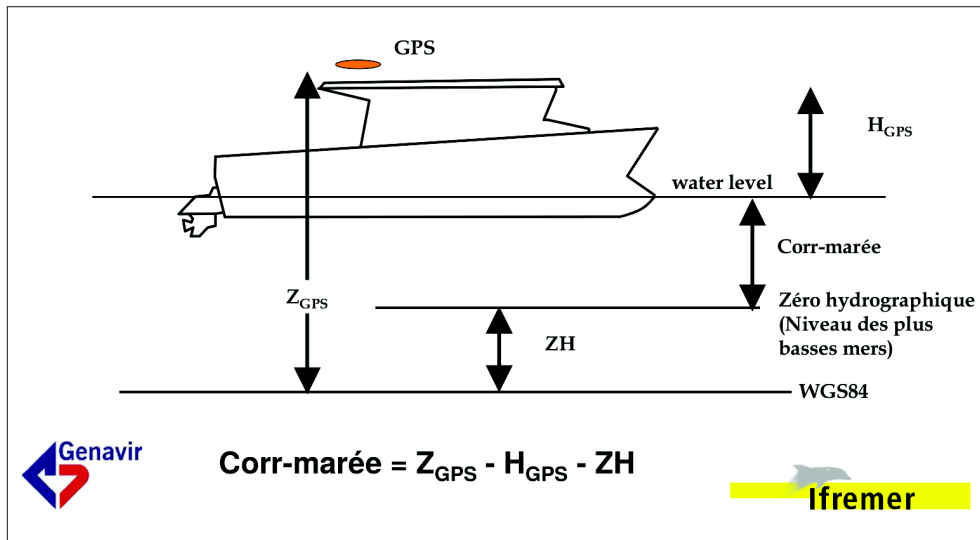
FIGURE 3.2 – Exploitation du Z RTK pour la correction de la marée, avec Z GPS : Mesure GPS (par rapport à l'ellipsoïde WGS84) moyennée sur trois minutes, afin de s'affranchir des variations à court terme (pilonnement) ; H GPS : Hauteur de l'antenne GPS au-dessus du niveau de l'eau ; ZH : Hauteur du zéro hydrographique au-dessus de l'ellipsoïde WGS84 (Source : Genavir, Ifremer).
