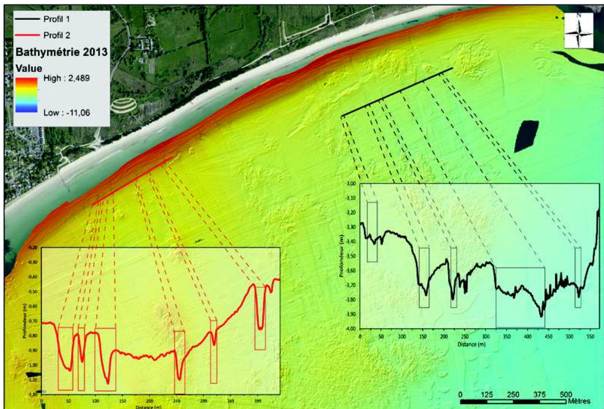
FIGURE 3.37 – Profils transverses à la côte d'un groupe de sillons
