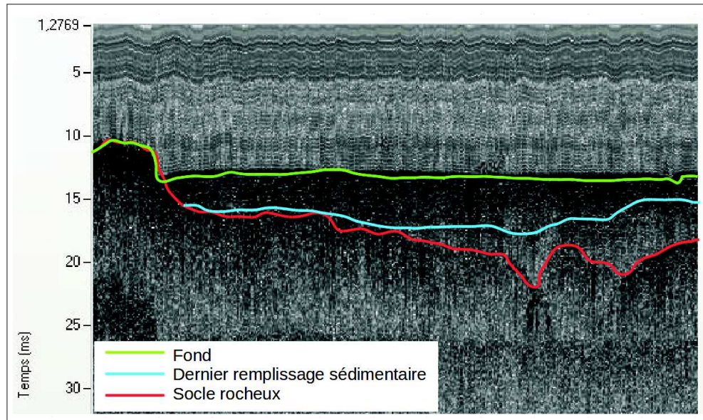
FIGURE 3.4 – Exemple de numérisation des différents horizons (mission Haliotis 2015 sur le secteur de l'anse du Pouldu).
