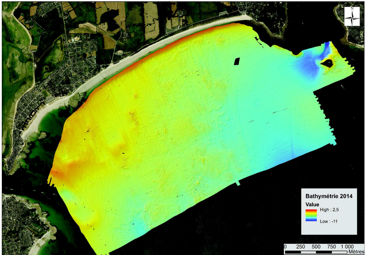
FIGURE 3.10 – Bathymétrie de 2014 sur le secteur de Combrit - Île-Tudy.
