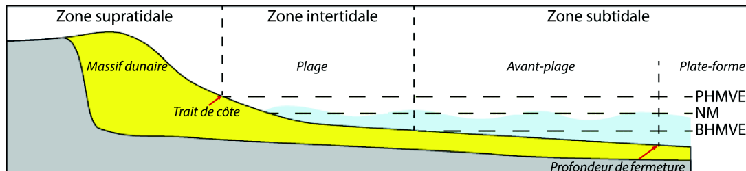
FIGURE 1.5 – Les différentes unités de la cellule littorale et leurs limites (PHMVE : Plus Hautes Mers de Vives-Eaux, BHMVE : Plus Basses Mers de Vives-Eaux et NM : Niveau Moyen).
