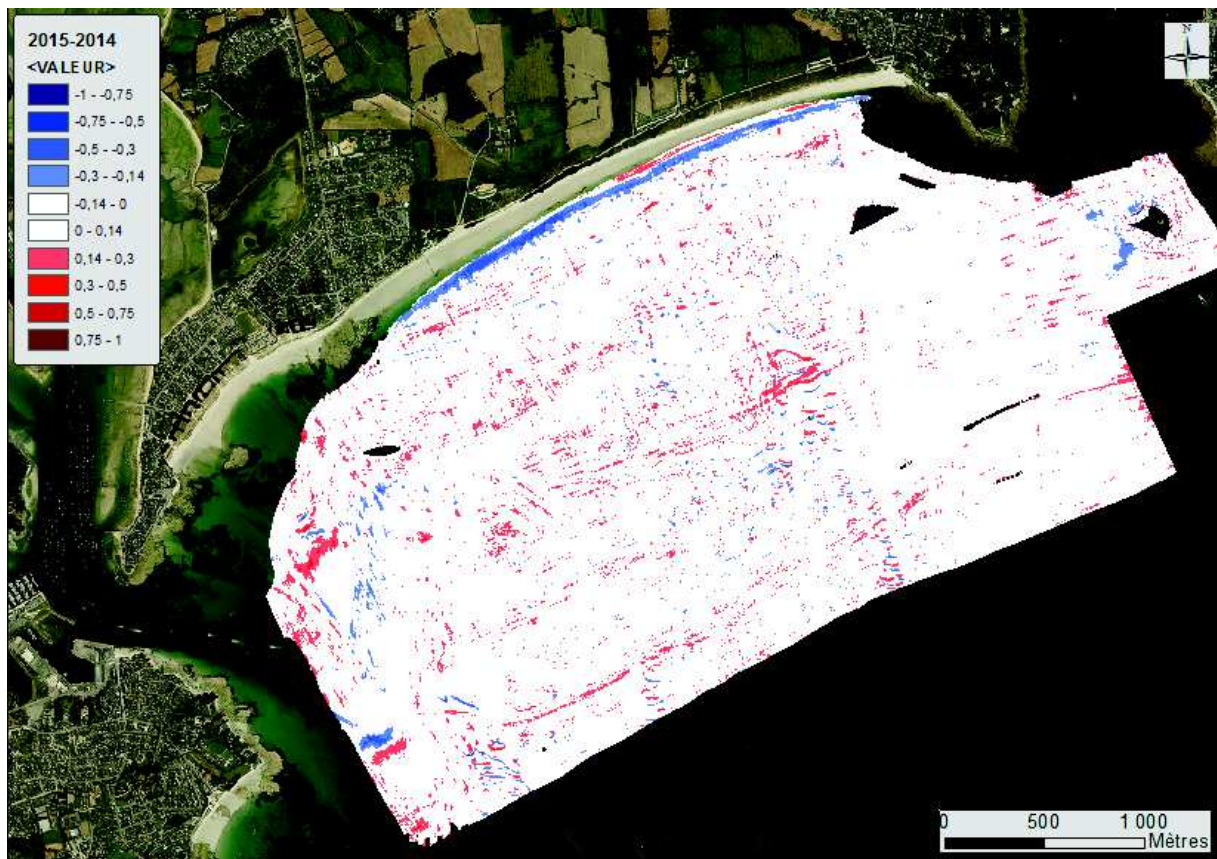
FIGURE 3.16 – Évolutions de la bathymétrie entre 2014 et 2015.
