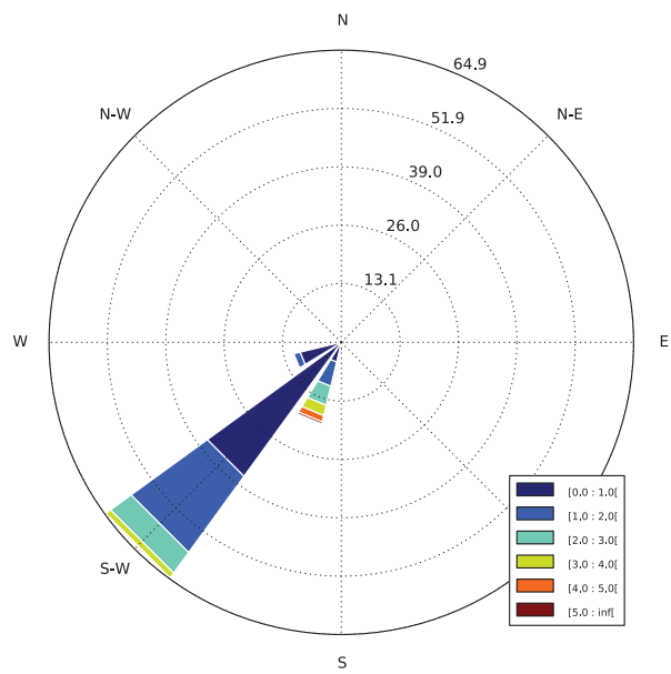
FIGURE .16 – Rose des houles au point 3898.
