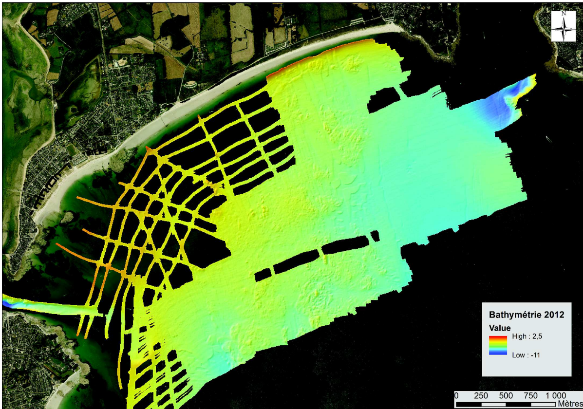
FIGURE 3.8 – Bathymétrie de 2012 sur le secteur de Combrit - Île-Tudy.
