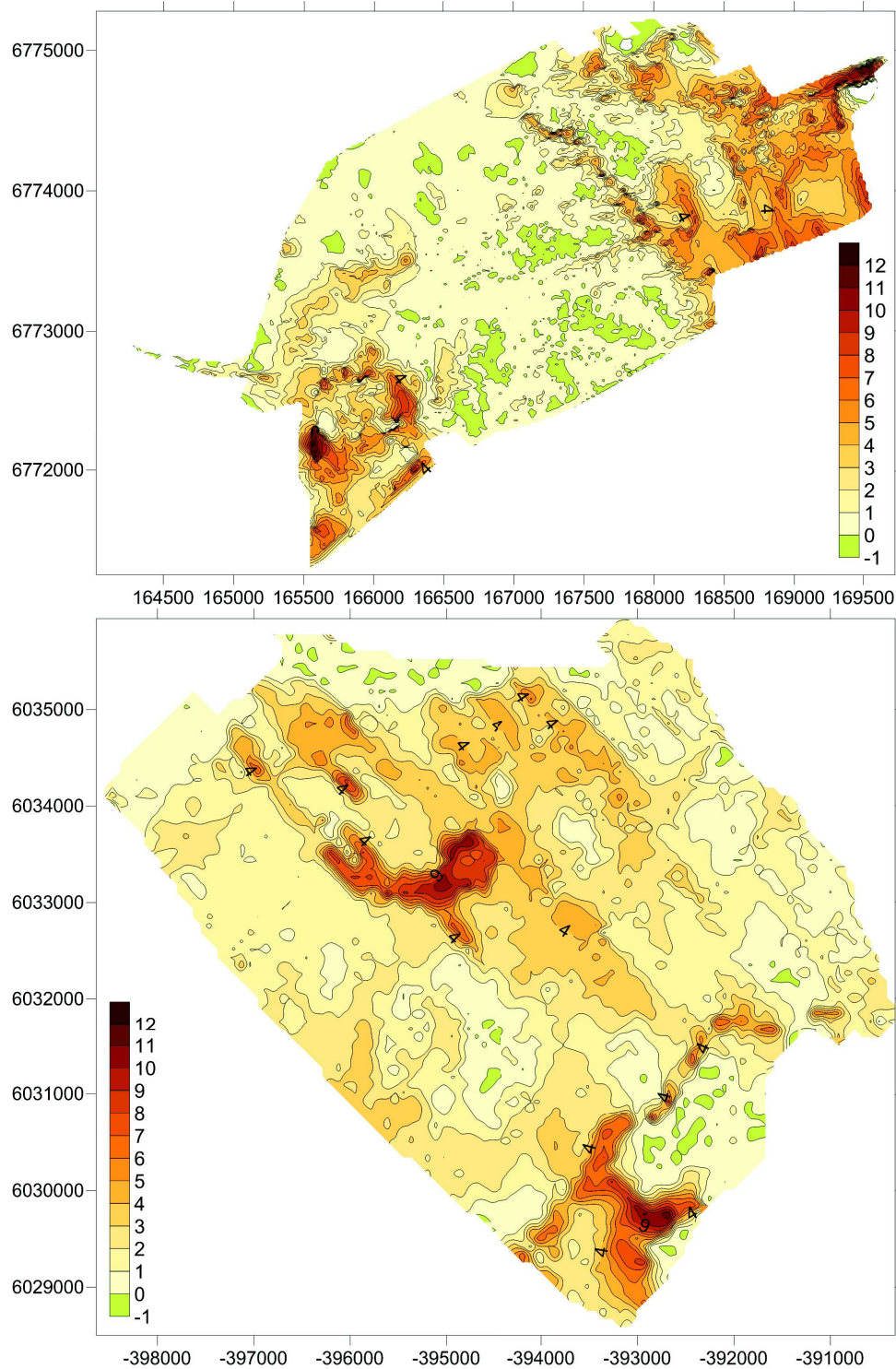
FIGURE 3.27 – Représentation des épaisseurs sédimentaires à Combrit-Île-Tudy (en haut) et Guidel (en bas) (valeurs en mètres).
