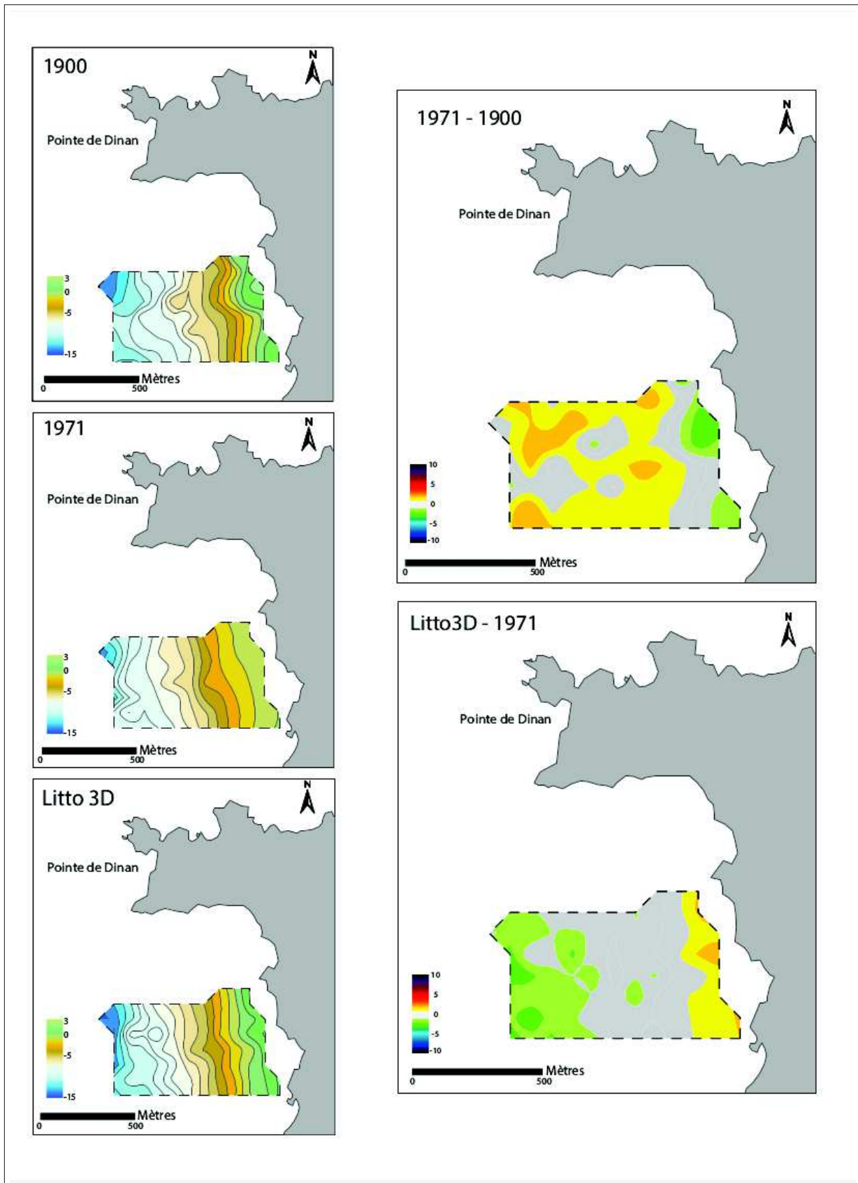
FIGURE 2.39 – Zone 5 nord : MNT et MNT différentiels (échelle de couleur : dégradé jaune-rouge = accrétion et dégradé vert-bleu = érosion)
