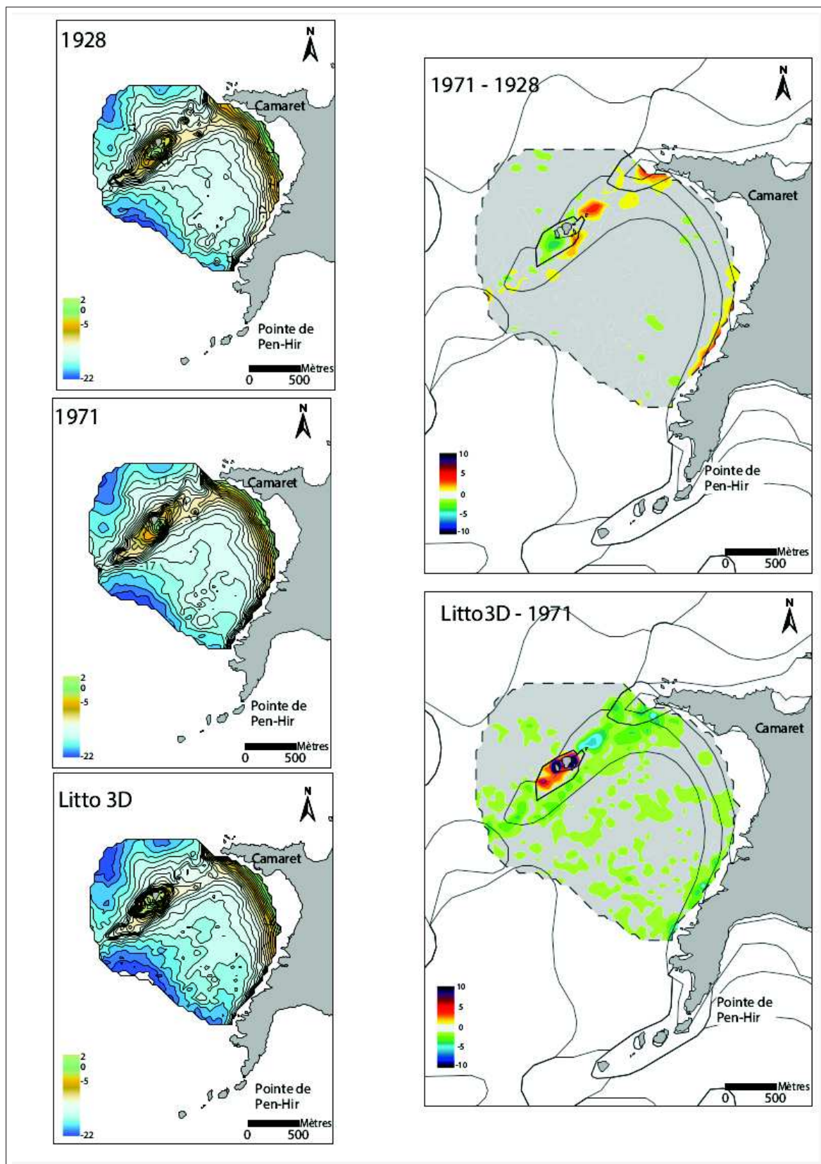
FIGURE 2.42 – Zone 6 : MNT et MNT différentiels (échelle de couleur : dégradé jaune-rouge = accrétion et dégradé vert-bleu = érosion)
