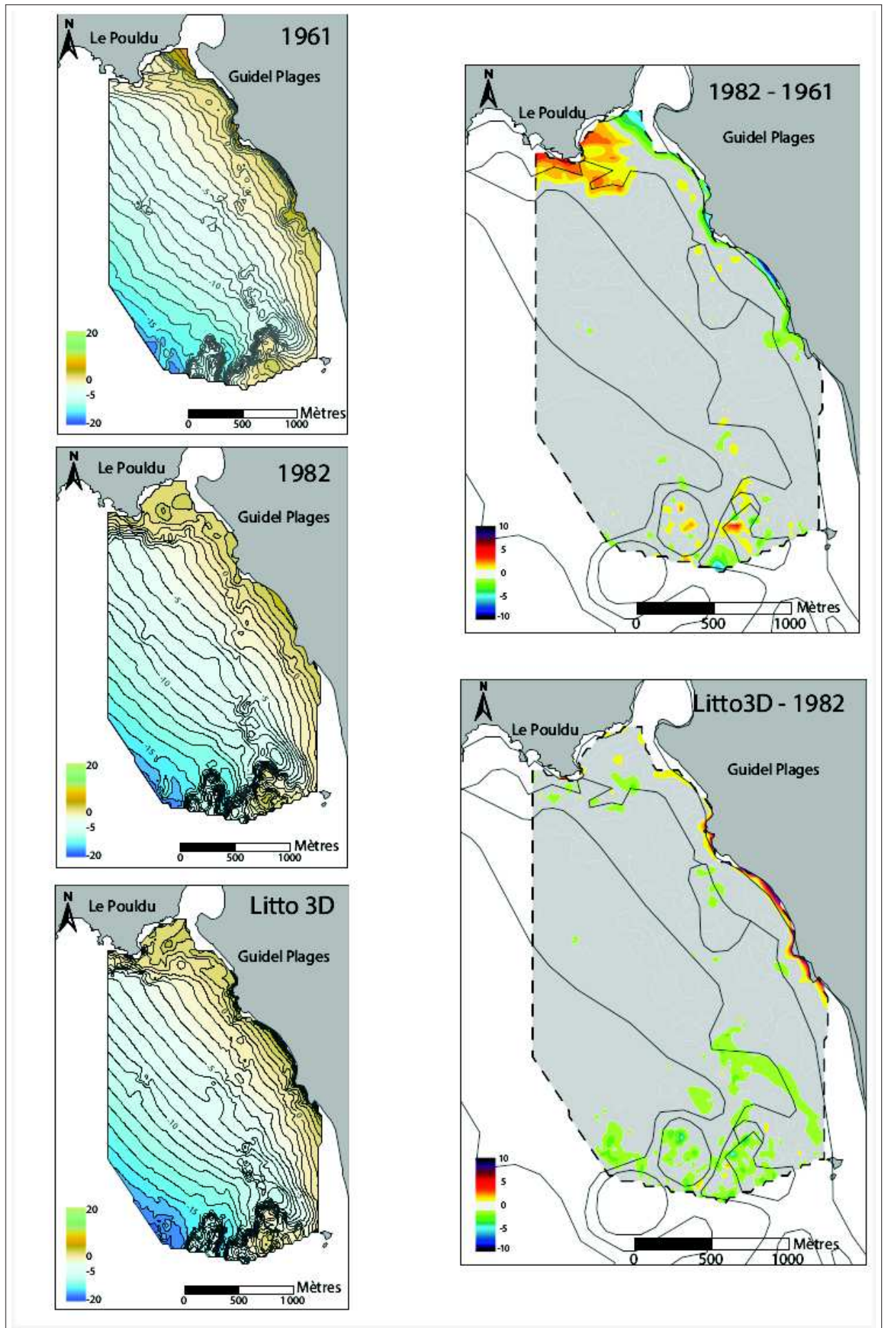
FIGURE 2.25 – Zone 1 : MNT et MNT différentiels (échelle de couleur : dégradé jaune-rouge = accrétion et dégradé vert-bleu = érosion)
