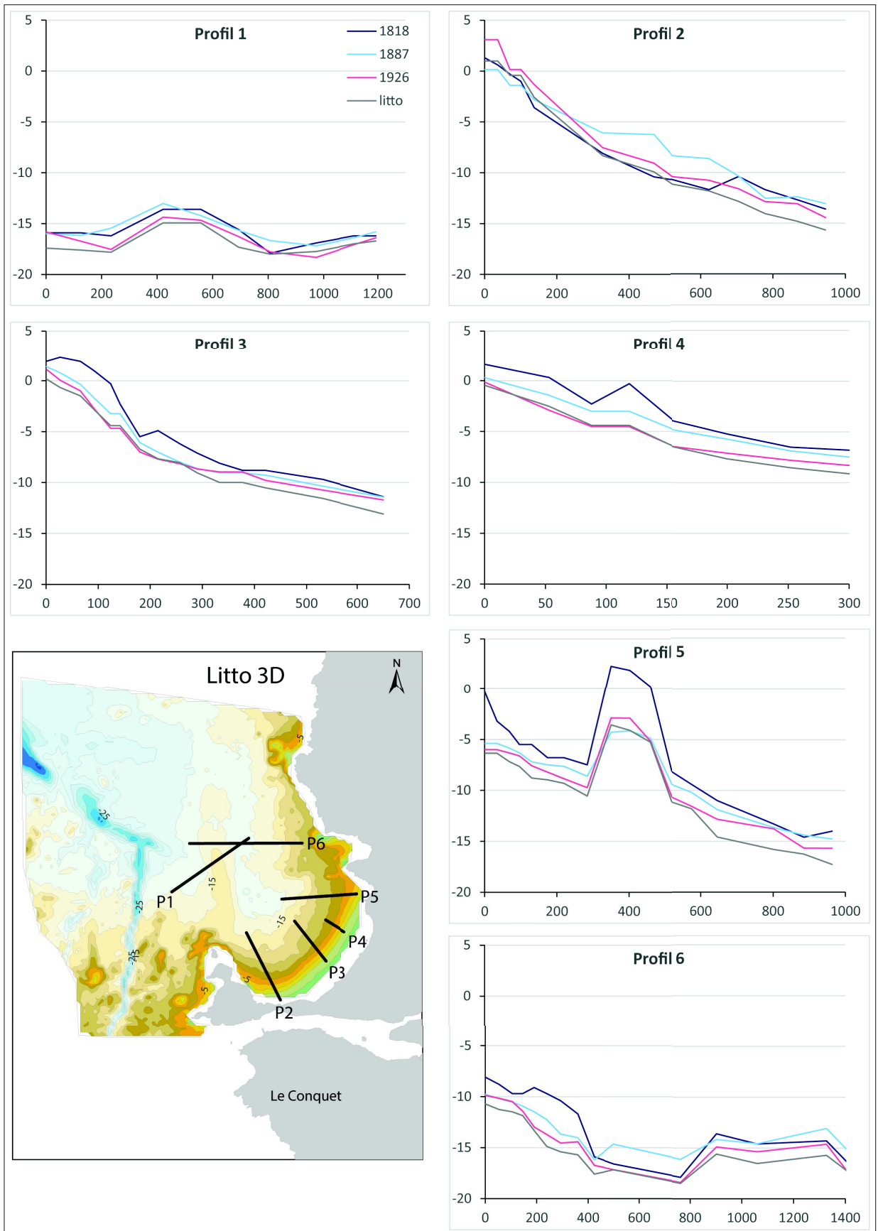
FIGURE 2.45 – Zone 7 : Profils
