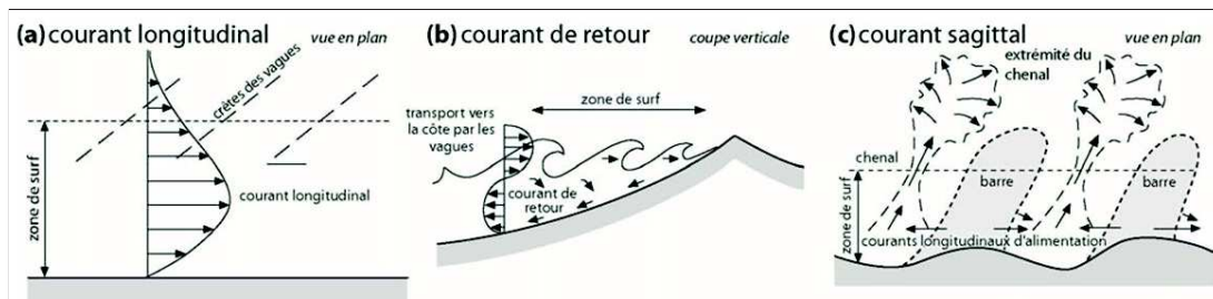
FIGURE 1.2 – Courants générés par les vagues : (a) courants longitudinaux induits par les vagues obliques à la côte, (b) courant de retour de fond, (c) courants sagittaux ((Dehouck, 2006) d'après Masselink and Hughes, 2003).
