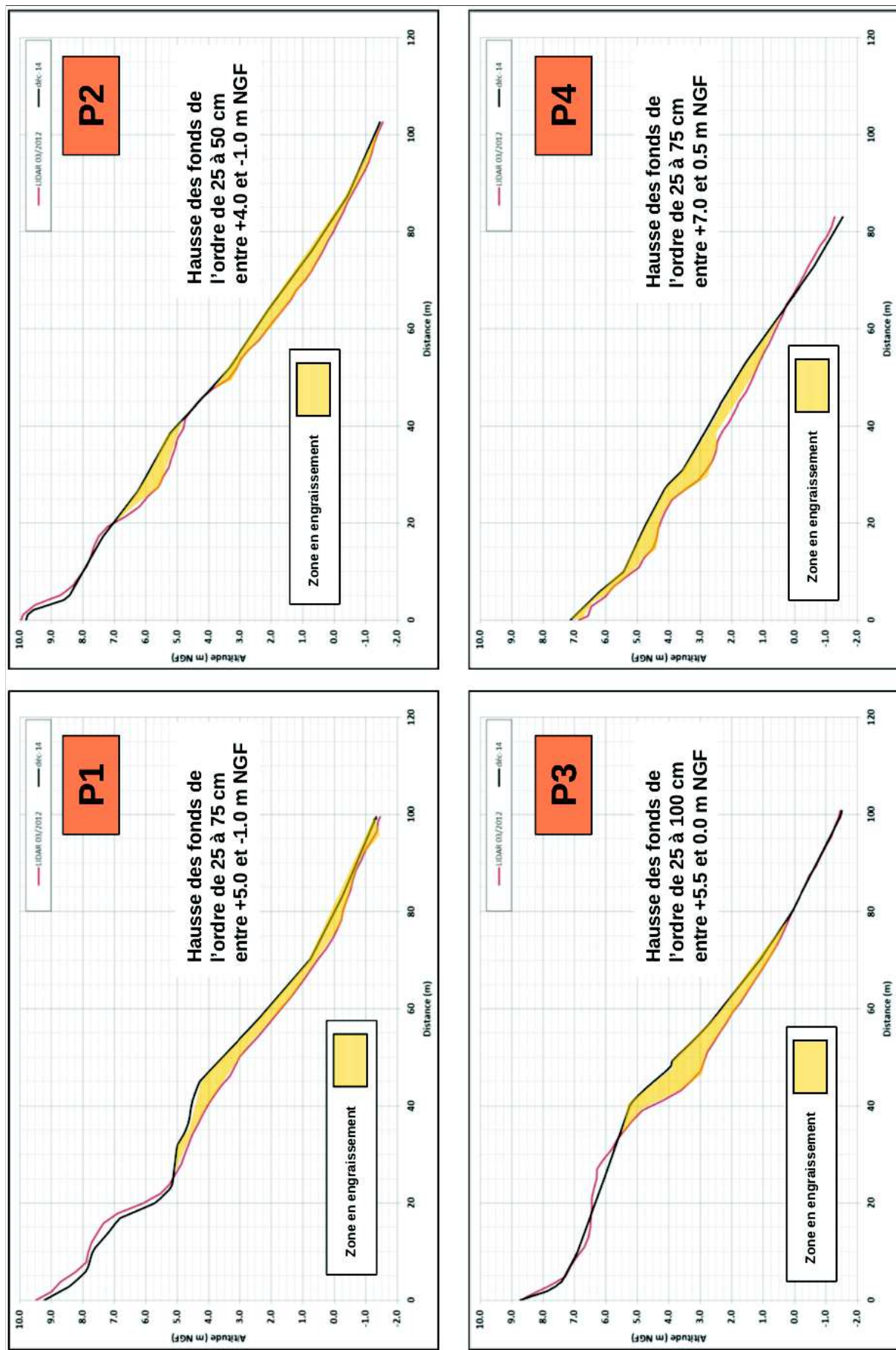
FIGURE 3.21 – Profils de plage dans le secteur de Penmorvan (Egis Eau, 2011).
