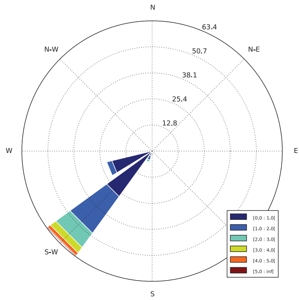
FIGURE .15 – Rose des houles au point 3899.
