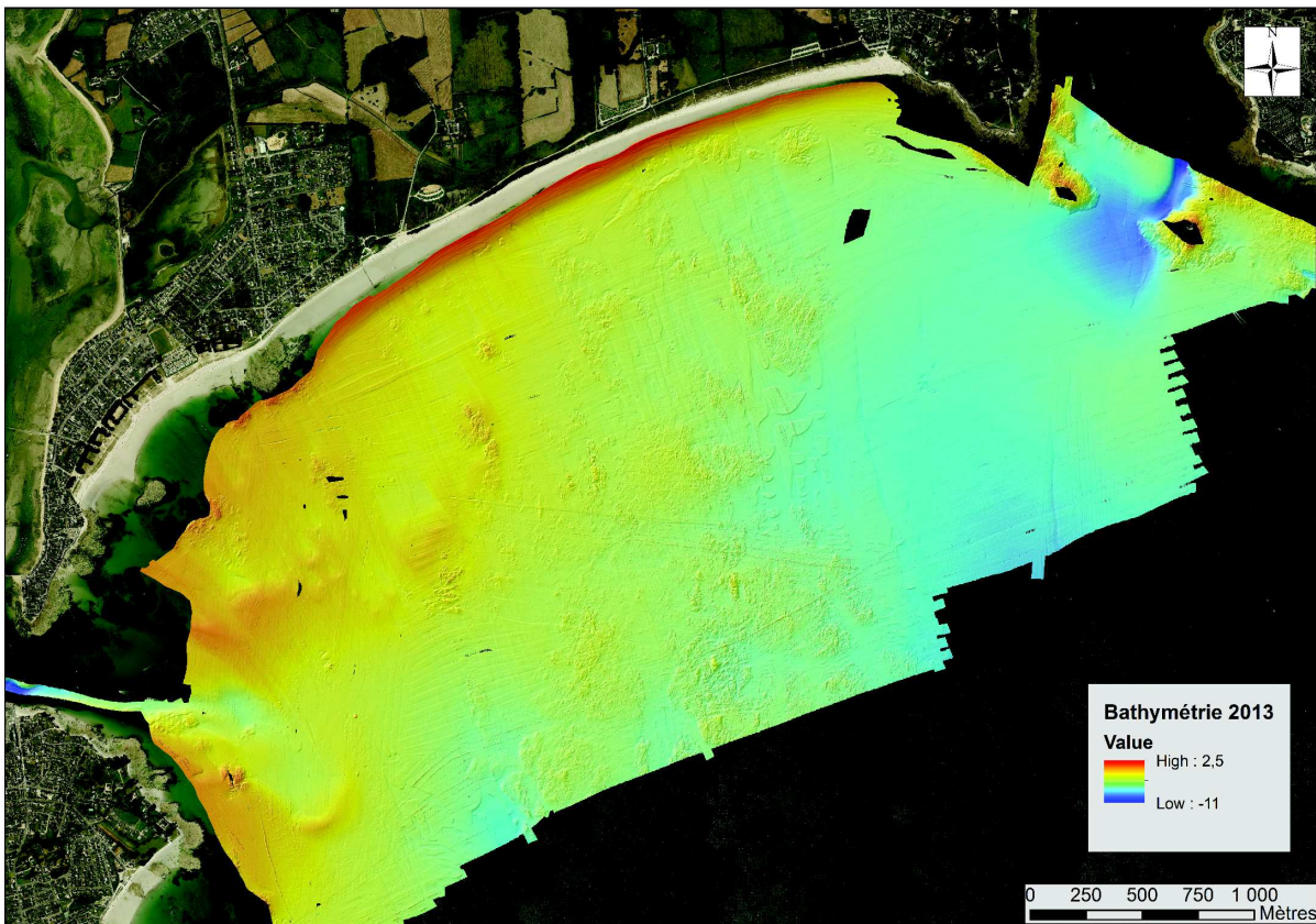
FIGURE 3.9 – Bathymétrie de 2013 sur le secteur de Combrit - Île-Tudy.
