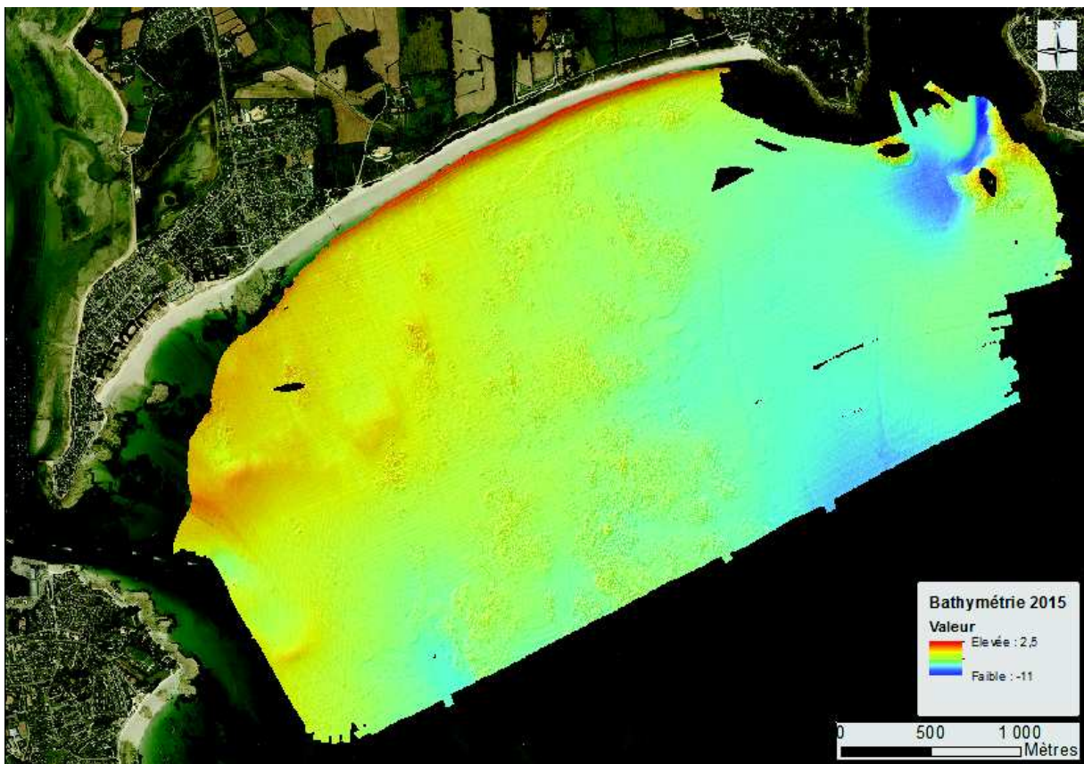
FIGURE 3.11 – Bathymétrie de 2015 sur le secteur de Combrit - Île-Tudy.
