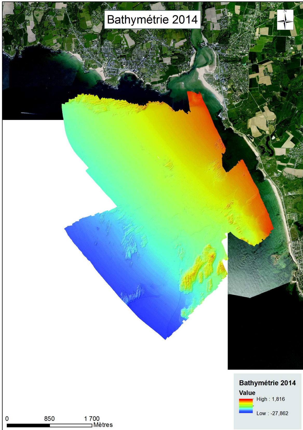
FIGURE 3.12 – Bathymétrie de 2014 sur le secteur de Guidel.
