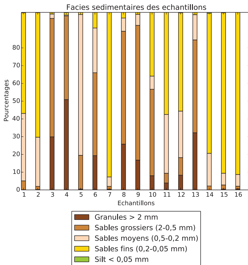
FIGURE 3.28 – Diagramme de la répartition de la granulométrie des échantillons analysés à Combrit - Île-Tudy (2015).
