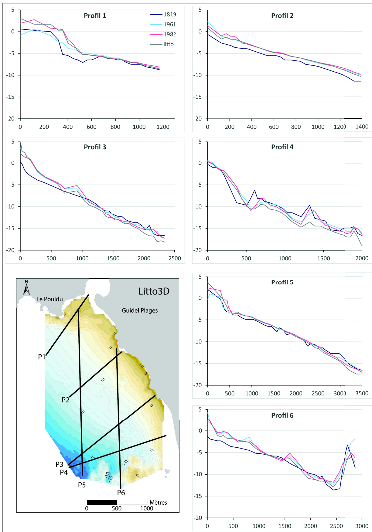
FIGURE 2.26 – Zone 1 : Profils
