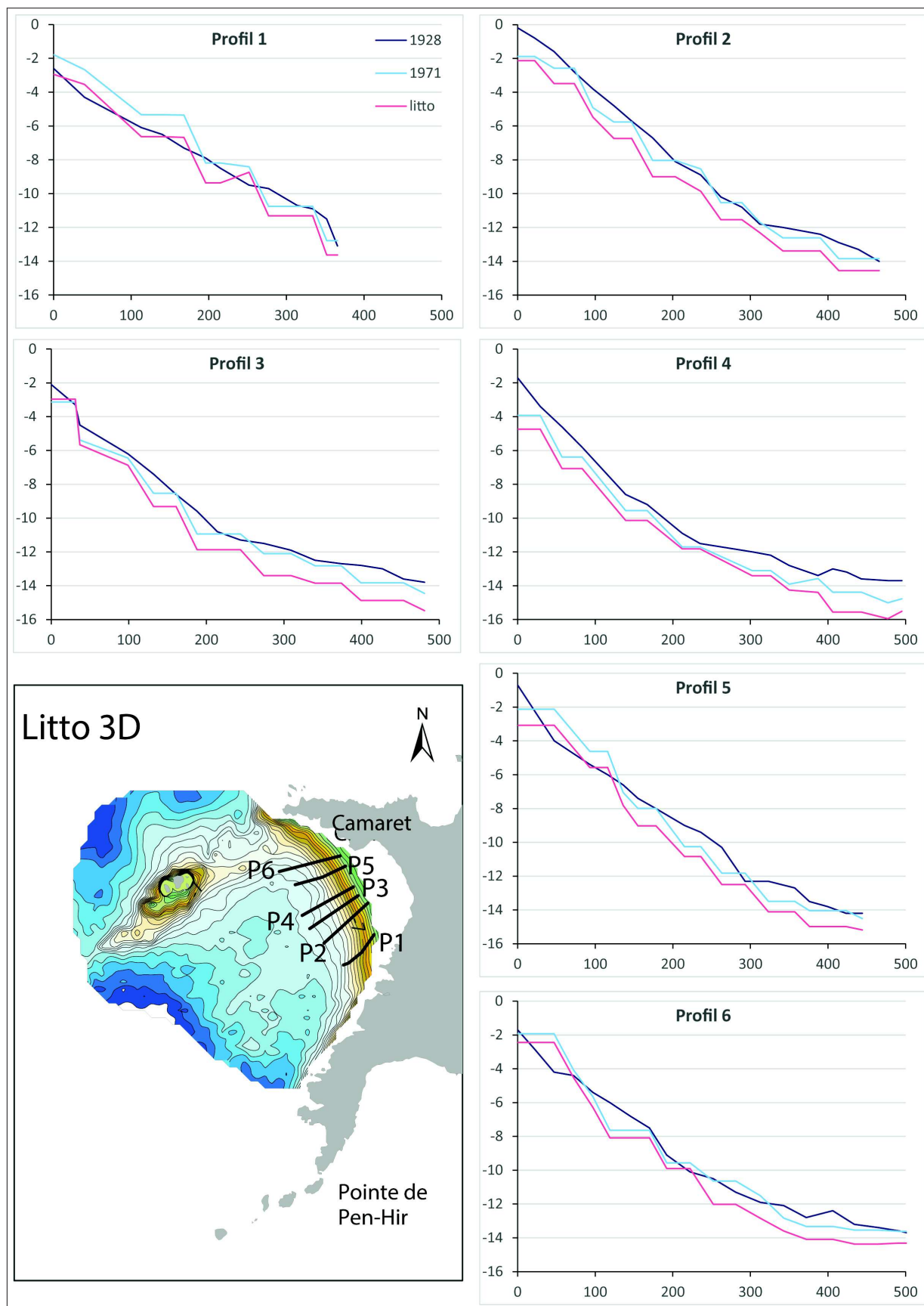
FIGURE 2.43 – Zone 6 : Profils
