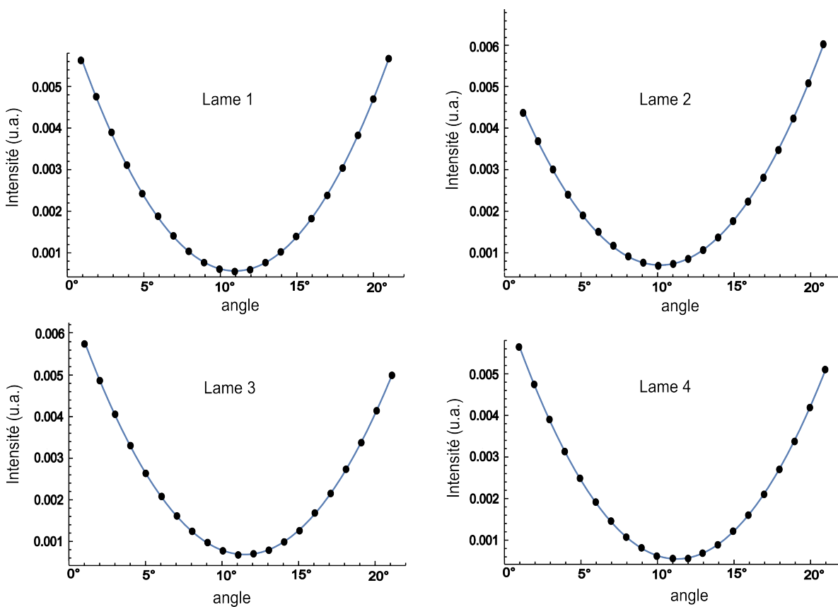
FIGURE II.17 – Interpolation polynomiale (en trait plein) pour les mesures d'intensité pour le polariseur et l'analyseur croisés.
