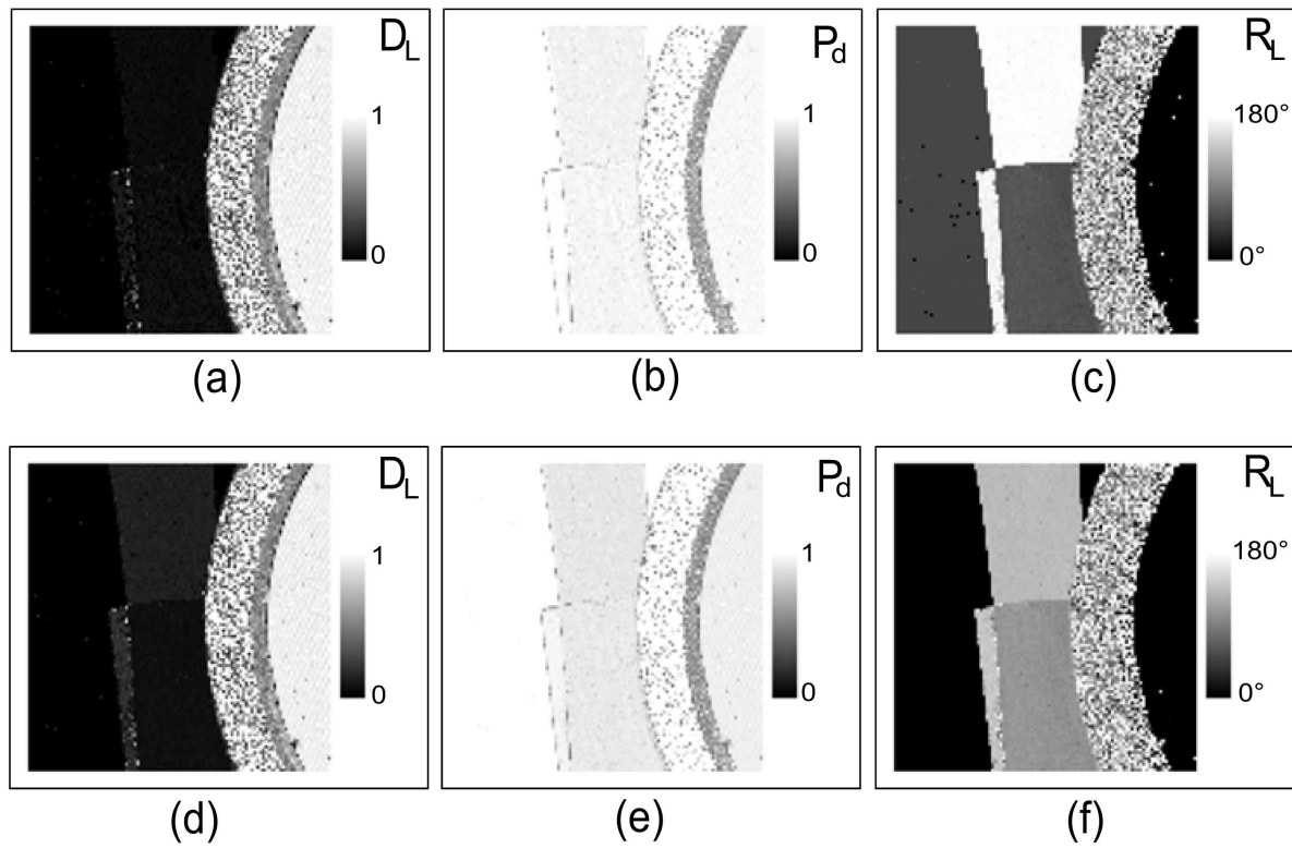
FIGURE II.34 – (a,b,c) Sans correction du cube. (d,e,f) Avec correction du cube. (a,d) D_L : Diatténuation linéaire, (b,e) P_d : Dépolarisation, (c,f) R_L : Retardance linéaire.
