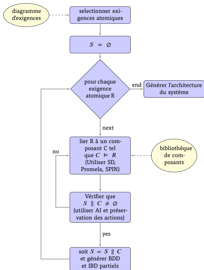
Figure 10.2 – Approche proposé pour la génération d'une architecture SBC à partir d'exigences SysML
