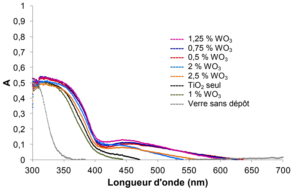
Figure 42: Superposition des spectres corrigés d'absorption des différents dépôts photocatalytiques \text{TiO}_2\text{-WO}_3 (IM-2)
