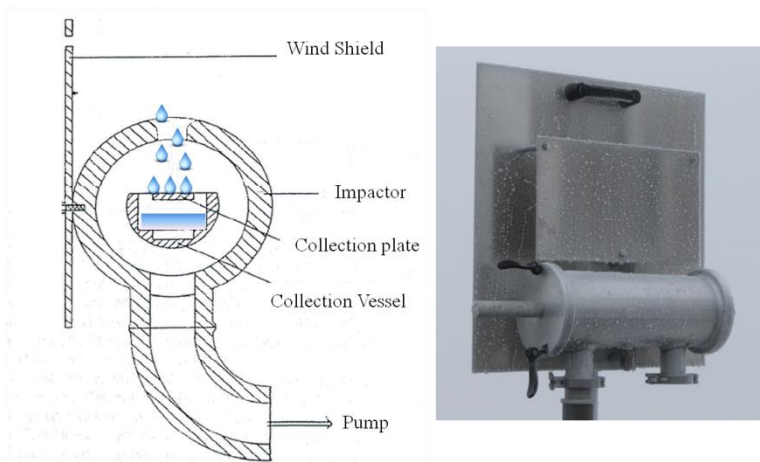
Figure 3: Impacteur à nuage.
