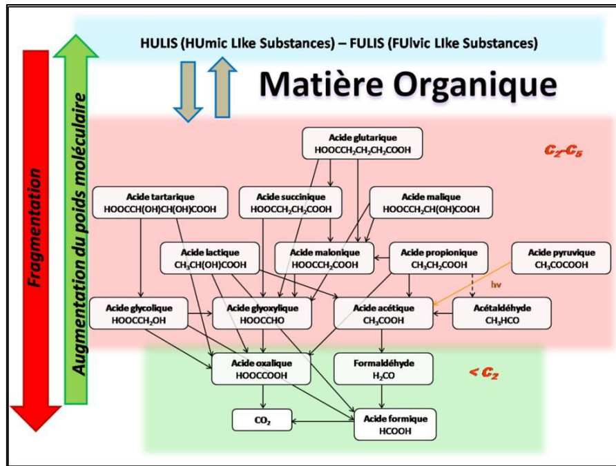
Figure 3: Représentation schématique des possibles voies de fragmentation (en acides carboxyliques et puis minéralisation en CO 2 ) et augmentation de la taille (jusqu'à la formation de substances type humiques, HULIS et FULIS) de la matière organique présente dans le nuage suite à la réaction avec les radicaux hydroxyles.
