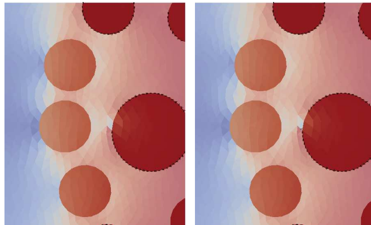
(a) Champ du gradient de température à t = 13.6\mu s .
