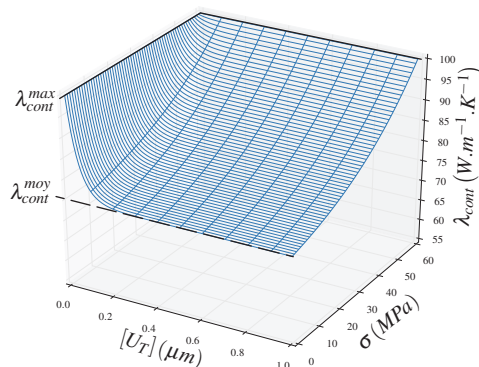
(a) Conductivité de contact à l'échelle macroscopique
