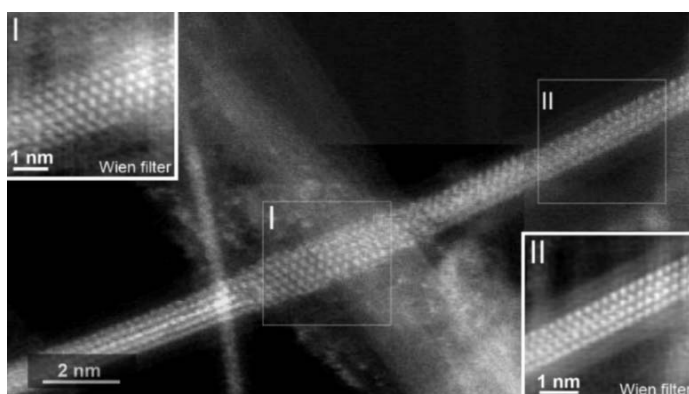
Fig. 2.2 - image ADF d'un nanocristal encapsulé de \text{NiI}_2 nanocristallins. Les encarts correspondent à l'application d'un filtre de Wien dans les zones I et II (programme "HRTEM Filter" développé par D. R. G. Mitchell ( http://www.dmscripting.com/hrtem_filter.html )).
