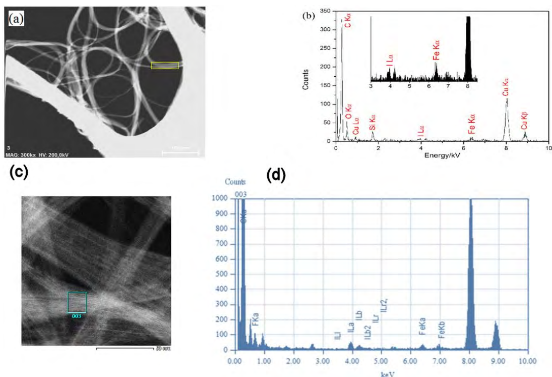
Figure 3.6 - (a) et (c) images STEM de FeI 2 @DWCNT-p et FeF 3 @DWCNT-p ; (b) et (d) spectres EDS correspondant aux zones encadrées en (a) et (c). L'encart présenté en (b) est un spectre agrandi de la région de 3 à 8,5 kV montrant les pics de I et Fe.
