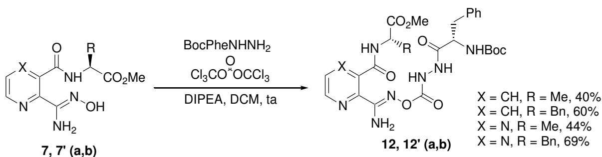
Schéma 12 Synthèse des peptidomimétiques 12 et 12'(a,b)
