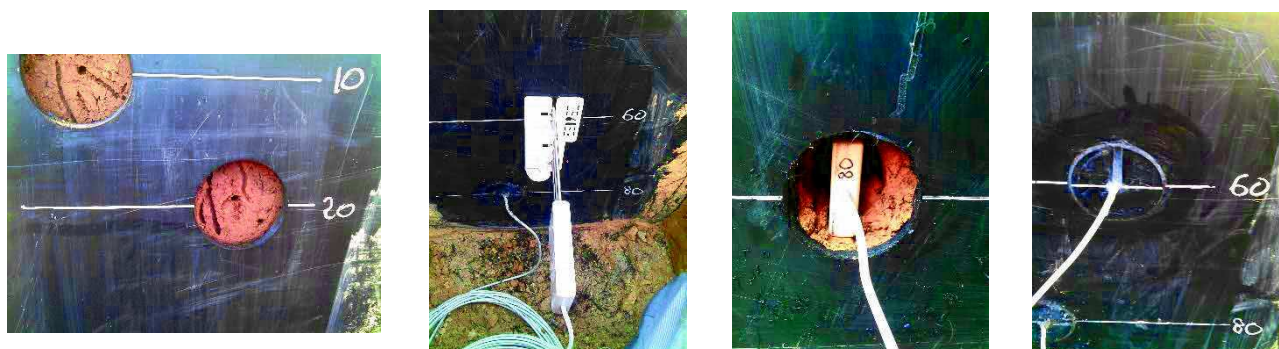
Image 2.15 : Mise en place des sondes TDR CS605 après la réalisation d'un trou dans la paroi de la Case 4 (01/08/2013).
