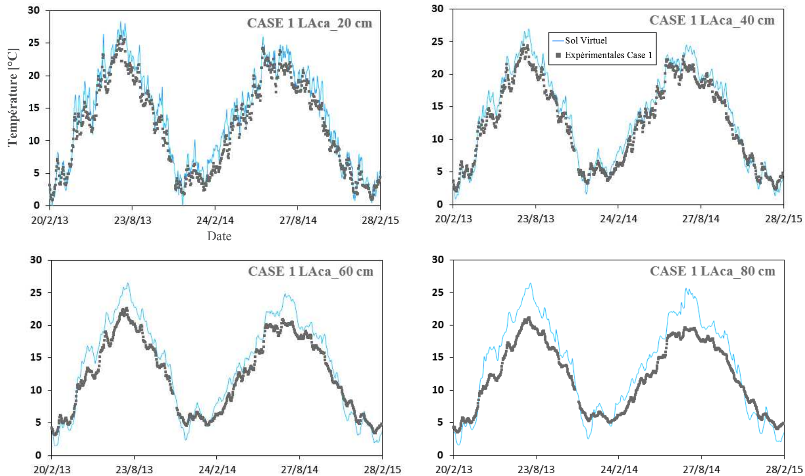
Figure II : Comparaison des données de température mesurées par les capteurs implantés à 20, 40, 60 et 80 cm sur la Case 1 (TEMOIN) et celles simulées par la plateforme Sol Virtuel.
