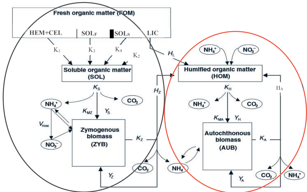
Figure 5.3 : Description de la transformation de la matière organique du sol par le modèle CANTIS.
