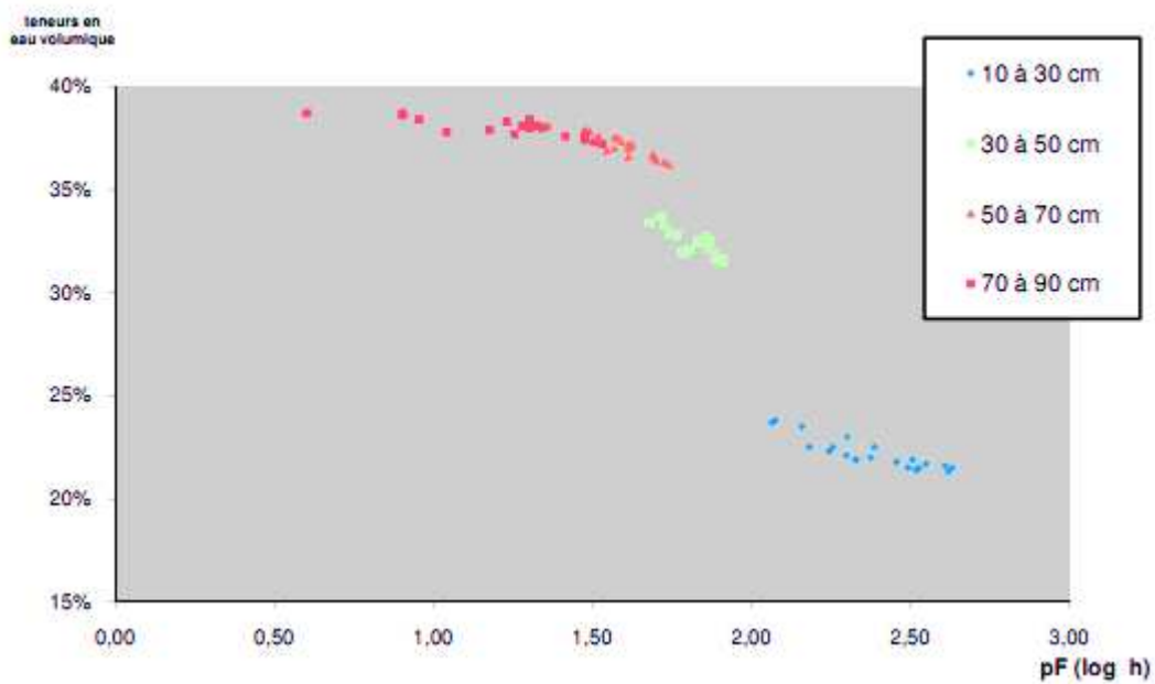
Figure II : Courbes de rétention en eau établies en 2010 à partir des dynamiques de données instrumentales observées in situ sur la Case 1.
