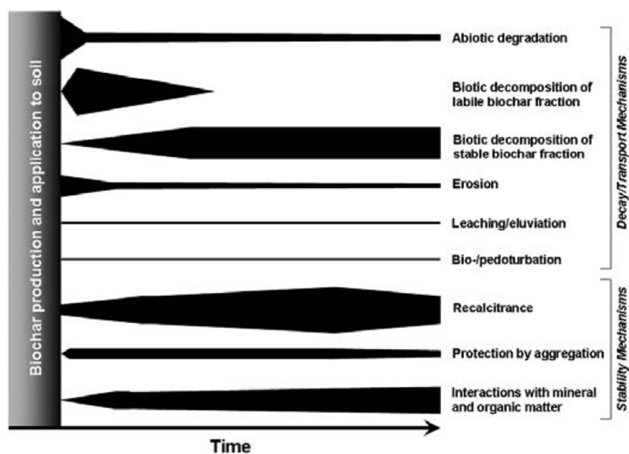
Figure I-2 : Facteurs qui influencent la stabilité et la décomposition ou transport du biochar dans les sols dans le temps. L'épaisseur des barres représente l'importance de chaque facteur dans le temps.
