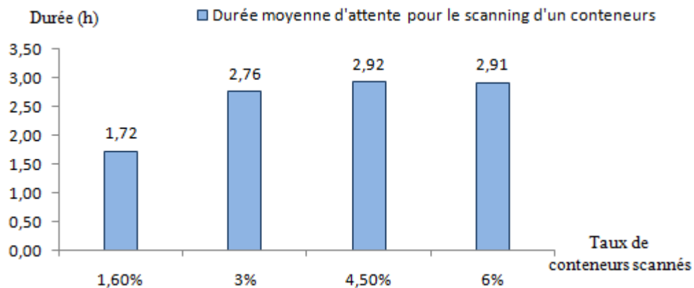
Figure III.21. Indicateur temps d'attente moyen dans la zone de stockage
