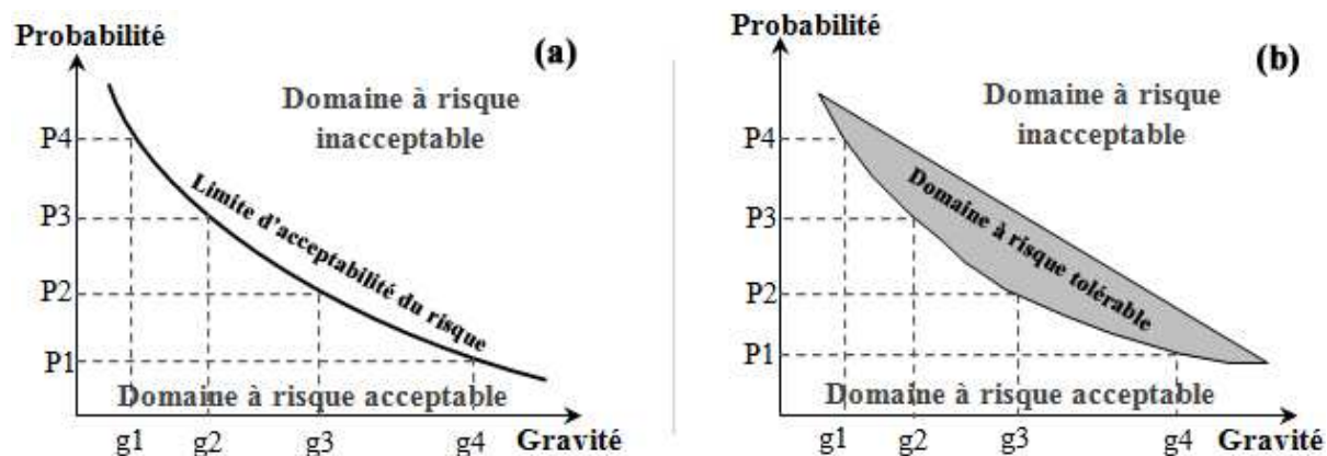
Figure II.3. (a) Diagramme de Farmer (b) domaine à risque tolérable
