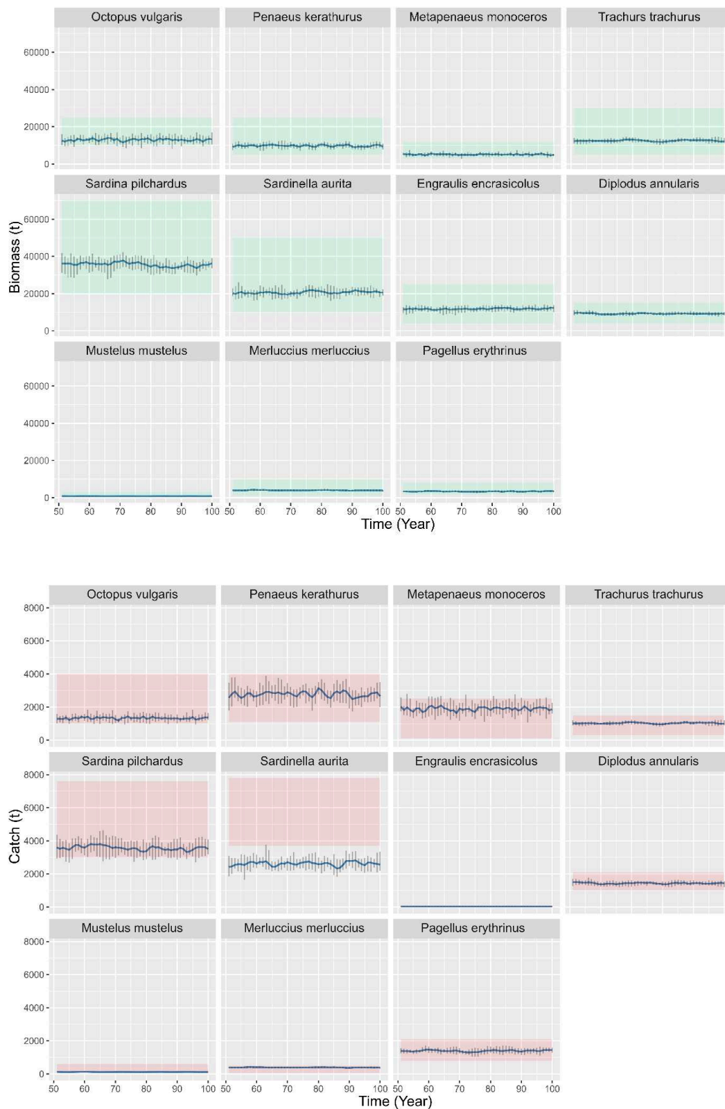
Figure 19 : Evolution moyenne des captures et des biomasses simulées des 11 espèces du modèle durant 50 années de simulation (lignes bleues), les barres d'erreur représentent l'intervalle de confiance obtenu à partir de 10 simulations. Les bandes colorées indiquent l'intervalle de référence (le maximum et le minimum des biomasses et des captures dans le golfe de Gabès sur la période 1998-2008)
