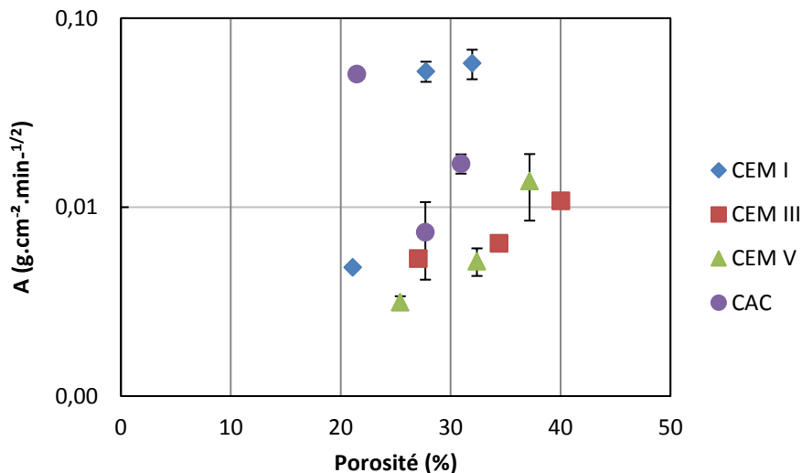
Figure IV.40 : coefficients de capillarité en fonction de la porosité avant soumission à l’essai de biocolonisation (échelle verticale logarithmique).
