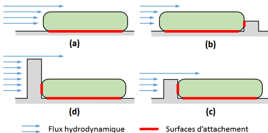
Figure I.15 : effet de micro-refuge des aspérités.
