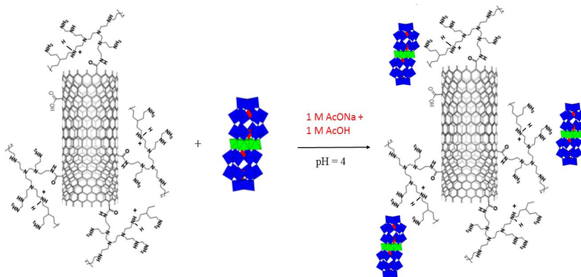
Figure 8. Schéma de synthèse de POM@SWCNT-PEI.
