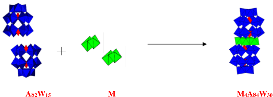
Figure 3. Schéma de synthèse d'un POM de type « sandwich » tétra-nucléaire.
