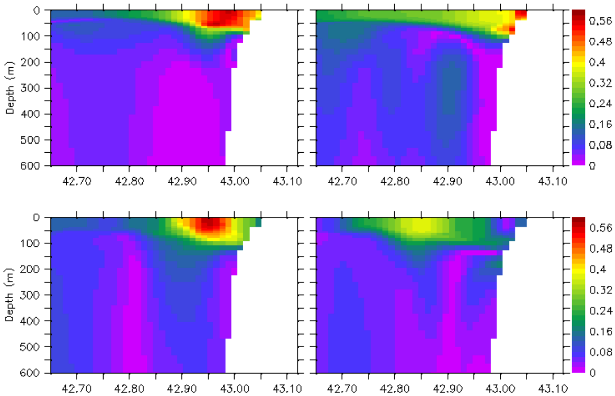
FIGURE 7.13 – Sections verticales, entre 0 et 600m, des courants ( \text{m}\cdot\text{s}^{-1} ) simulés le 17 Novembre 2013 (haut) et le 01 Décembre 2013 (bas) par GLAZUR64-2W de référence (gauche) et optimum (droite) à la sortie du zoom ( 5.8^\circ\text{E} ). Le positionnement exact des sections est présenté en figure 6.1.
