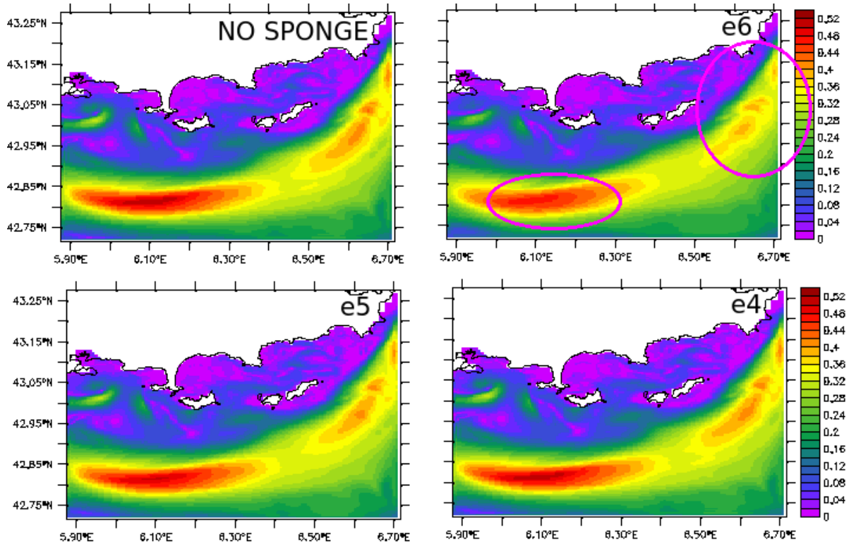
FIGURE D.8 – Courant de surface pour différentes valeurs de coefficient du bilaplacien : Gauche : A_{hm} = -4e^6 \text{ m}^4 \cdot \text{s}^{-1} ; Milieu : A_{hm} = -4e^5 \text{ m}^4 \cdot \text{s}^{-1} ; Droite : A_{hm} = -4e^4 \text{ m}^4 \cdot \text{s}^{-1}
