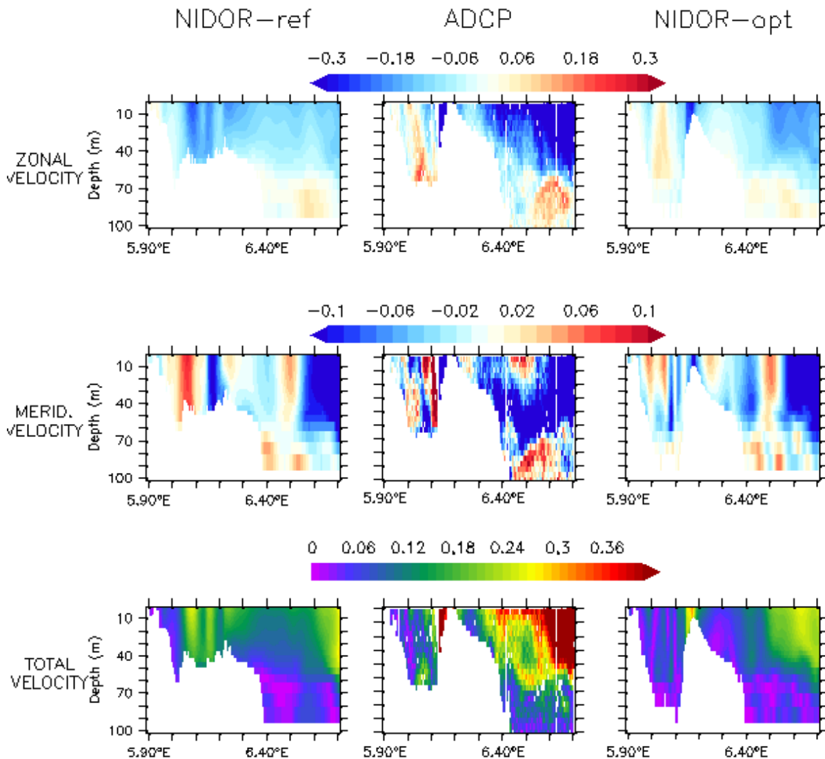
FIGURE 7.9 – Comparaison entre les champs de vitesse simulés et ceux observés par ADCP le 24 Octobre 2013 dans la baie (trajet identique à celui exploité en figure 4.3). Coupe verticale sur 140 m des composantes zonale et méridienne ainsi que du module ( \text{m}\cdot\text{s}^{-1} ) du courant le long du transect pour NIDOR192-référence (gauche), les données ADCP (milieu) et NIDOR192-optimum (droite).
