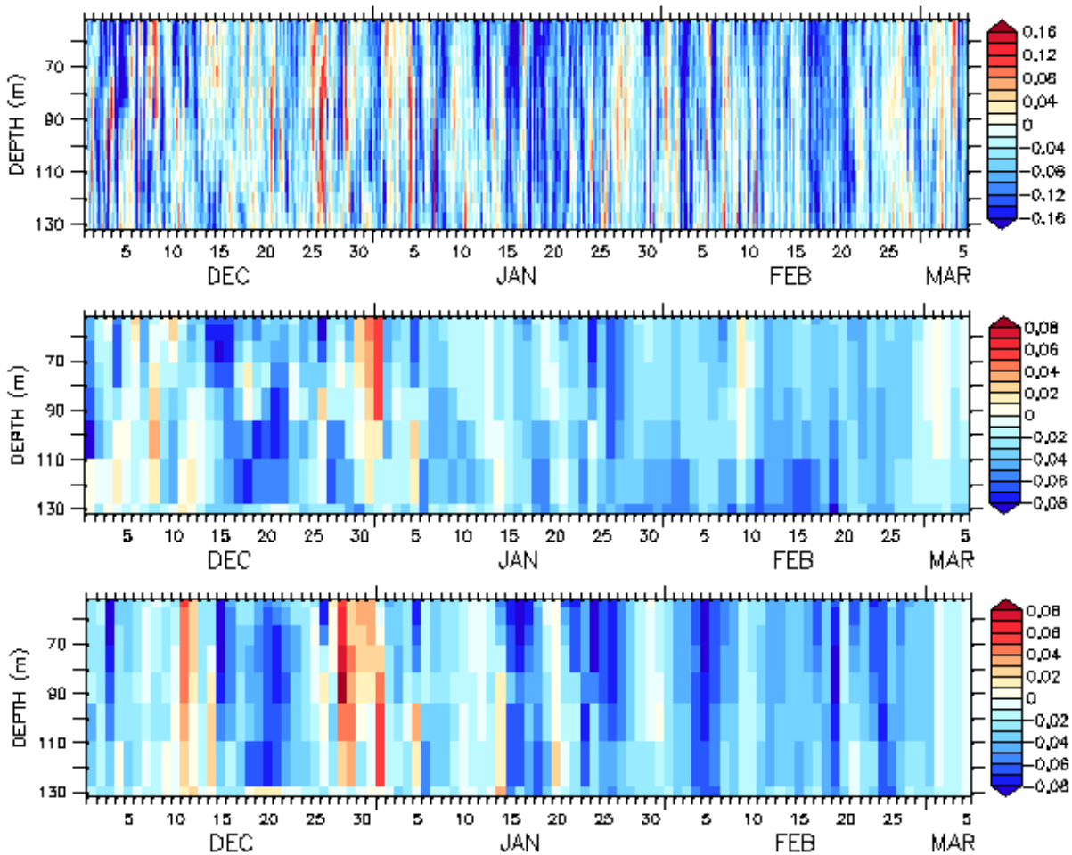
FIGURE 4.6 – Comparaison de l'évolution temporelle des profils verticaux de vitesses méridiennes ( \text{m}\cdot\text{s}^{-1} ) mesurés par ADCP au mouillage BOMBYX (haut) et simulés par GLAZUR64 (milieu) et NIDOR192 (bas).
