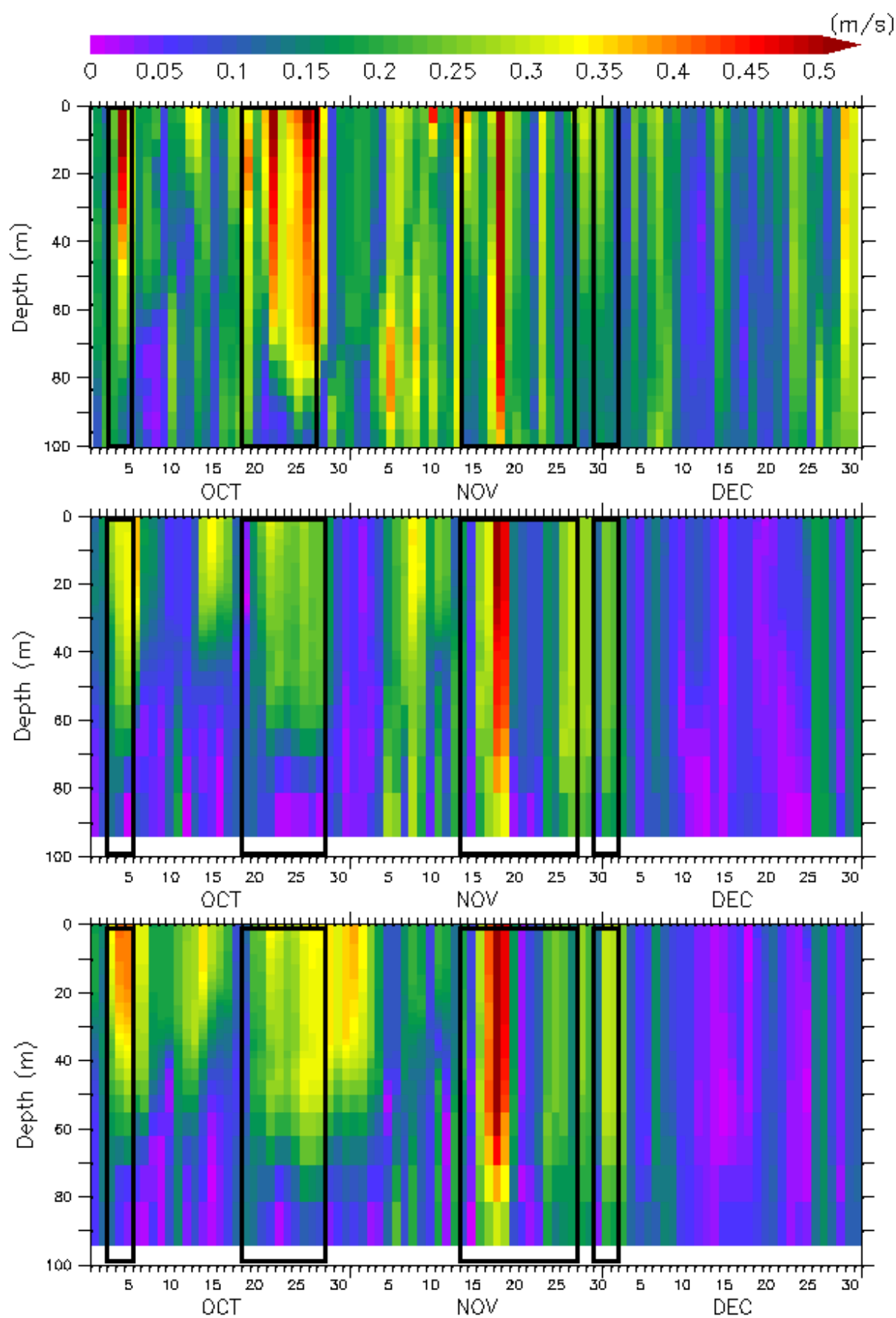
FIGURE 7.12 – Évolution temporelle du profil vertical de courant ( \text{m}\cdot\text{s}^{-1} ) au mouillage JULIO d'Octobre à Décembre 2013. Les observations ADCP sont présentées en haut et les simulations de GLAZUR64-2W de référence au milieu et optimum en bas. Les encadrés noirs superposés représentent les événements d'intrusions étudiés.
