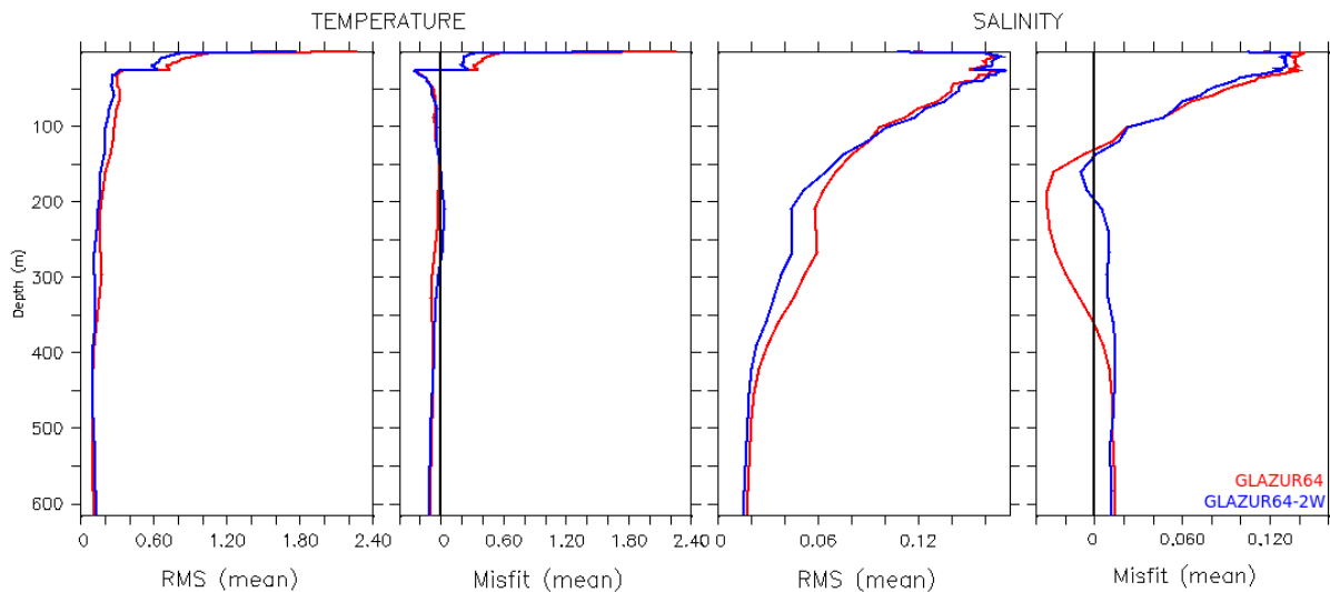
FIGURE 6.4 – Profils verticaux, entre 0 et 600 m, moyens des RMS et écarts entre les simulations et les observations glider, GLAZUR64 (rouge), GLAZUR64-2W (bleu), pour la température ( ^{\circ}\text{C} ) et la salinité (PSU).
