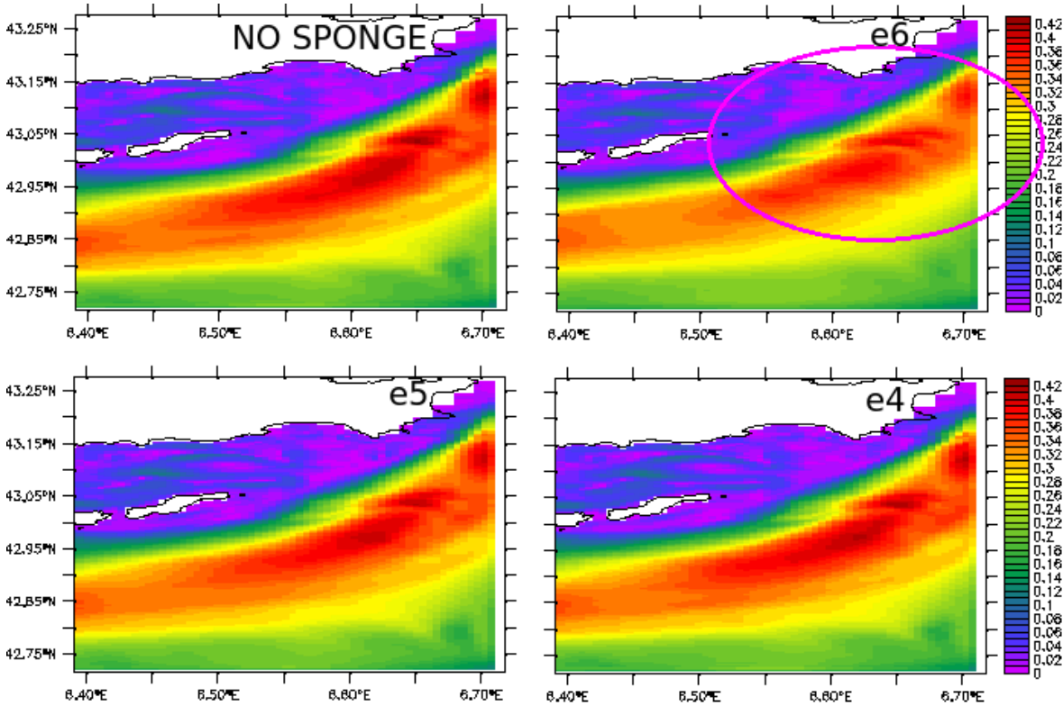
FIGURE D.7 – Courant de surface proche de la frontière Est de NIDOR. Gauche : A_{hm} = -4e^6 m^4.s^{-1} ; Milieu : A_{hm} = -4e^5 m^4.s^{-1} ; Droite : A_{hm} = -4e^4 m^4.s^{-1}
