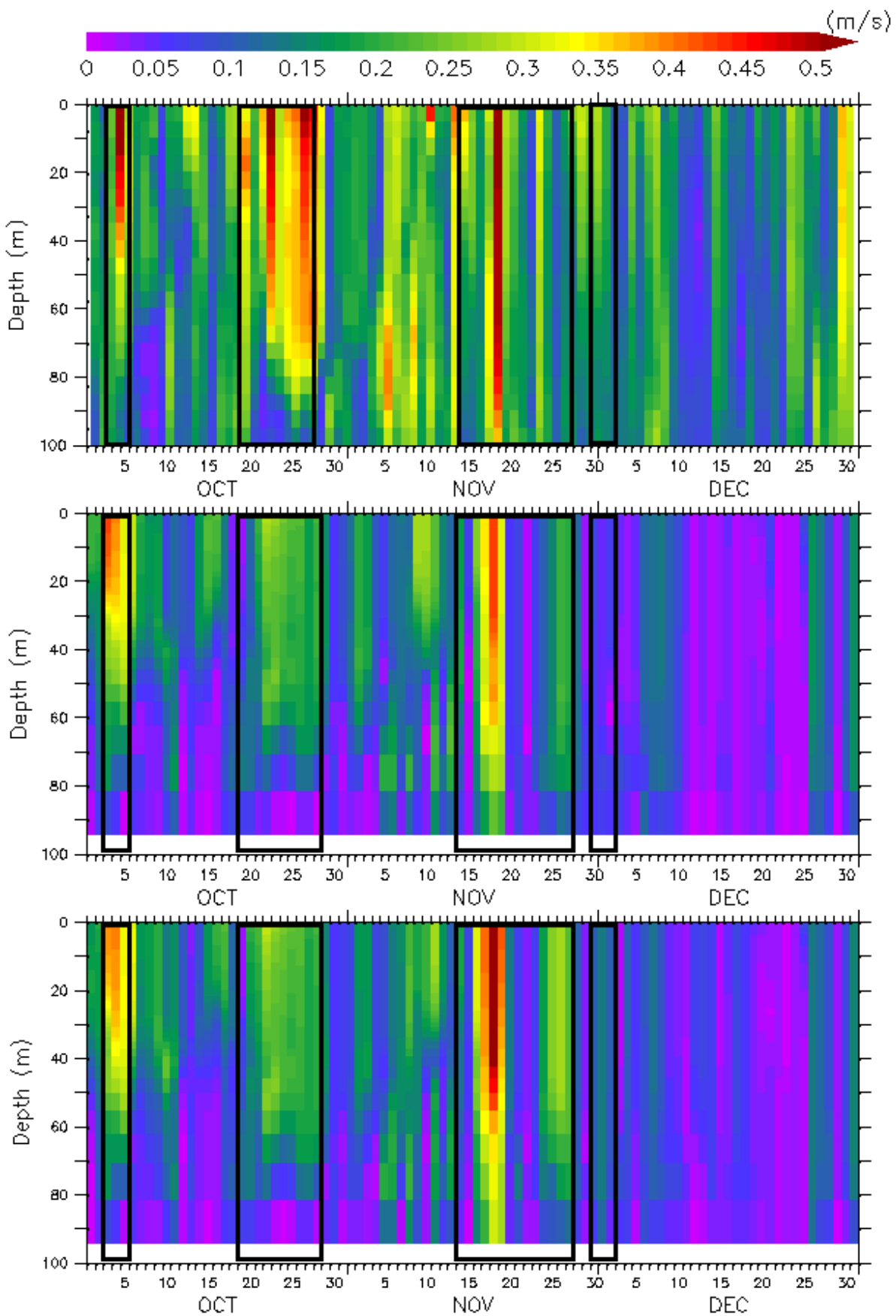
FIGURE 6.5 – Évolution temporelle du profil vertical de courant ( \text{m}\cdot\text{s}^{-1} ) au mouillage JULIO d’Octobre à Décembre 2013. Les observations ADCP sont présentées en haut et les simulations de GLAZUR64 au milieu et GLAZUR64-2W en bas. Les encadrés noirs superposés représentent les événements d’intrusions étudiés.
