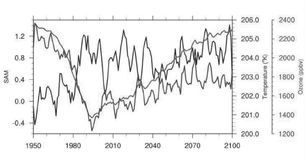
FIGURE 3.23: Série temporelle de l'indice SAM normalisé (unité = 1 écart type) pour l'ensemble HIST (1950-2005) et l'ensemble RCP8.5 (2006-2100) pour la saison DJF. Les courbes bleue et rouge correspondent aux indices de température et concentration d'ozone calculés sur la couche 30-100 hPa au niveau du pôle sud (60°S - 90°S) pour la saison SON.
