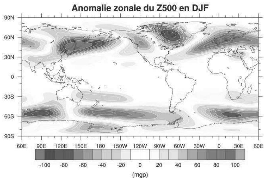
FIGURE 1.10: Champ d’écart à la moyenne zonale du géopotentiel à 500 hPa (en mgp) en DJF calculé dans la ré-analyse NCEP sur la période 1948-2015.
