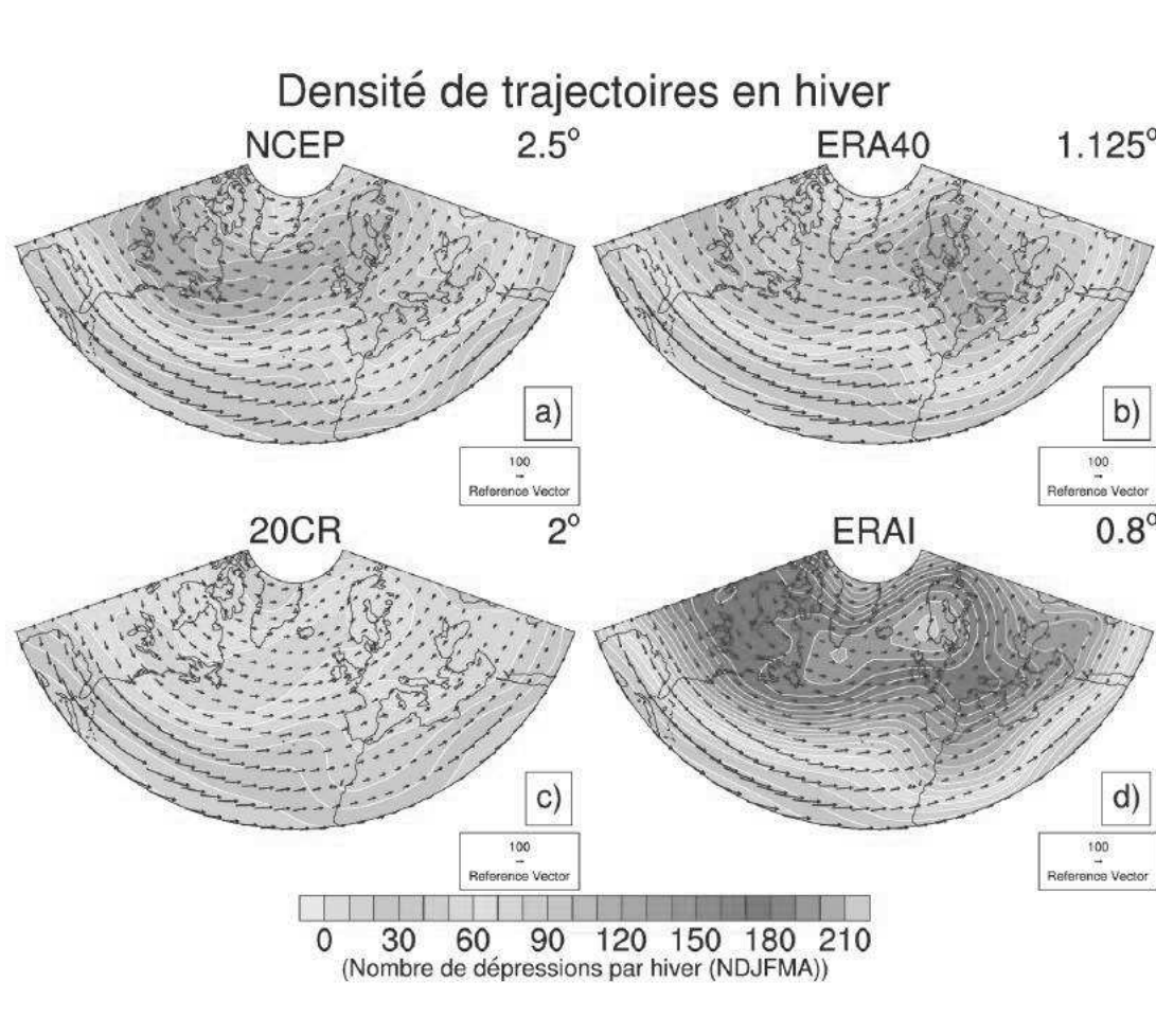
FIGURE 5.1: Densité de trajectoires des dépressions dans les 4 ré-analyses atmosphérique : (a) NCEP, (b) ERA40, (c) 20CR et (d) ERAI pour l’hiver étendu NDJFMA et sur leur période commune 1979-2001. Les vecteurs indiquent la vitesse et la direction moyenne de déplacement. La résolution de chaque ré-analyse est indiquée à la droite de chaque figure.
