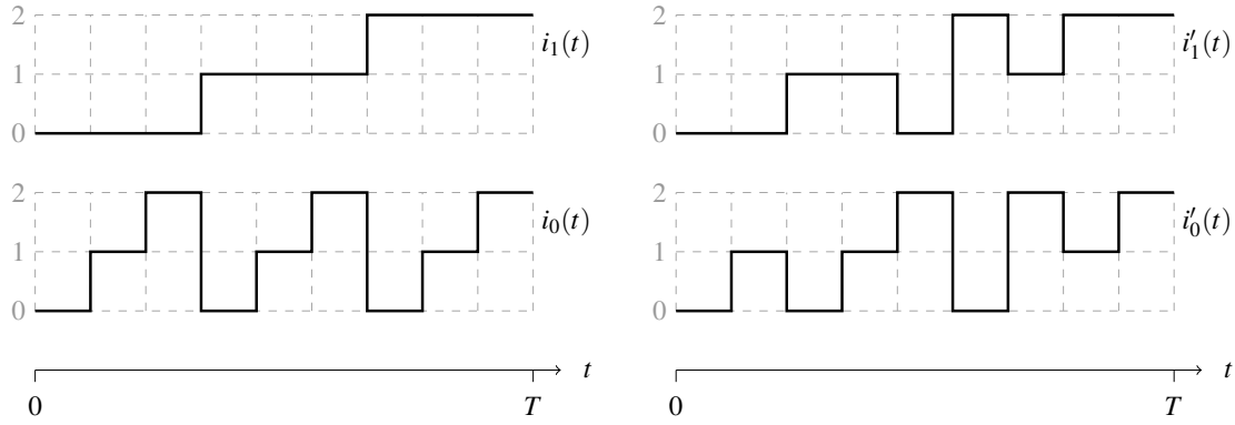
FIGURE 4.2 – Exemples d’ordonnement des vecteurs de sélection avec m = 2 . Les vecteurs [i'_0(t), i'_1(t)] (à droite) sont mieux ordonnés que les vecteur [i_0(t), i_1(t)] définis par l’équation 4.8 (à gauche)
