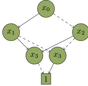
Figure 2.7: A BDD encoding of x_0 \cdot (x_1 \leftrightarrow \neg x_3) \vee \neg x_0 \cdot (x_2 \leftrightarrow \neg x_3)
