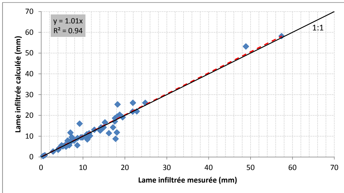
Figure 13. 10. Relation entre lames d'eau infiltrées mesurées et calculées sur Cult (champ). Droite de régression (en pointillé rouge) et première bissectrice (en noir).
