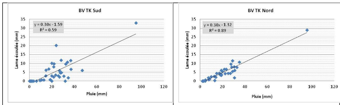
Figure 12. 10. Relation entre pluie et lame écoulée sur les bassins du site sédimentaire sur la période 2011-2012.
