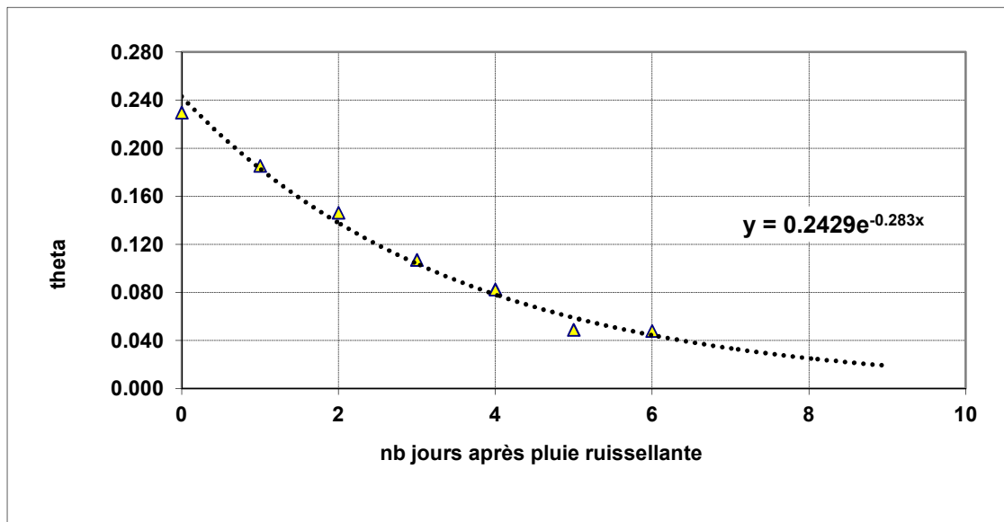
Figure 13. 1. Décroissance de la teneur en eau en 2012 au cours des jours sans pluies sur l'état de surface BIOL (site cristallin).
