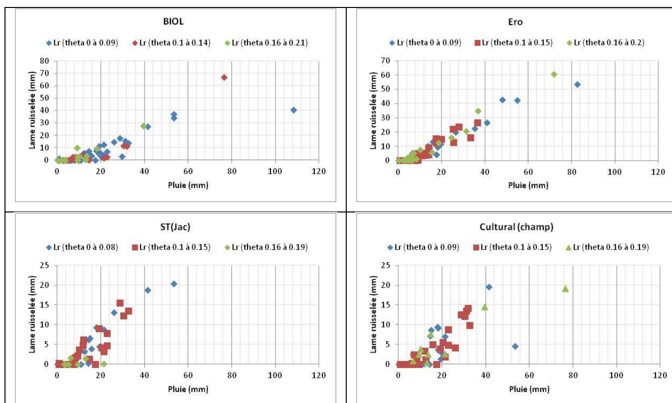
Figure 11. 9. Effet de l'humidité initiale sur le ruissellement par état de surface (site cristallin).
