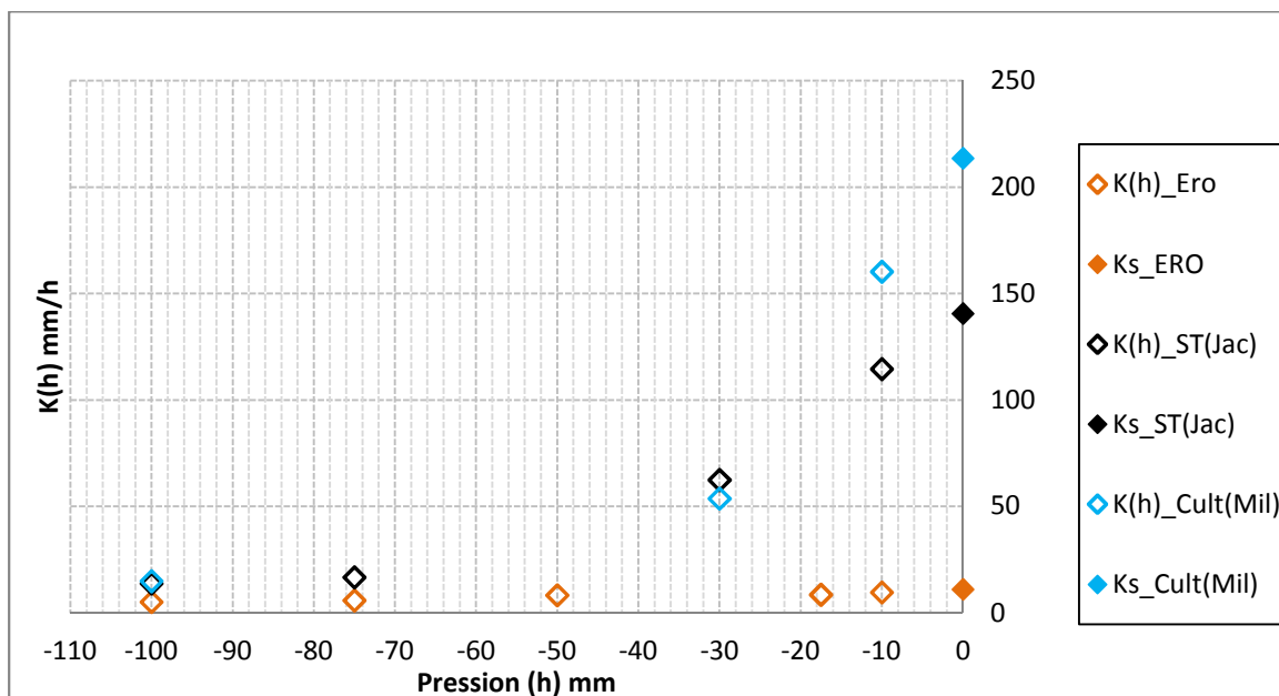
Figure 10. 4. Relation K(h) issue de la méthode MP avec petit disque ( r = 40 mm). Le nombre de répétitions est de 3 pour chaque état de surface
