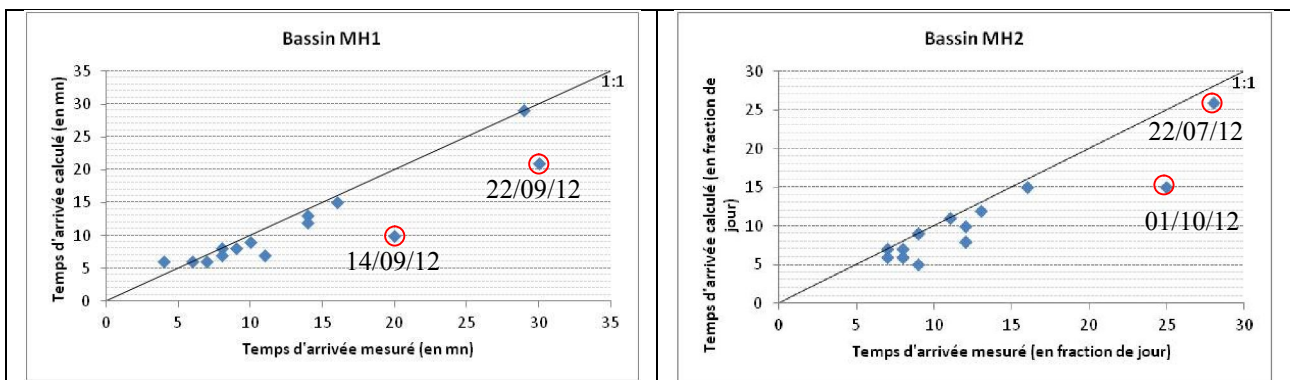
Figure 14. 3. Temps d'arrivée mesuré et calculé de l'écoulement à l'exutoire des bassins MH1 (à gauche) et MH2 (à droite) en 2012.
