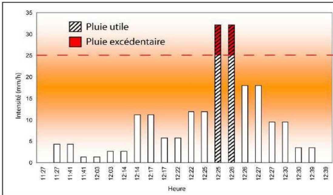
Figure 13. 12. Principe de détermination des pluies utile et excédentaire. Extrait de Le Breton (2012).
