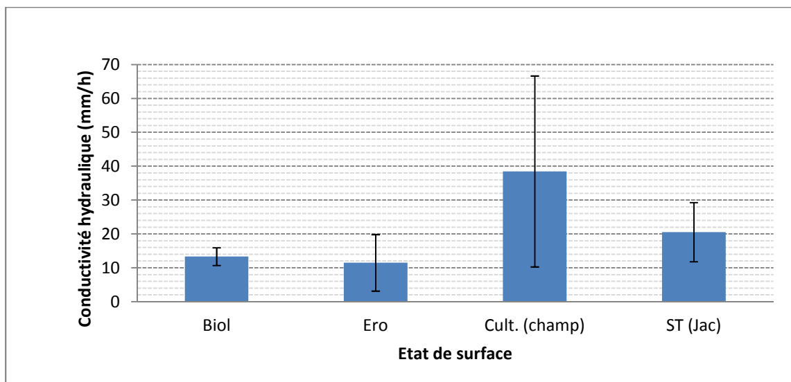
Figure 10. 9. Conductivité hydraulique en surface (0-3 cm) des états de surface du site cristallin.
