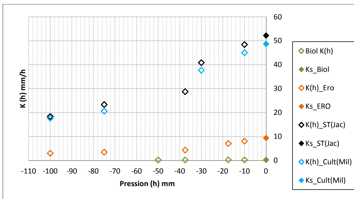
Figure 10. 3. Relation K(h) issue de la méthode MP grand disque ( r = 125 mm).
