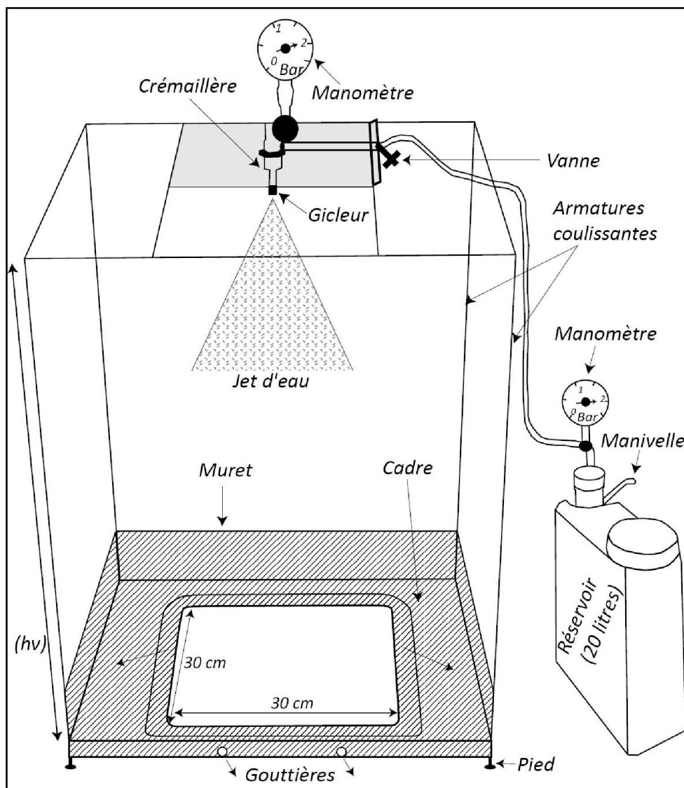
Figure 7.1. Schéma du saturomètre
