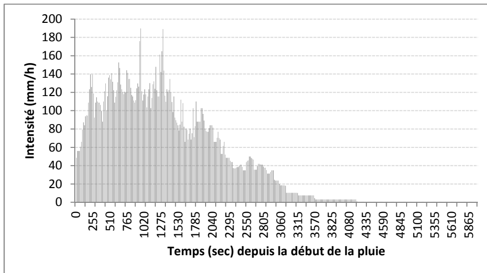
Figure 2.5. Hyetogramme de la pluie du 25/07/2011 (Site de Melé Haoussa)
