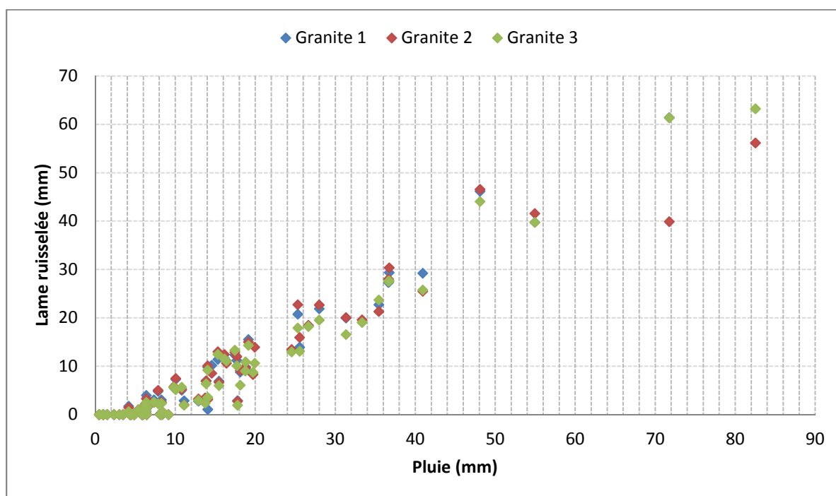
Figure 11. 2. Exemple d'homogénéité des lames ruisselées sur les différentes parcelles d'un même état de surface (ici parcelles de Granite).
