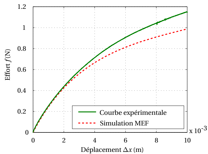
FIGURE 4.30 – Caractéristique effort/déplacement pour la solution BM.
