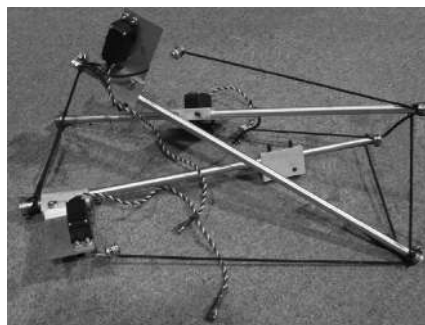
FIGURE 1.10 – Robot mobile basé sur une tensegrité T3 proposé dans [Paul 2006]. Les longueurs des trois câbles élastiques latéraux sont contrôlés par des actionneurs.
