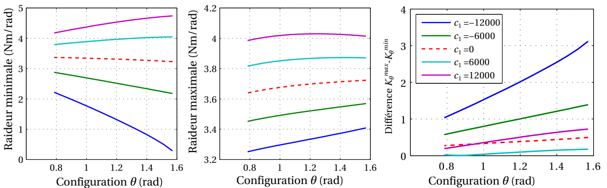
FIGURE 4.12 – Influence de c_1 sur K_{\theta}^{min} et K_{\theta}^{max} pour c_2 constant et R_L = 1 .
