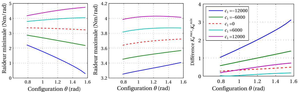
FIGURE 4.12 – Influence de c_1 sur K_{\theta}^{min} et K_{\theta}^{max} pour c_2 constant et R_L = 1 .
