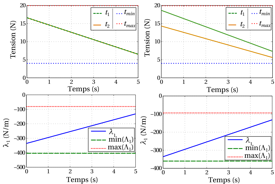
FIGURE 5.7 – Simulation d'une variation linéaire de raideur entre K_\theta = 0.5 et 1 Nm/rad sur 5 s pour \theta^* = \pi/2 rad à gauche, et \theta^* = 1.31 rad à droite.
