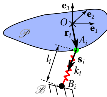
FIGURE C.1 – Paramétrage d'un élément du système élastique.
