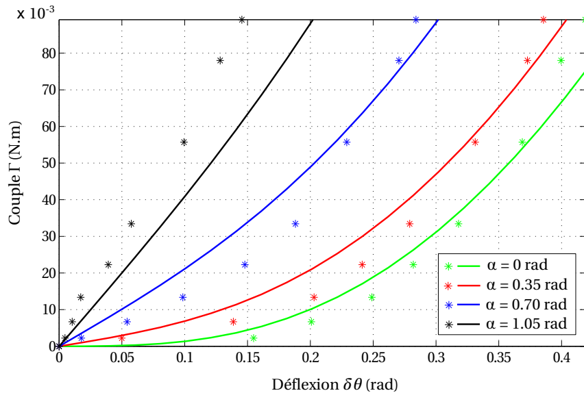
FIGURE 2.27 – Caractéristique couple/déflexion pour une rotation autour de l'axe de la liaison.
