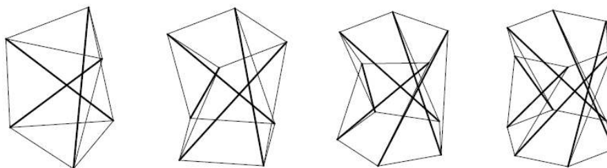
FIGURE 1.9 – Tenségrités antiprismatiques T3 à T6 [Arsenault 2006a].
