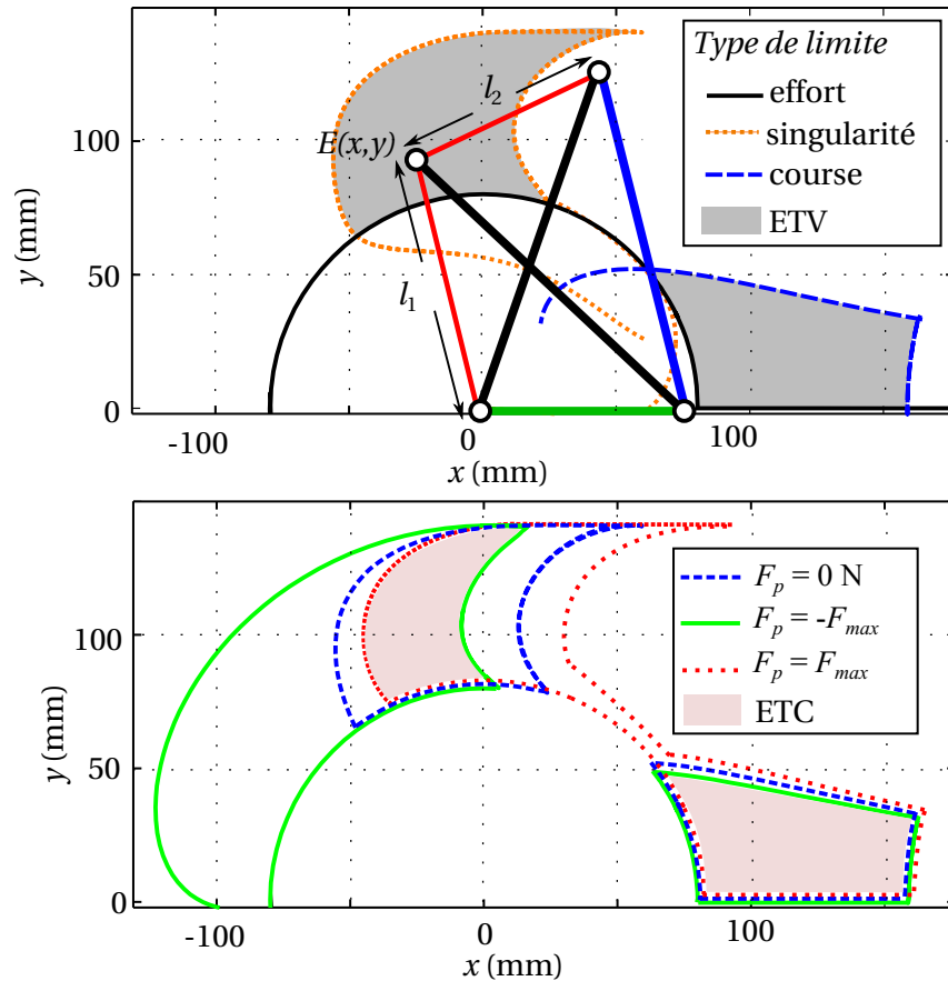
FIGURE 2.8 – Espace de travail du mécanisme de tenségrité à 2 DDL. En haut, limites de l'ETV, en bas représentation de l'ETC. Le mécanisme est représenté à gauche pour \rho = [75, 136]^T mm et F_p = 0 N.
