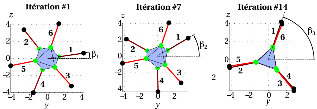
FIGURE 3.8 – Représentation du système dans le plan (O, \mathbf{e}_2, \mathbf{e}_3) pour 3 itérations différentes.
