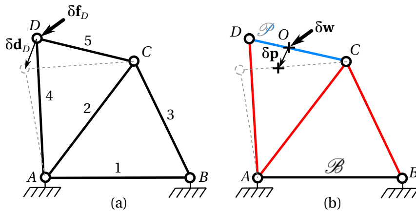
FIGURE 2.10 – Exemple d'un assemblage modélisé au sens de la mécanique des structures (a) ; au sens de la robotique (b) en considérant deux corps rigides \mathcal{B} et \mathcal{P} reliés par trois éléments élastiques (rouge).
