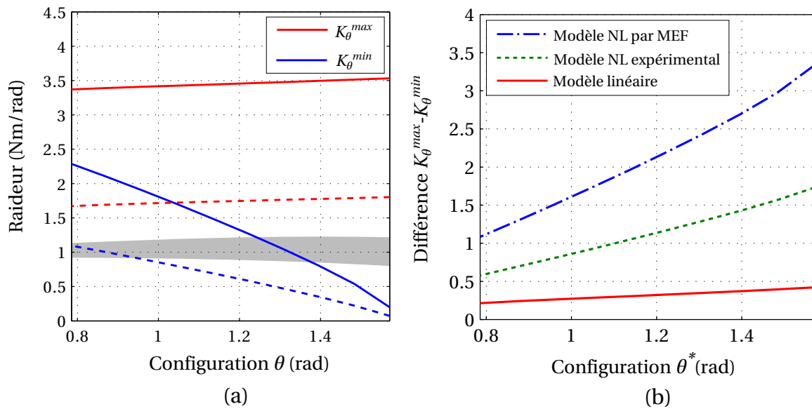
FIGURE 4.33 – Modulation de raideur avec un ressort dégressif. (a) Raideurs minimum et maximum ; (b) Différence K_\theta^{max} - K_\theta^{min} .
