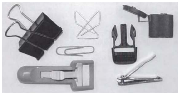
FIGURE 4.17 – Exemples de mécanismes compliant [Howell 2001].
