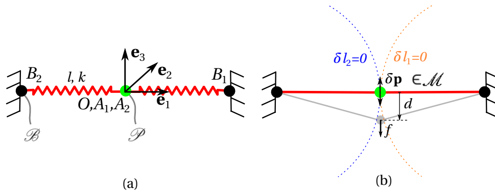
FIGURE 2.15 – Exemple de système élastique singulier à deux éléments colinéaires (a) et un de ses modes de déformation inextensible (b).
