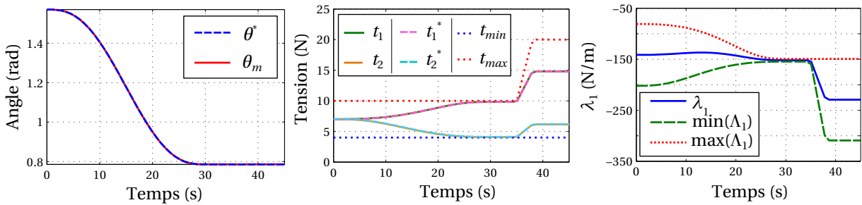
FIGURE 5.6 – Simulation d'une reconfiguration le long d'une trajectoire du troisième ordre avec la stratégie de commande en effort.
