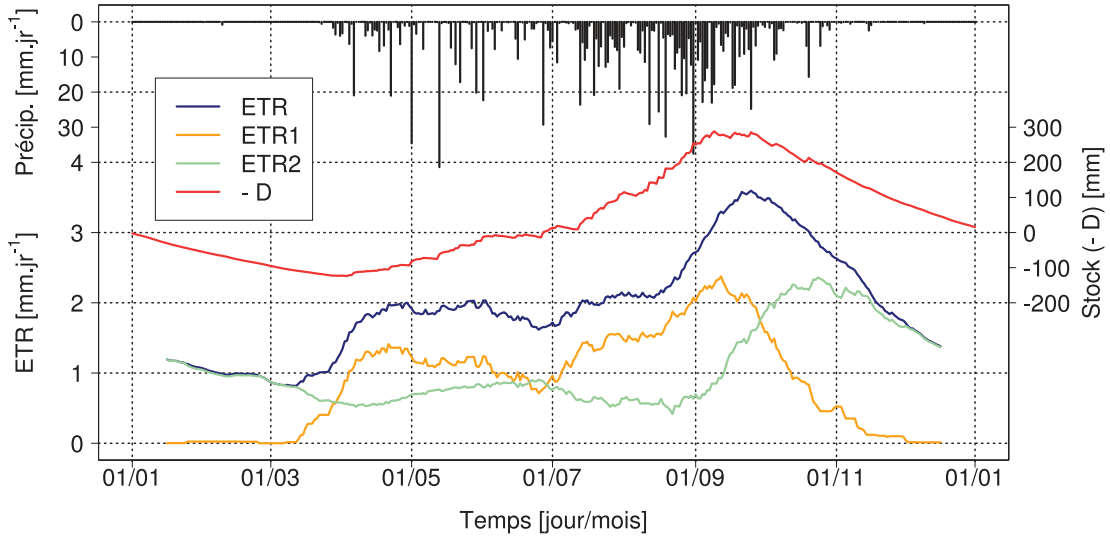
FIGURE 9.2 – Chroniques d'évapotranspiration ETR , ETR_1 et ETR_2 (mésos-échelle) de la simulation de référence pour l'année 2007. Les évapotranspirations sont moyennées sur 31 jours pour une meilleure visibilité. Chronique de variation temporelle de -\bar{D} pour la même année.
