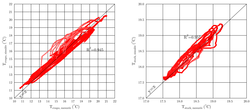
FIGURE A.12 – Coefficients de détermination de la comparaison entre simulation et mesures sur la température du stockage et de l'évaporateur durant la séquence 2 de mesure
