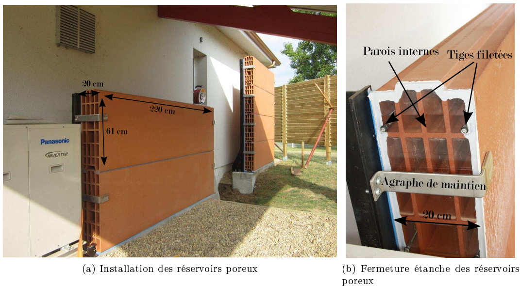
FIGURE 3.2 – Vues des réservoirs poreux (briques BHE) positionnés côté nord de la maison
