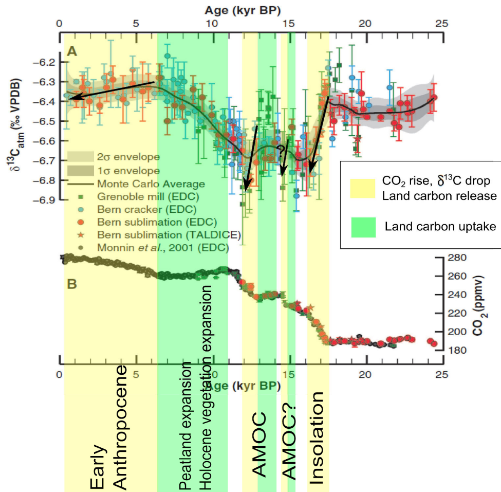
Figure 10, les données de \text{CO}_2 et \delta^{13}\text{C} rapportées par Schmitt et al (2012) avec les mécanismes proposés superposées. Les flèches indiquent la tendance générale qui peut être vu dans les données
