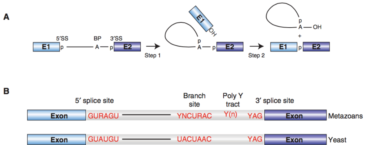
Figure 1.05 : L'élimination des introns se fait par deux étapes de trans-estérification. (A.) Représentation des deux étapes de trans-estérification. Le groupe OH de l'Adénosine de la boîte de branchement (BP) attaque le phosphate de l'exon 1 en amont (E1 5'SS). Dans un second temps, le 3'OH libéré en 3' de l'exon 1 est lié au phosphate 5' de l'exon 2 en aval (E2 3'SS). Les produits obtenus sont les deux exons ligaturés et l'intron intermédiaire ou « lariat ». (B.) Les trois éléments cis impliqués dans l'épissage sont conservés entre les eucaryotes supérieurs et S.cerevisiae . La séquence de la boîte de branchement est moins conservés chez les eucaryotes supérieurs. Y : résidus pyrimidines ; R : résidus purines. D'après Will et Luhrmann, 2011.
