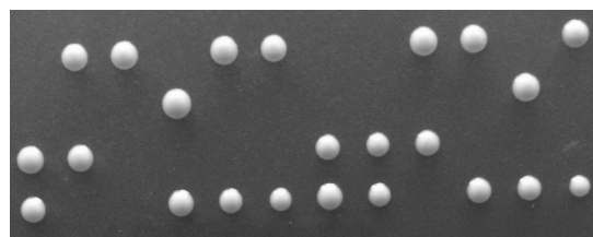
Figure 2.18 : La mutation des deux motifs en doigt de zinc de Pcf11 est létale chez S. cerevisiae . (haut) Représentation schématique de la mutation de l'allèle pcf11-20 mutations au niveau de deux motifs en doigt de zinc (C421S, C424S, C564S, C567S). (bas) Étude de la ségrégation des spores pour la mutation de deux motifs en doigt de zinc de Pcf11. Les spores sont séparées à l'aide d'un micromanipulateur sur milieu YPD(A) puis incubées à 24°C 3 jours. La présence de cellules est vérifiée au microscope.
