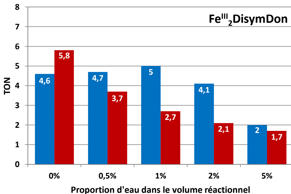
Figure IV.14 : Valeurs de TON pour la réaction d'oxydation du cyclohexane par le peroxyde d'hydrogène en présence de complexe Fe III 2 DisymDon (en bleu : cyclohexanol, en rouge : cyclohexanone), dans un mélange acétonitrile/eau à température ambiante (estimée à 30°C). Conditions : complexe/H 2 O 2 /cyclohexane (1/100/1000).
