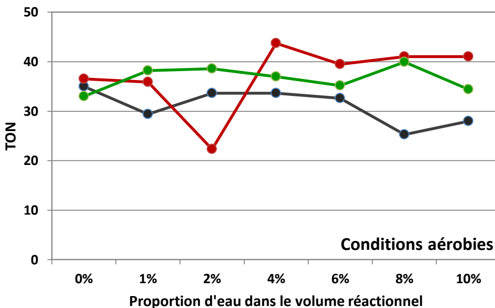
Figure IV.16 : Valeurs de TON pour la réaction d'oxydation du cyclohexène par le peroxyde d'hydrogène en présence de catalyseur (en noir : \text{Fe}^{\text{III}}_2\text{Ref} , en rouge : \text{Fe}^{\text{III}}_2\text{DisymDon} et en vert : \text{Fe}^{\text{III}}_2\text{SymDon} ), dans un mélange acétonitrile/eau à température ambiante (estimée à 30°C), en conditions aérobies. Conditions : complexe/ \text{H}_2\text{O}_2 /cyclohexène (1/10/1000).
