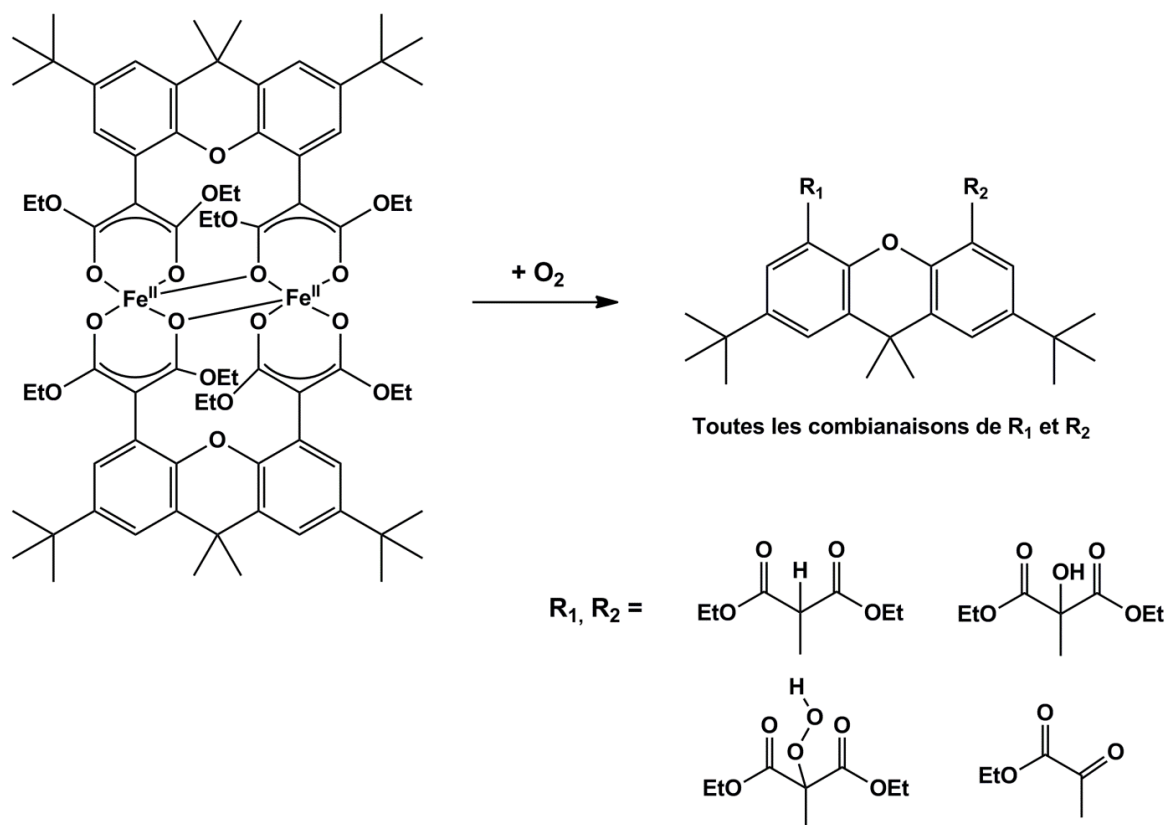
Figure I.36 : Oxydation intramoléculaire en position \alpha des fonctions esters du ligand.
