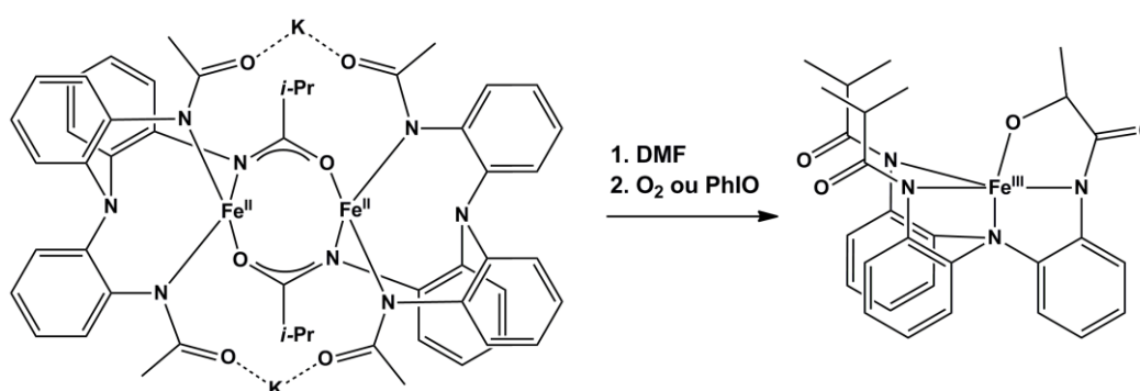
Figure I.35 : Oxydation intramoléculaire d'une liaison C-H aliphatique par le dioxygène, catalysée par un complexe \text{Fe}^{\text{II}}\text{Fe}^{\text{II}} .
