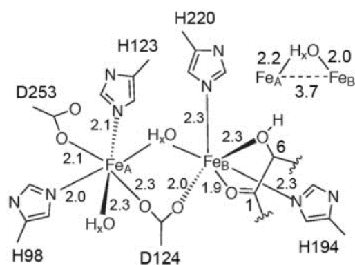
Figure I.17 : Structure du site actif de la MIOX. Les distances sont données en Angstroms. Seuls les atomes de carbone C1 et C6 de la molécule de myo-inositol sont représentés pour plus de clarté. 168
