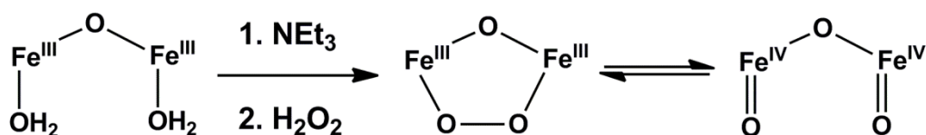
Figure I.33 : Équilibre dynamique entre les intermédiaires \mu -oxo- \mu -peroxy- \text{Fe}^{\text{III}}\text{Fe}^{\text{III}} et \mu -oxo-bis-oxo- \text{Fe}^{\text{IV}}\text{Fe}^{\text{IV}} .
