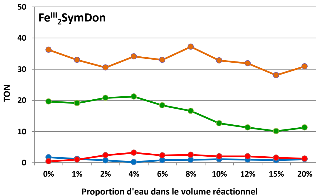
Figure IV.21 : Valeurs de TON pour la réaction d'oxydation du cyclohexène par le peroxyde d'hydrogène en présence de complexe Fe III 2 SymDon (en bleu : époxyde, en rouge : cis-1,2-diol, en vert : énone, en orange : énone), dans un mélange acétonitrile/eau à température ambiante (estimée à 30°C), en conditions anaérobies. Conditions : complexe/H 2 O 2 /cyclohexène (1/100/1000).
