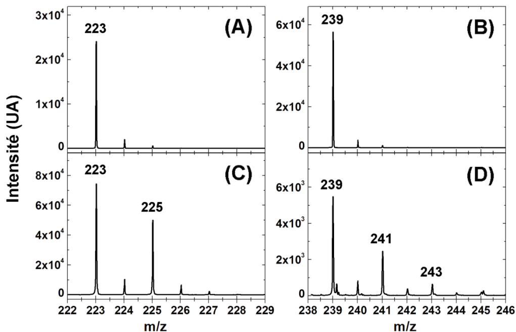
Figure IV.7 : Massifs isotopiques du DBTO ( m/z 223) et du DBTO 2 ( m/z 239) après la réaction d'oxydation du DBT par H 2 O 2 et Fe III 2 Ref en absence (A et B) et en présence (C et D) de 1000 équivalents d'eau marquée H 2 18 O dans le milieu réactionnel.
