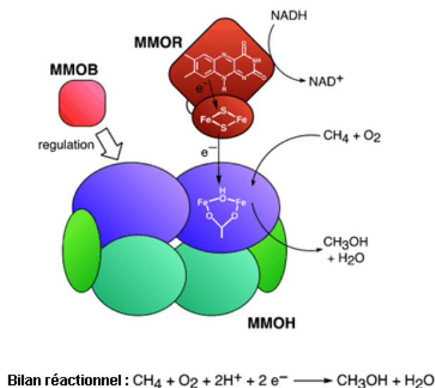
Schéma I.9 : Représentation schématique du mécanisme d'action concerté des trois sous-unités de la sMMO. 51
