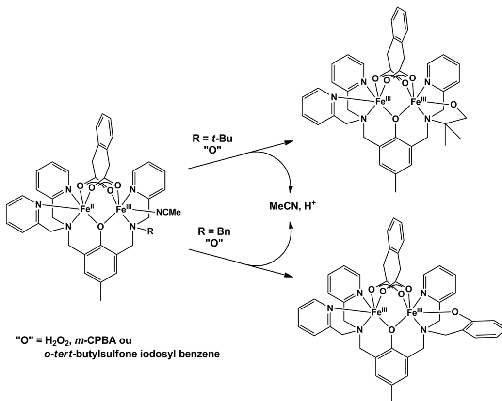
Figure I.38 : Oxydation intramoléculaire de liaisons C-H aliphatiques et aromatiques par des réactifs de transfert d'oxygène.
