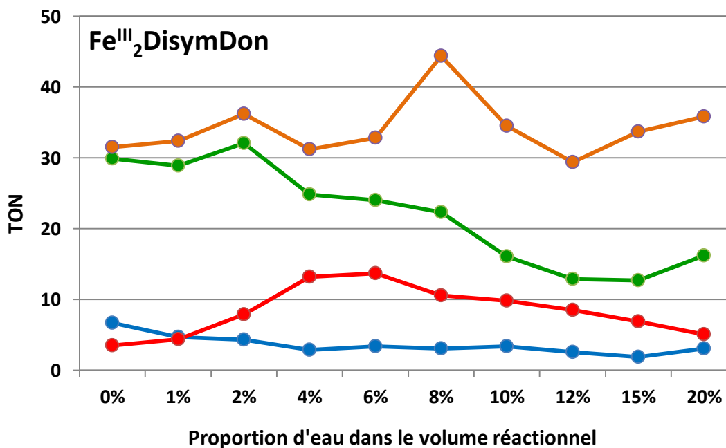
Figure IV.20 : Valeurs de TON pour la réaction d'oxydation du cyclohexène par le peroxyde d'hydrogène en présence de complexe Fe III 2 DisymDon (en bleu : époxyde, en rouge : cis-1,2-diol, en vert : énonol, en orange : énone), dans un mélange acétonitrile/eau à température ambiante (estimée à 30°C), en conditions anaérobies. Conditions : complexe/H 2 O 2 /cyclohexène (1/100/1000).
