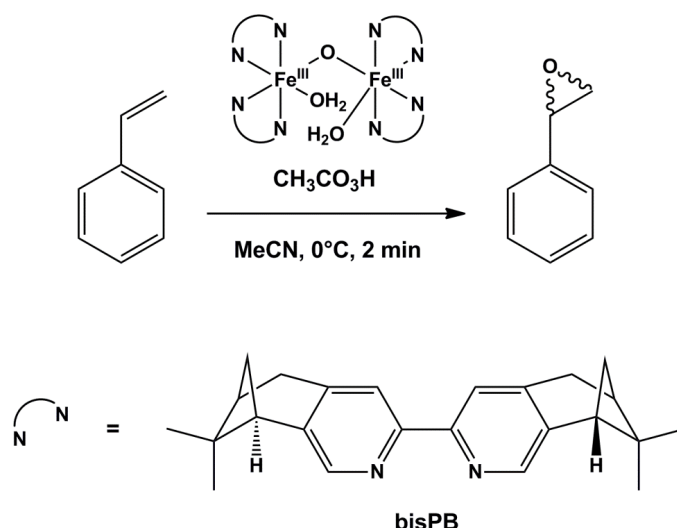
Figure I.44 : Epoxydation du styrène par l'acide peroxyacétique catalysée par le complexe chiral [\text{Fe}_2(\mu\text{-O})(\text{bisPB})_4(\text{H}_2\text{O})_2](\text{ClO}_4)_4 .
