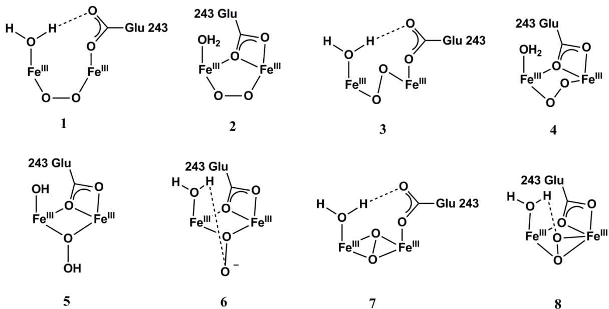
Figure I.3 : Structures possibles de l'intermédiaire MMOH P . 68
