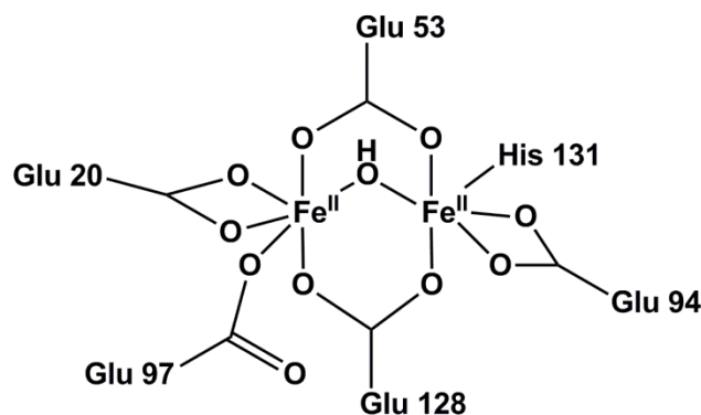
Figure I.21 : Site actif de la Rubrérythrine sous forme réduite (Rr red ). 180
