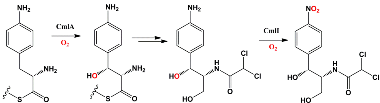
Schéma I.13 : Biosynthèse du chloramphénicol chez Streptomyces venezuelae .
