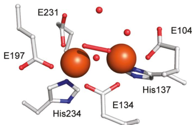
Figure I.8 : Structure tridimensionnelle de l'intermédiaire peroxy-T4MO obtenue par diffraction des rayons X. Les molécules d'eau sont représentées par des sphères rouges et le ligand peroxy est représenté par un bâton rouge. 113
