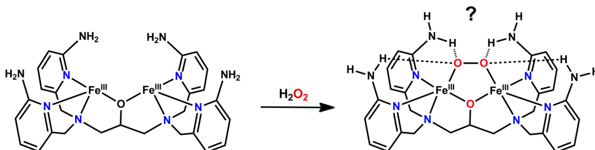
Schéma III.1 : Formation potentielle de liaisons hydrogène au sein d'un intermédiaire \mu -peroxo- \text{Fe}^{\text{III}}\text{Fe}^{\text{III}} obtenu à partir du complexe \text{Fe}^{\text{III}}_2\text{AmineSym} .
