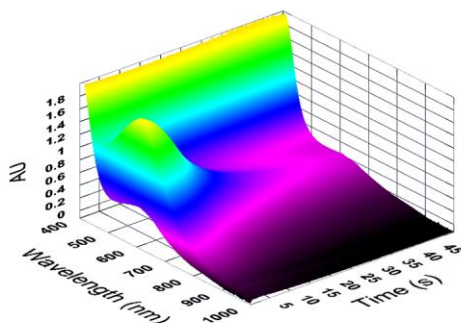
Figure III.5 : Spectre d'absorption électronique UV/visible obtenu par la méthode de flux stoppé, lors du suivi de la réaction entre le peroxyde d'hydrogène et le complexe \text{Fe}^{\text{III}}_2\text{SymDon} , dans l'acétonitrile à température ambiante.
