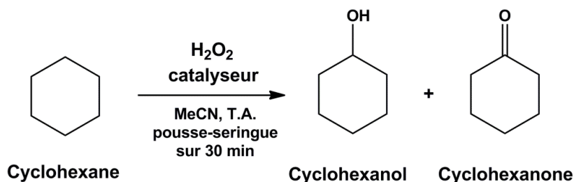
Schéma IV.9 : Oxydation du cyclohexane par le peroxyde d'hydrogène en présence de catalyseur, dans l'acétonitrile à température ambiante.
