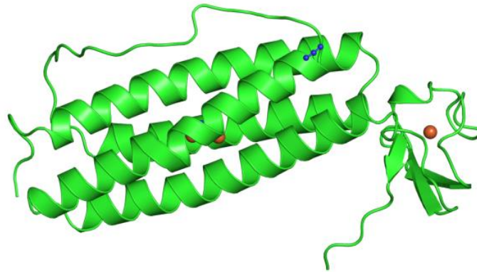
Figure I.20 : Structure d'une unité monomérique de la rubrérythrine en présence d'un ion azoture (Rr red -N 3 ). 181
