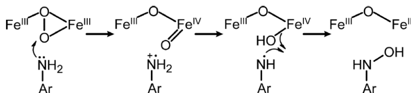
Figure I.14 : Mécanisme proposé pour la première étape d'oxydation d'arylamines par CmlII. 156
