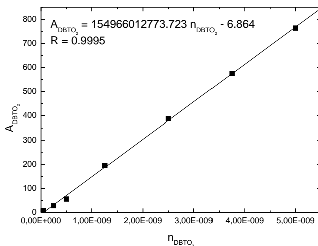
Figure PE.4 : Droite d'étalonnage A_{DBTO_2} - n_{DBTO_2}
