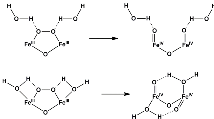
Schéma IV.13 : Mécanisme proposé pour la stabilisation des intermédiaires \mu -peroxo- \text{Fe}^{\text{III}}\text{Fe}^{\text{III}} et bis-oxo- \text{Fe}^{\text{IV}}\text{Fe}^{\text{IV}} par liaisons hydrogène intra ou intermoléculaires, en présence d'eau dans le milieu réactionnel.
