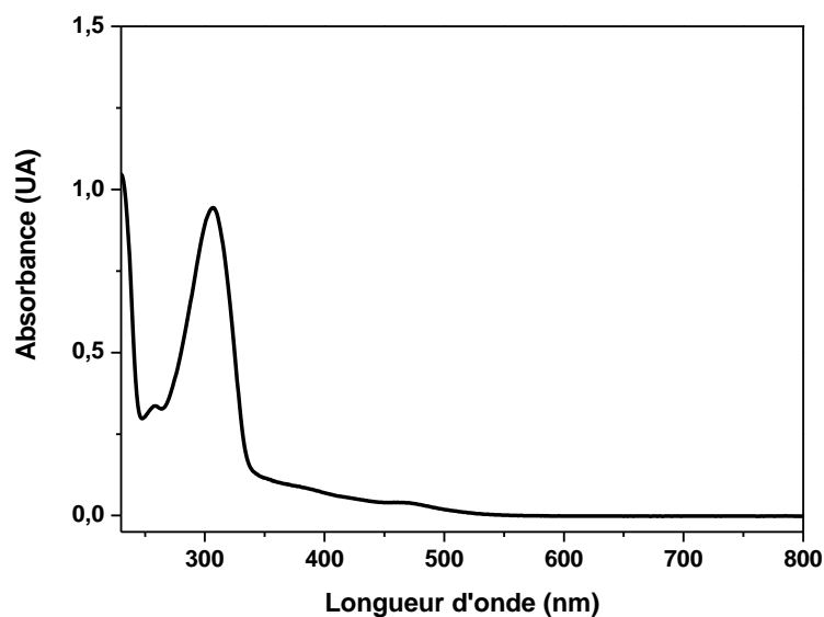
Figure II.10 : Spectre d'absorption UV/visible du complexe \text{Fe}^{\text{III}}_2\text{AmineSym} formé in situ , enregistré dans l'acétonitrile à 25°C et à une concentration de 25 \mu\text{M} .
