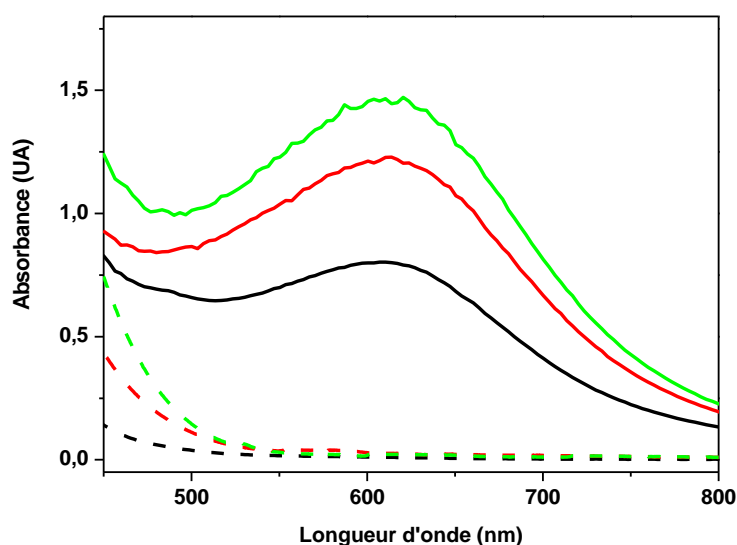
Figure III.2 : Spectres d'absorption UV/visible des intermédiaires formés par addition de 50 équivalents de peroxyde d'hydrogène sur les complexes \text{Fe}^{\text{III}}_2\text{Ref} (en noir), \text{Fe}^{\text{III}}_2\text{DisymDon} (en rouge) et \text{Fe}^{\text{III}}_2\text{SymDon} (en vert), enregistrés dans l'acétonitrile à 20°C et à une concentration de 1 mM.
