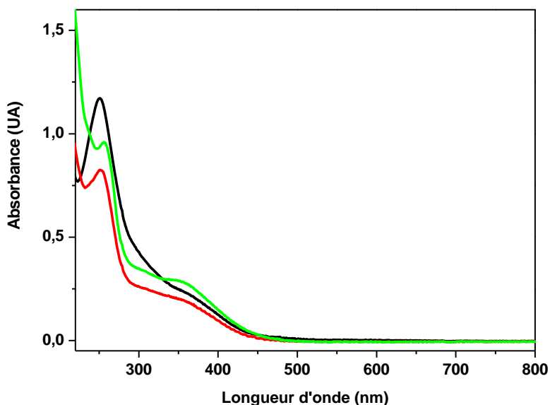
Figure II.5 : Spectres d'absorption UV/visible des complexes \text{Fe}^{\text{III}}_2\text{Ref} (en noir), \text{Fe}^{\text{III}}_2\text{DisymDon} (en rouge) et \text{Fe}^{\text{III}}_2\text{SymDon} (en vert), enregistrés dans l'acétonitrile à 25°C et à une concentration de 25 \mu\text{M} .
