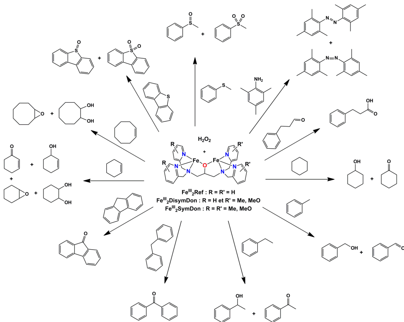
Schéma IV.20 : Schéma global des différentes réactions d'oxydation étudiées dans ce chapitre.
