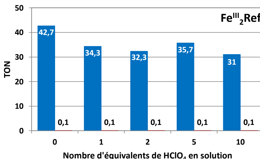
Figure IV.28 : Valeurs de TON pour la réaction d'oxydation du cyclooctène par le peroxyde d'hydrogène en présence de complexe Fe III 2 Ref (en bleu : époxyde, en rouge : cis -1,2-diol), dans l'acétonitrile à température ambiante (estimée à 30°C), en conditions aérobies. Conditions : complexe/H 2 O 2 /cyclooctène/acide perchlorique (1/100/1000/x) avec x = [0 – 10].
