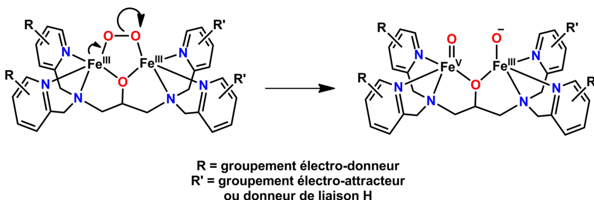
Schéma II.9 : Rupture hétérolytique de la liaison O-O d'un intermédiaire \mu -peroxo- \text{Fe}^{\text{III}}\text{Fe}^{\text{III}} dans un complexe possédant une seconde sphère de coordination fortement dissymétrique.
