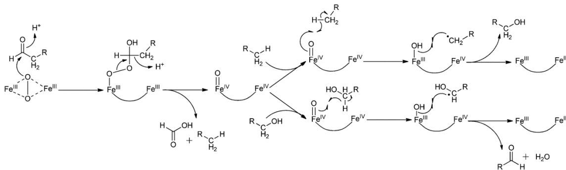
Figure I.12 : Mécanisme alternatif proposé pour la réaction de déformylation des aldéhydes par la cADO. 147
