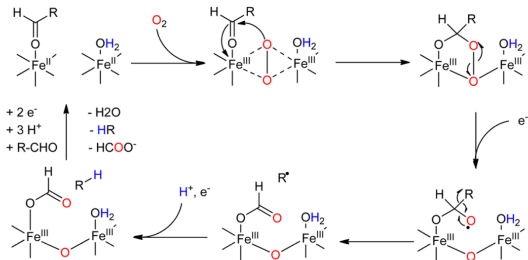
Figure I.11 : Mécanisme proposé pour la déformylation d'aldéhydes par la cADO. 147
