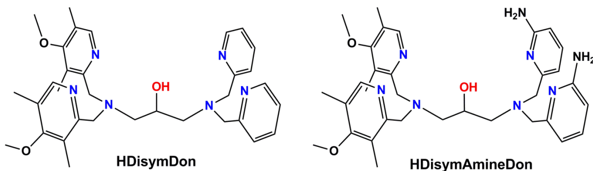
Schéma II.14 : Ligand HDisymDon (à gauche) et exemple du ligand HDisymAmineDon , à forte dissymétrie (à droite).
