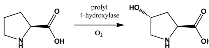
Schéma I.6 : Conversion de la L-proline en (2S, 4R)-4-hydroxyproline catalysée par la prolyl 4-hydroxylase.
