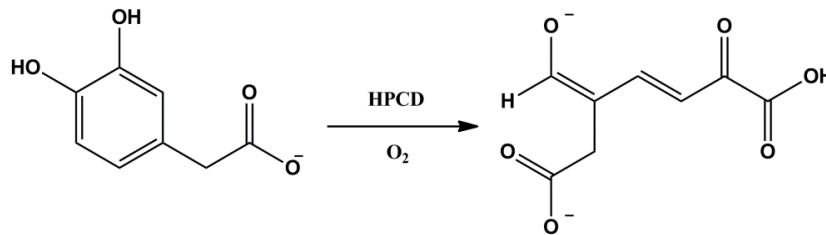
Schéma I.5 : Oxydation du 3,4-dihydroxyphénylacétate par le dioxygène catalysée par HPCD.
