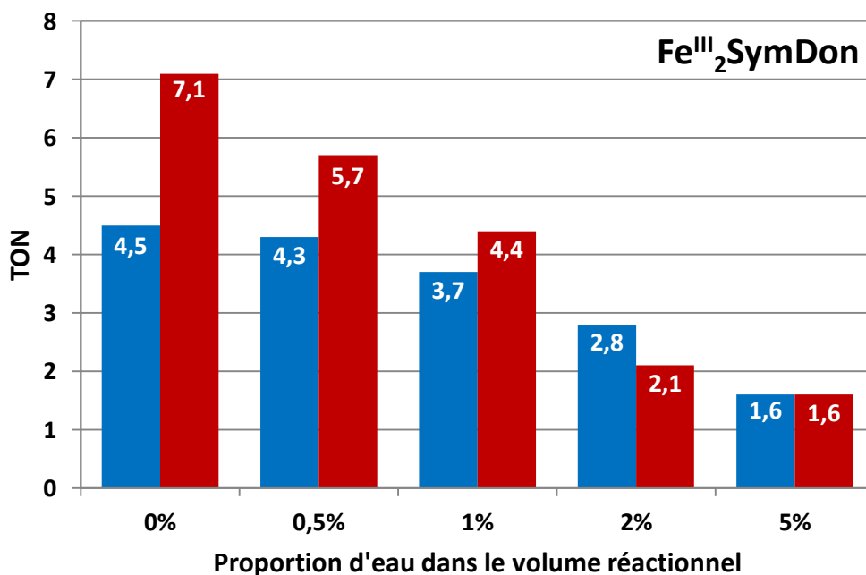
Figure IV.15 : Valeurs de TON pour la réaction d'oxydation du cyclohexane par le peroxyde d'hydrogène en présence de complexe Fe III 2 SymDon (en bleu : cyclohexanol, en rouge : cyclohexanone), dans un mélange acétonitrile/eau à température ambiante (estimée à 30°C). Conditions : complexe/H 2 O 2 /cyclohexane (1/100/1000).
