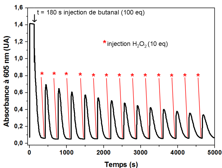
Figure IV.33 : Suivi de l'absorbance à 605 nm lors de l'ajout de 10 équivalents de peroxyde d'hydrogène (à t = 0 s) à une solution de complexe Fe III 2 SymDon à 0,5 mM, dans un mélange acétonitrile/méthanol en proportions égales, à 5°C. A t = 180 s, injection de 100 équivalents de butanal, puis réinjection de 10 équivalents de peroxyde d'hydrogène à t = 480, 840, 1200, 1560, 1920, 2280, 2640, 3000, 3360, 3720, 4080, 4440 et 4800 s.
