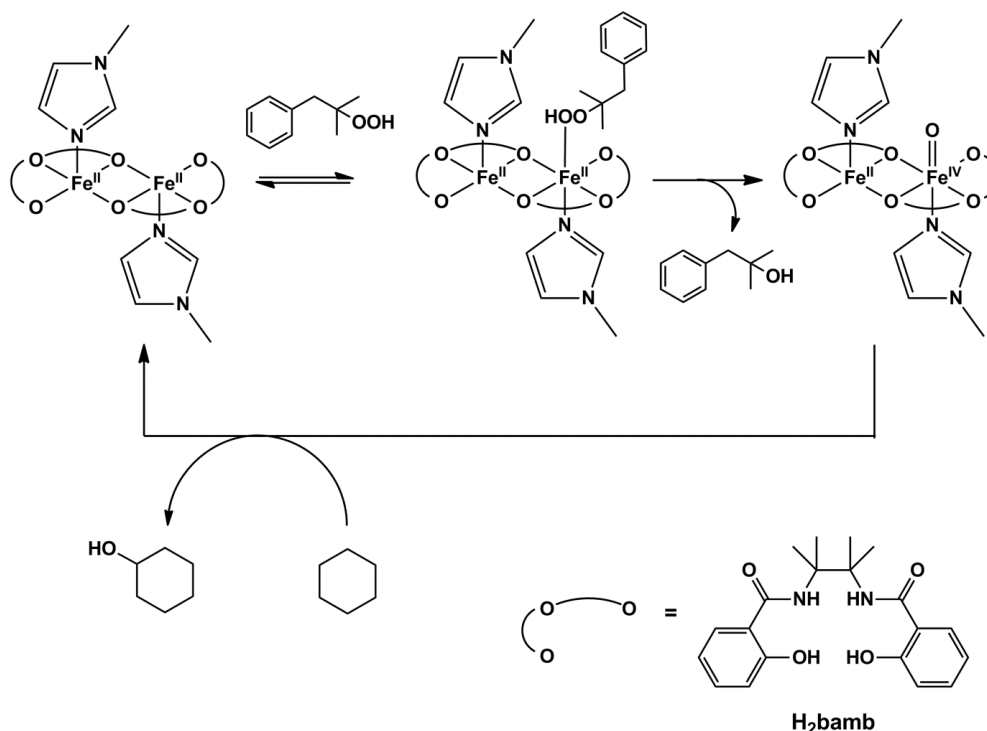
Figure I.40 : Mécanisme proposé pour l'hydroxylation du cyclohexane par MPPH, catalysée par le complexe [(\text{H}_2\text{bamb})_2\text{Fe}_2(\text{N-Melm})_2] .
