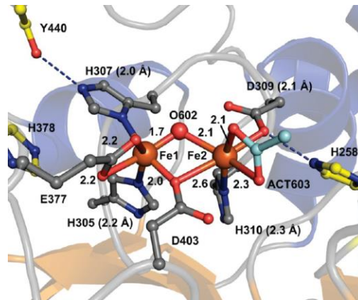
Figure I.13 : Structure du site actif binucléaire à fer de la CmlA \beta -hydroxylase, obtenue par diffraction des rayons X. Les longueurs de liaisons sont indiquées en Angstroms et les liaisons hydrogènes sont représentées en pointillés. 154
