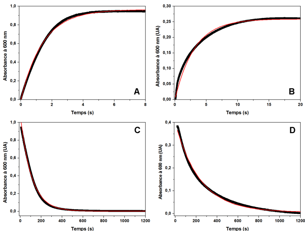
Figure III.9 : Cinétique de formation et de dégradation des intermédiaires \mu -peroxo- \text{Fe}^{\text{III}}\text{Fe}^{\text{III}} , absorbance à 600 nm en fonction du temps. Les courbes A et B correspondent à la formation des intermédiaires \mu -peroxo- \text{Fe}^{\text{III}}\text{Fe}^{\text{III}} formés respectivement à partir des complexes \text{Fe}^{\text{III}}_2\text{Ref} et \text{Fe}^{\text{III}}_2\text{AmineSym} , tandis que les courbes C et D correspondent à la dégradation des intermédiaires \mu -peroxo- \text{Fe}^{\text{III}}\text{Fe}^{\text{III}} formés respectivement à partir des complexes \text{Fe}^{\text{III}}_2\text{Ref} et \text{Fe}^{\text{III}}_2\text{AmineSym} . Les courbes en rouge représentent les courbes de régression non linéaire à partir desquelles ont été calculées les valeurs des constantes de vitesse.
