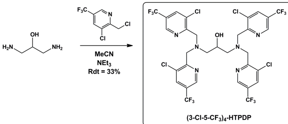
Schéma II.6 : Synthèse du ligand (3-Cl-5-CF 3 ) 4 -HTPDP.
