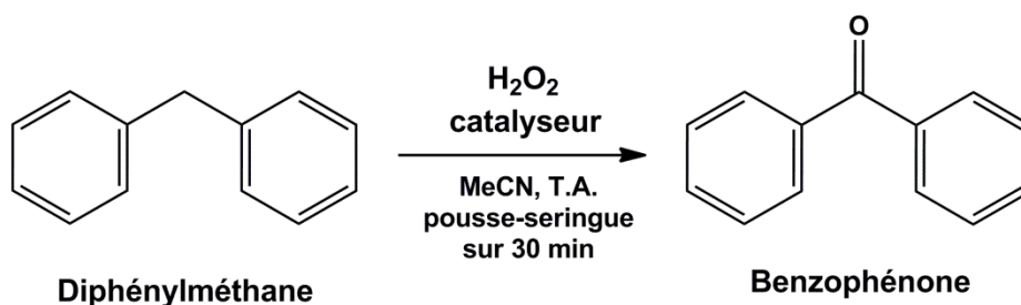
Schéma IV.5 : Oxydation du diphenylmethane par le peroxyde d'hydrogene en presence de catalyseur, dans l'acetonitrile a temperature ambiante.
