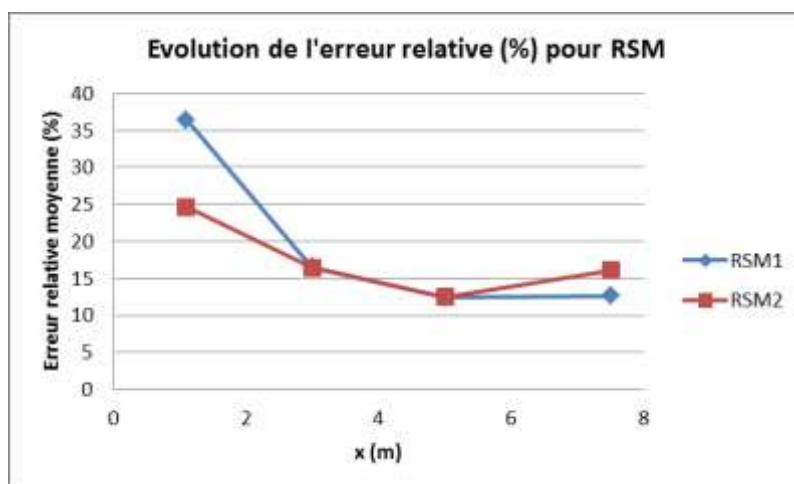
Figure 47. Évolution de l'erreur relative moyenne (%) le long du canal LNEC dans le Cas I
