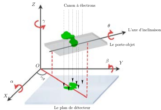
FIGURE 1.15 — Le mécanisme d'un microscope MET
