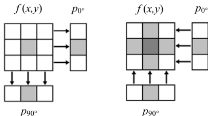
FIGURE 2.6 — Rétroprojection directe (à gauche : acquisition, à droite : reconstruction avec présence d'artefacts en étoile autour du pixel central) [Tra13]
